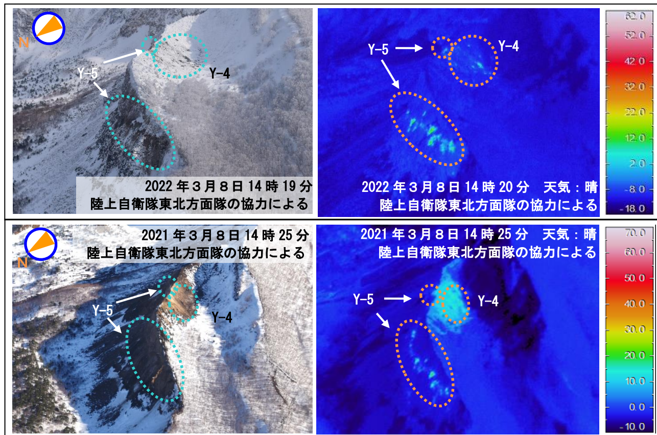
図6 磐梯山 上空から撮影した山体北側火口壁噴気地帯（Y-4、5）の状況と地表面温度分布 ※地熱域以外の温度の高い部分は日射による影響と推定されます。
