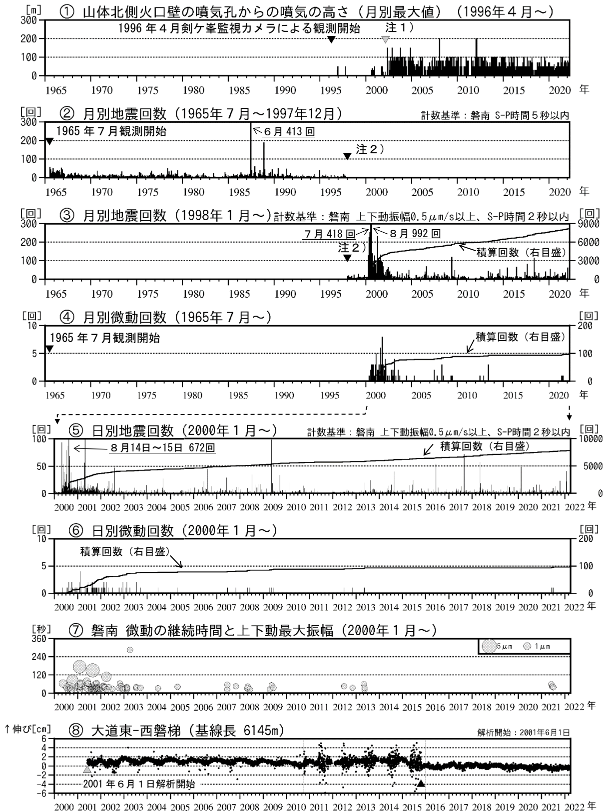
図7 磐梯山 火山活動経過図（1965年7月～2022年3月）
