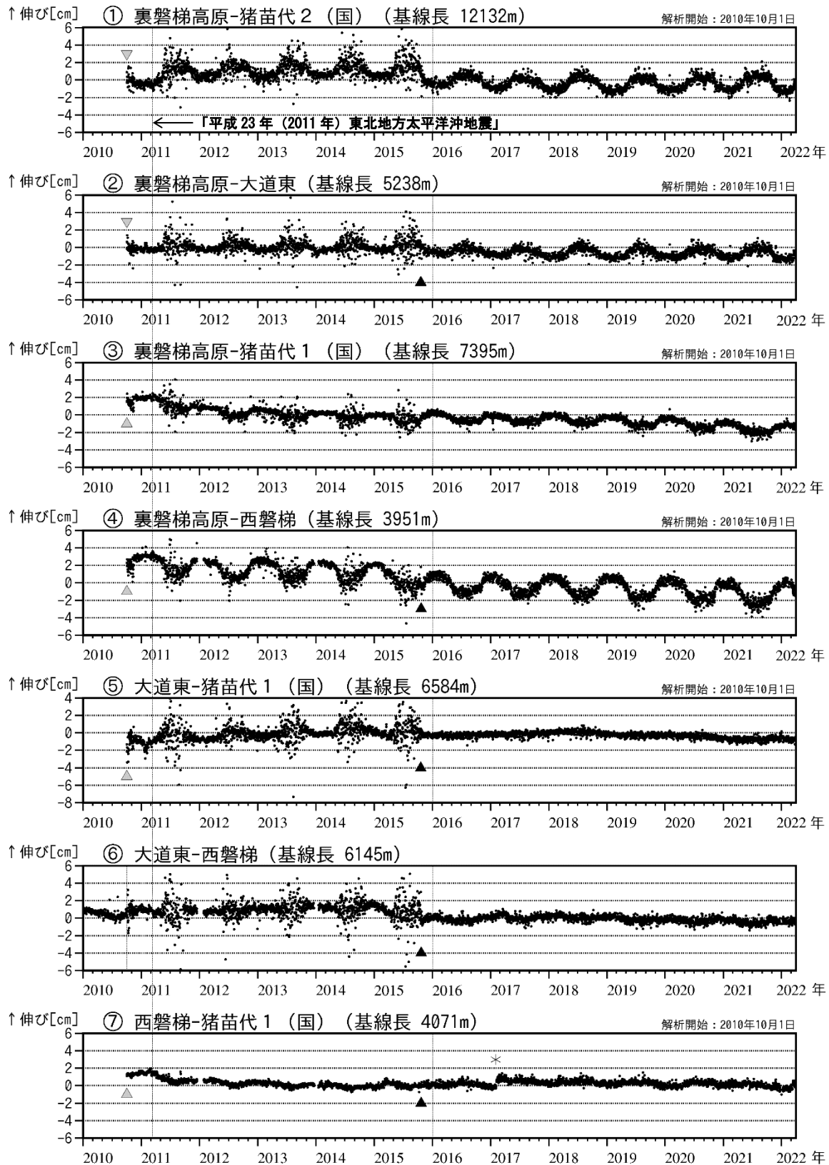
図8 磐梯山 GNSS 基線長変化図（2010年1月～2022年3月）
