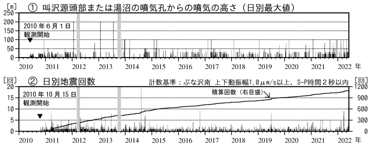
図3 秋田焼山 火山活動経過図（2010年6月～2022年5月）
