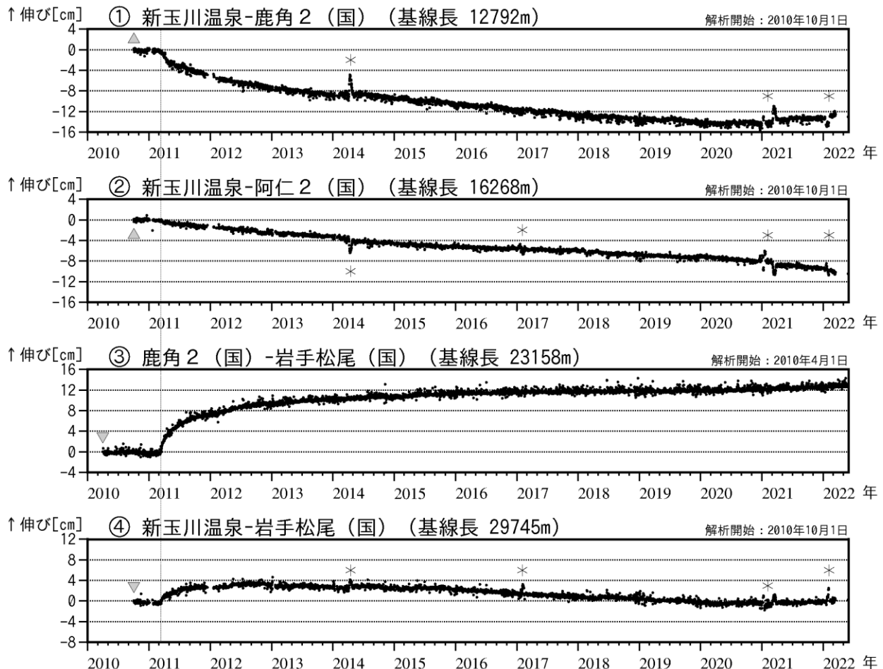
図4 秋田焼山 GNSS 基線長変化図（2010年4月～2022年5月）
