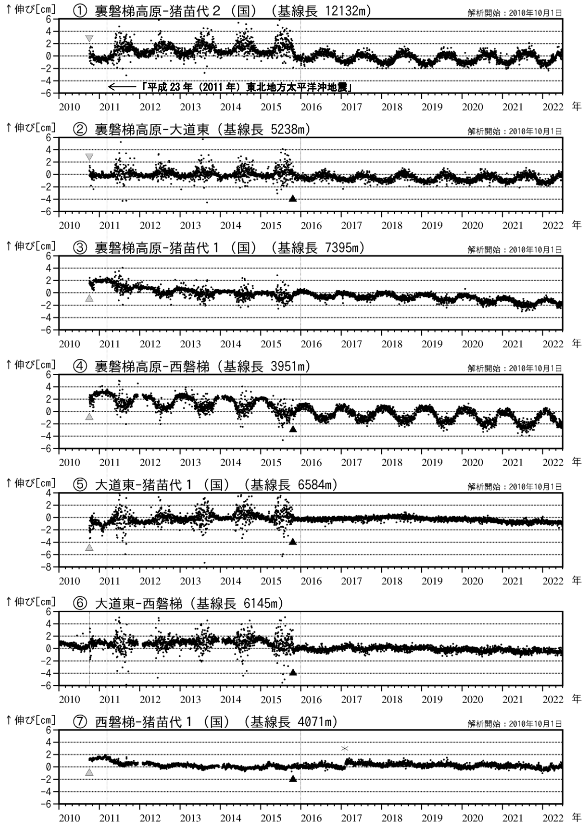
図4 磐梯山 GNSS 基線長変化図 (2010年1月～2022年6月)
