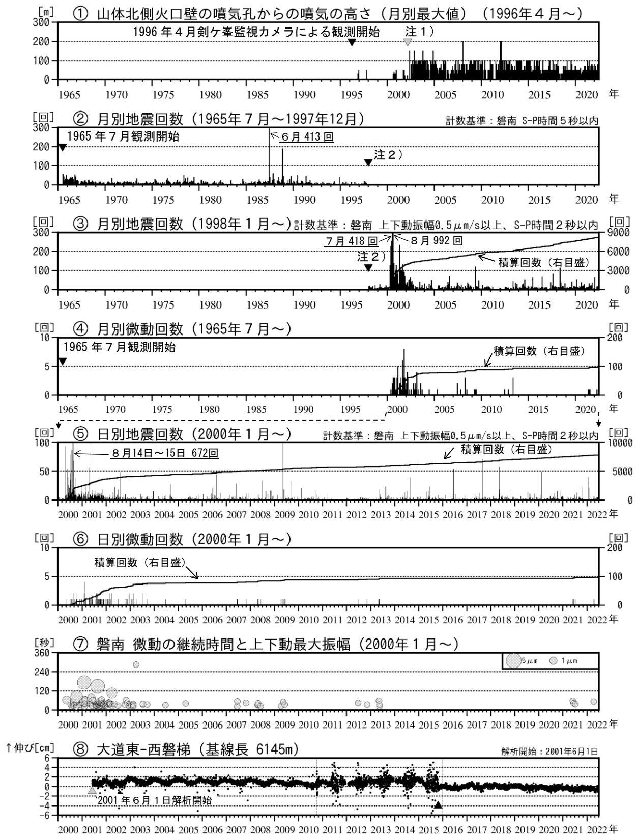
図3 磐梯山 火山活動経過図（1965年7月～2022年6月）
