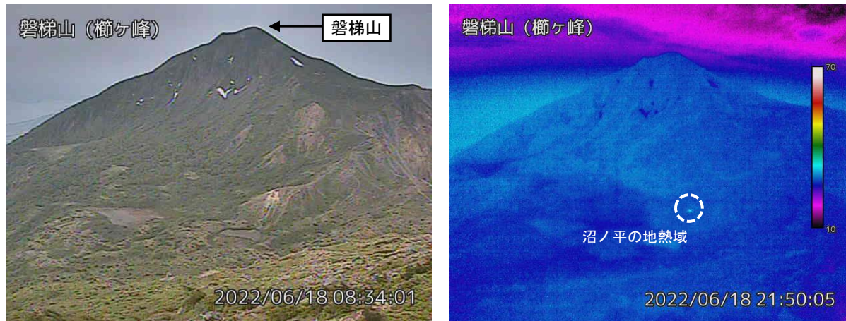
図2 磐梯山 沼ノ平周辺の状況と地表面温度分布（6月18日）
