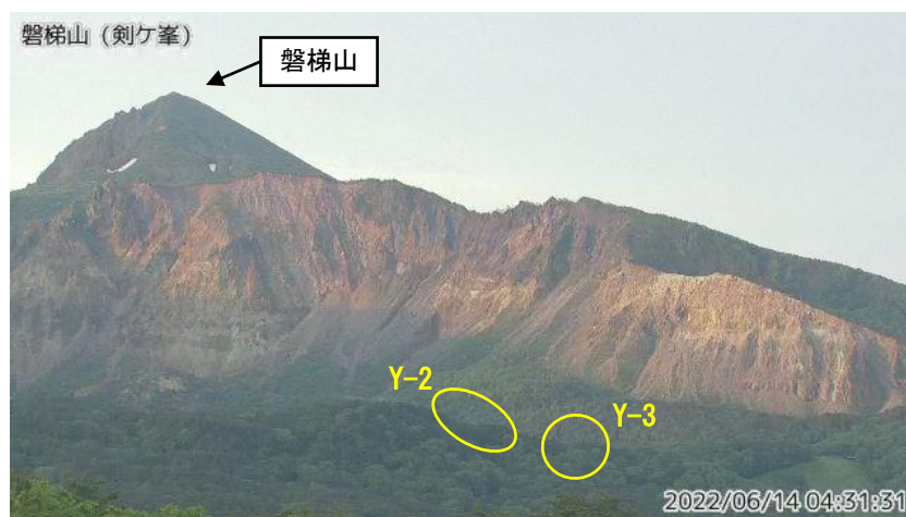
図1 磐梯山 山体北側火口壁の噴気の状況（6月14日）
