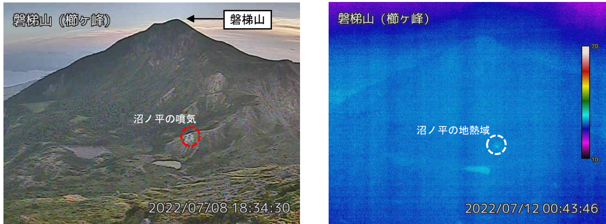
図2 磐梯山 沼ノ平周辺の状況（7月8日）と地表面温度分布（7月12日）
