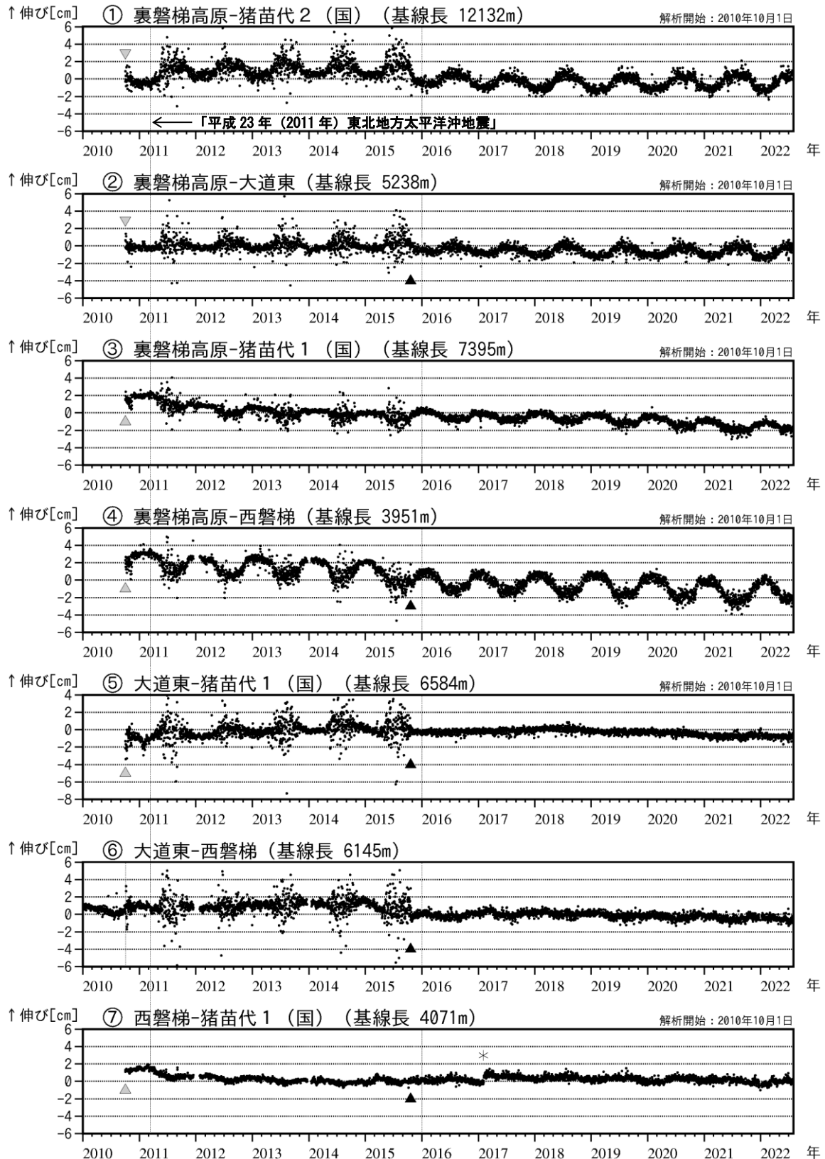
図4 磐梯山 GNSS 基線長変化図 (2010年1月～2022年7月)
