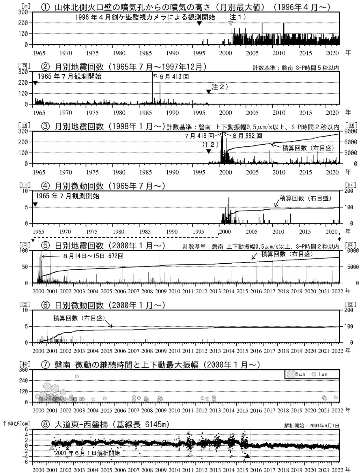
図3 磐梯山 火山活動経過図（1965年7月～2022年7月）
