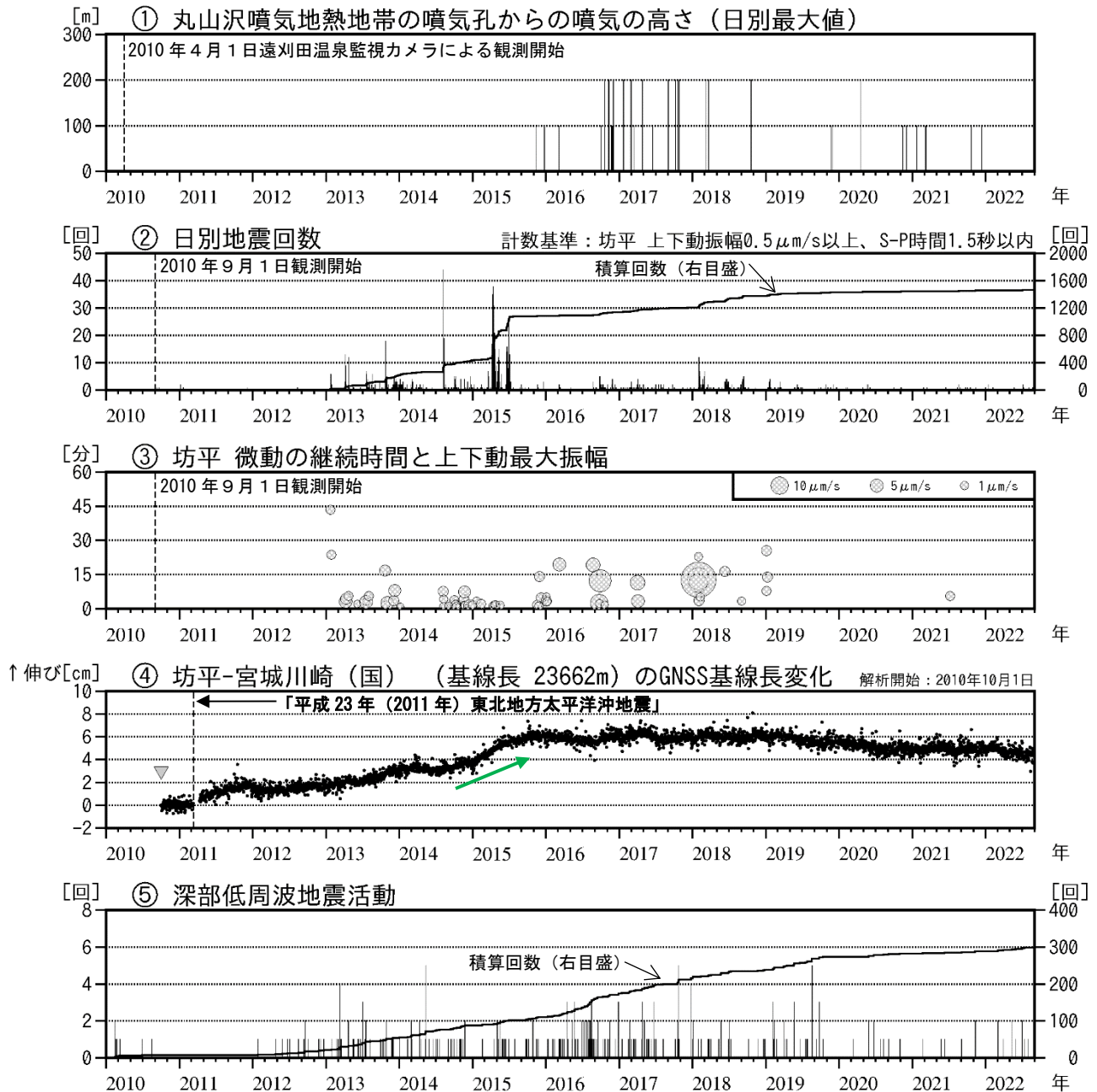
図2 蔵王山 火山活動経過図（2010年4月～2022年8月）
