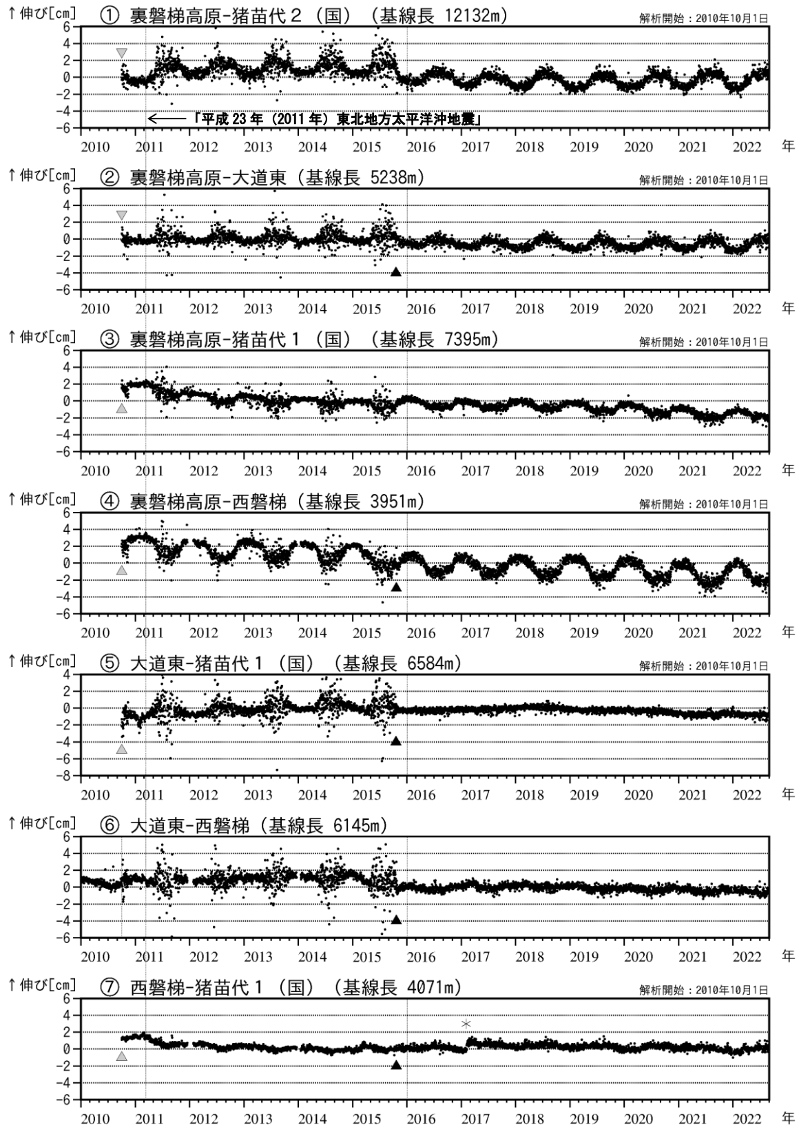
図4 磐梯山 GNSS 基線長変化図 (2010年1月～2022年8月)
