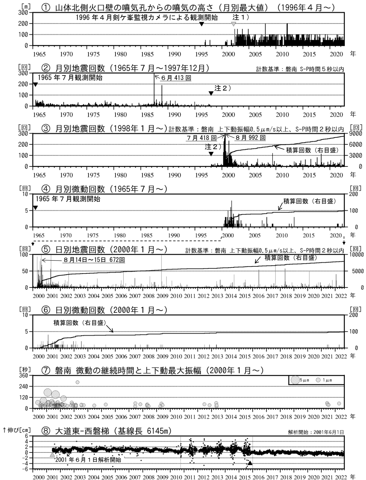
図3 磐梯山 火山活動経過図（1965年7月～2022年8月）
