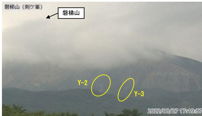
図1 磐梯山 山体北側火口壁の噴気の状況（8月27日）
