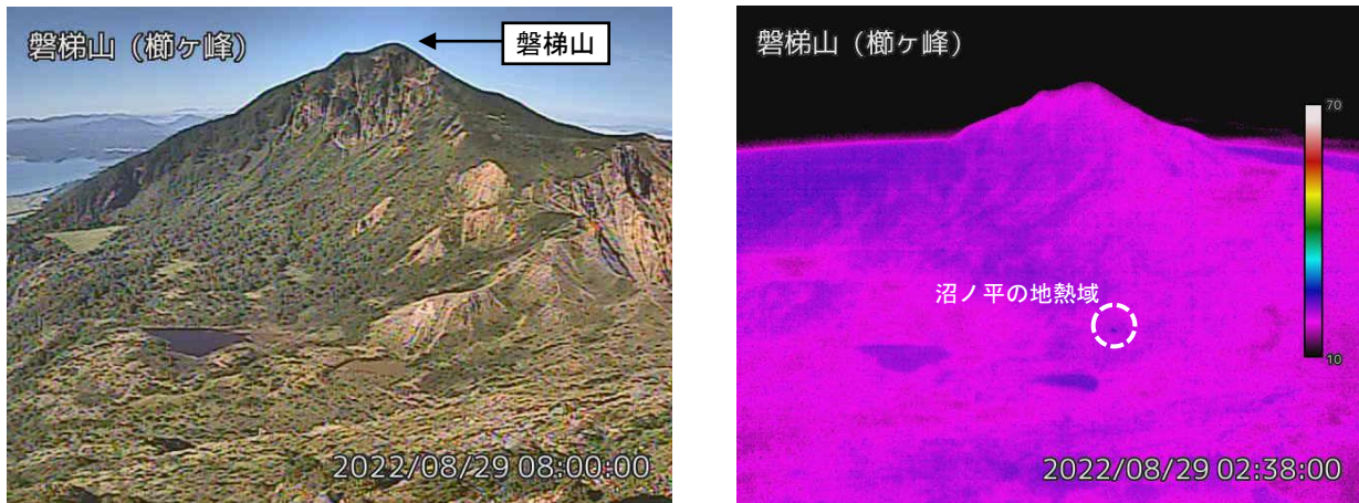
図2 磐梯山 沼ノ平周辺の状況と地表面温度分布（8月29日）
