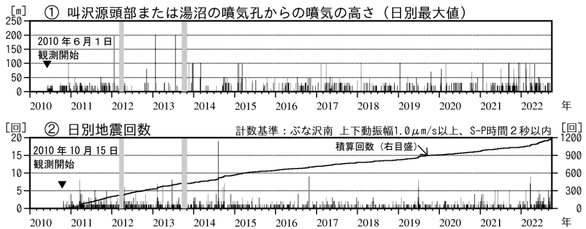
図3 秋田焼山 火山活動経過図（2010年6月～2022年9月）
