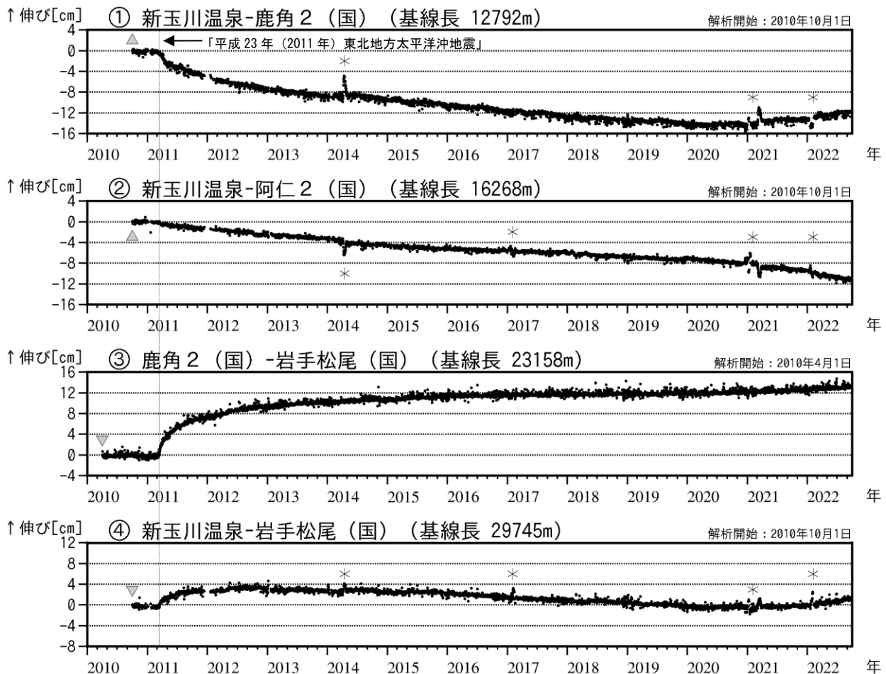
図4 秋田焼山 GNSS 基線長変化図（2010年4月～2022年9月）
