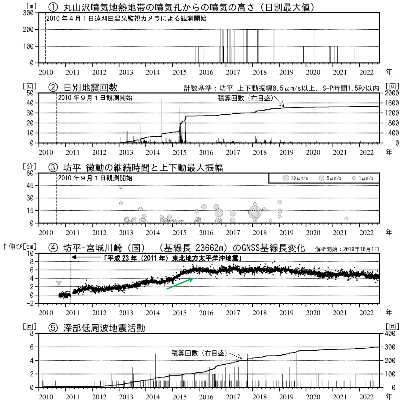
図2 蔵王山 火山活動経過図（2010年4月～2022年9月）
