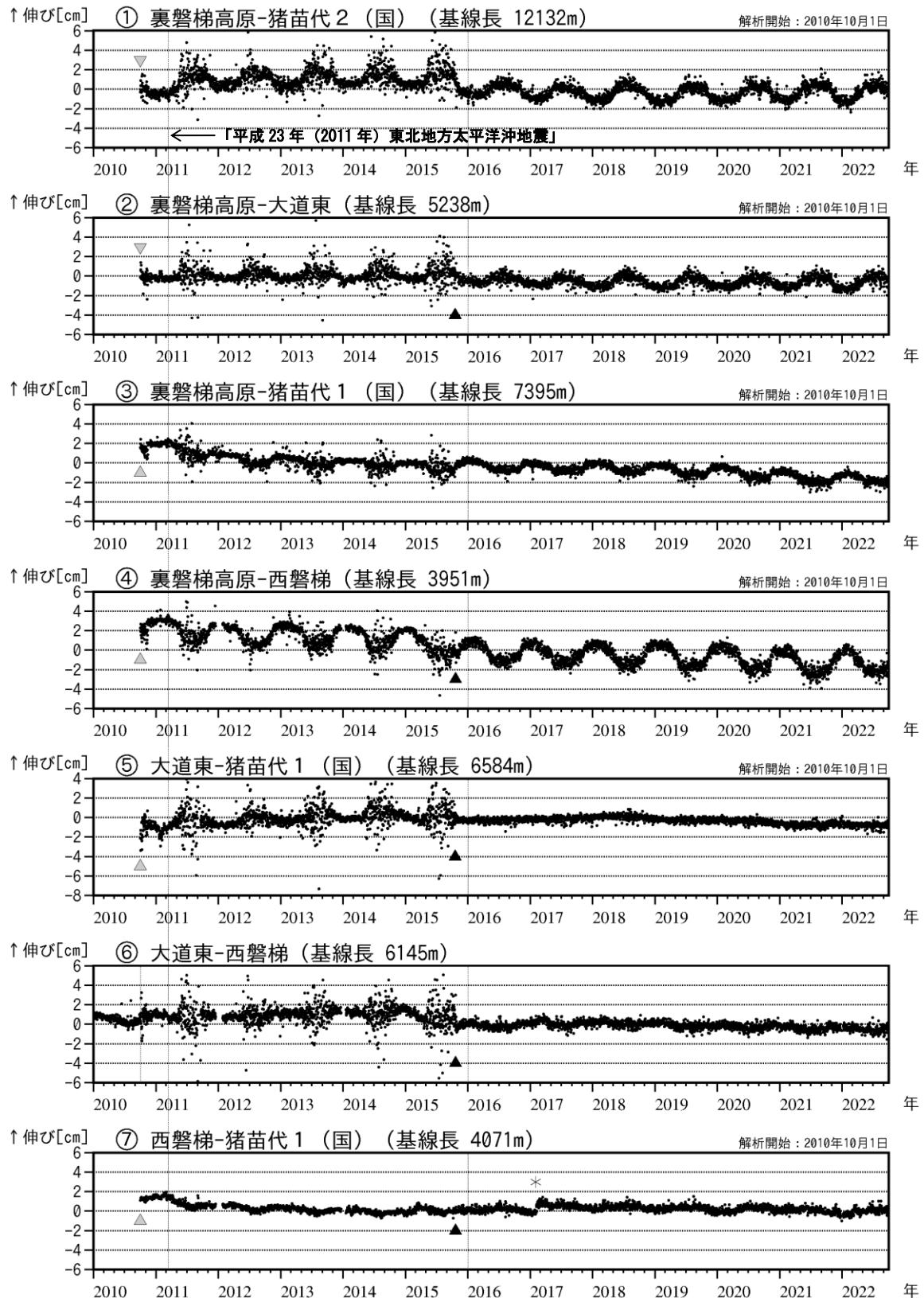
図4 磐梯山 GNSS 基線長変化図 (2010 年 1 月～2022 年 9 月)
