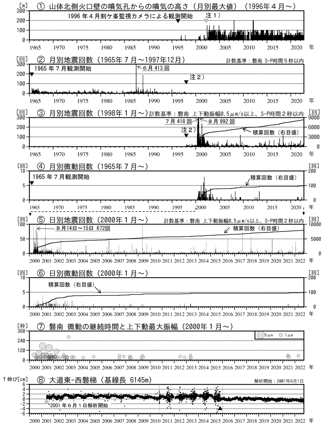
図3 磐梯山 火山活動経過図（1965年7月～2022年9月）
