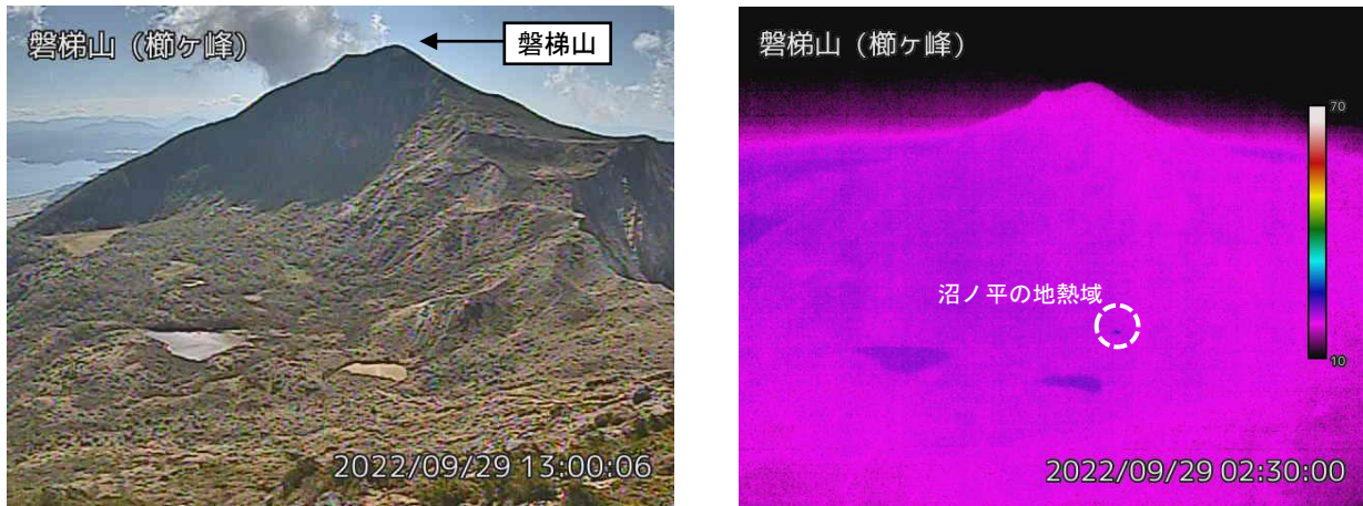
図2 磐梯山 沼ノ平周辺の状況と地表面温度分布（9月29日）
