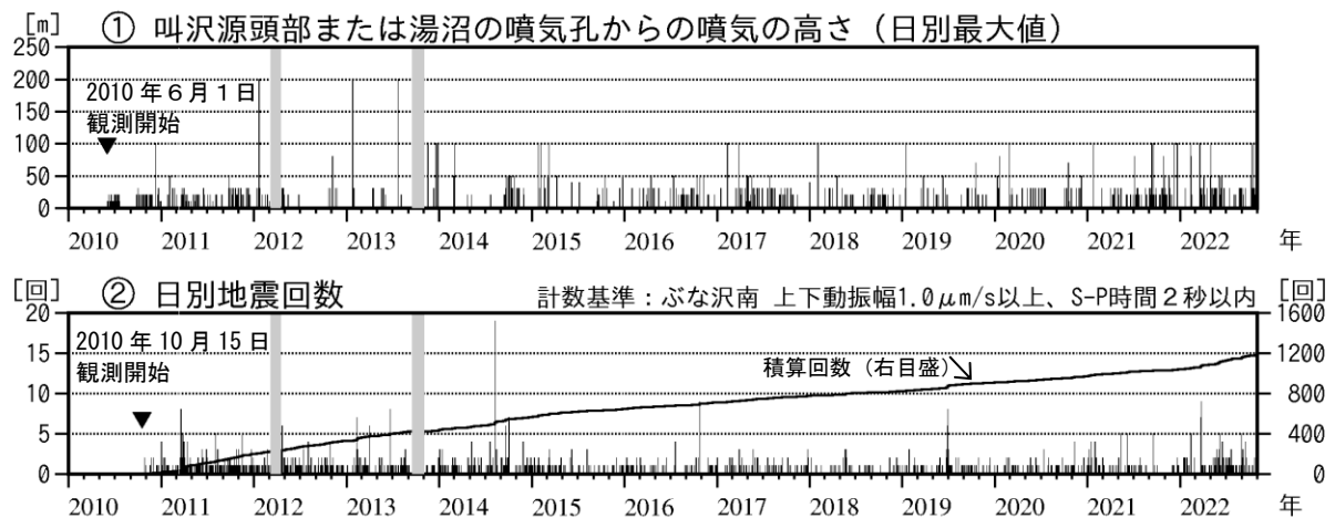
図3 秋田焼山 火山活動経過図（2010年6月～2022年10月）
