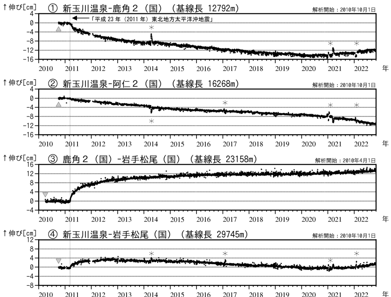
図4 秋田焼山 GNSS 基線長変化図（2010年4月～2022年10月）
