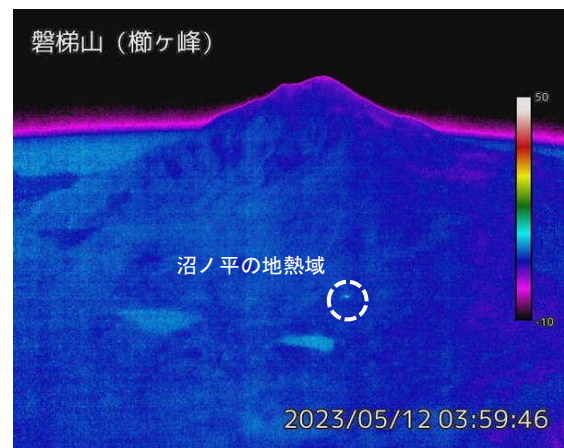
図2 磐梯山 沼ノ平周辺の状況と地表面温度分布（5月12日）
