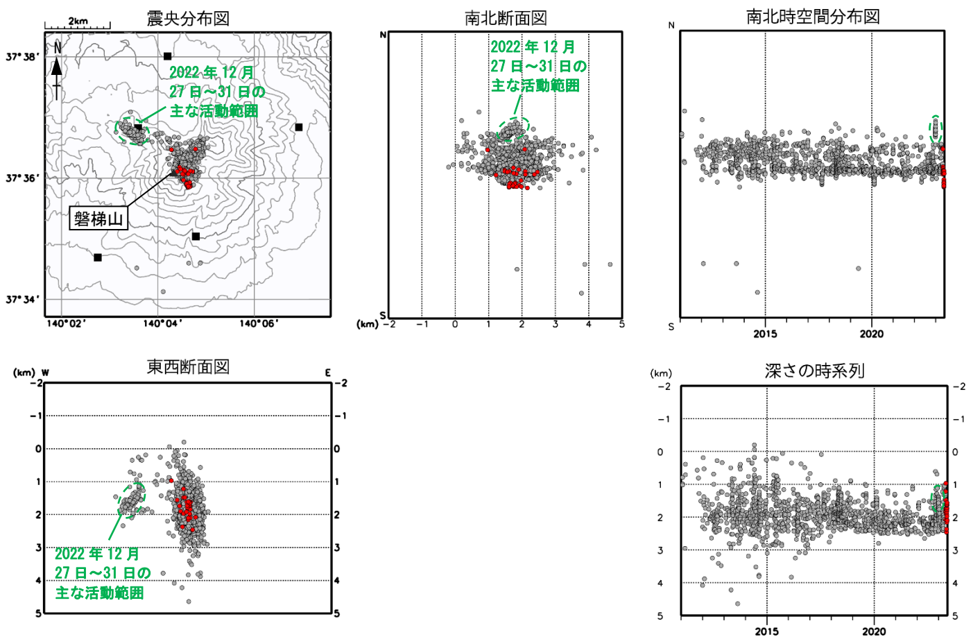
図5 磐梯山 震源分布図（2011年1月～2023年5月）
