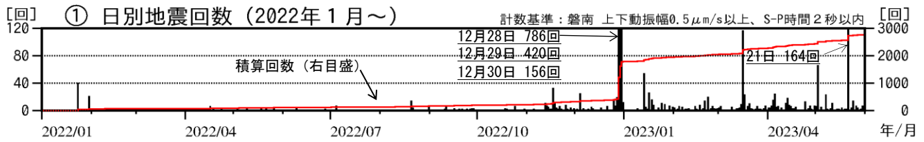
図4 磐梯山 地震回数（2022年1月～2023年5月）
