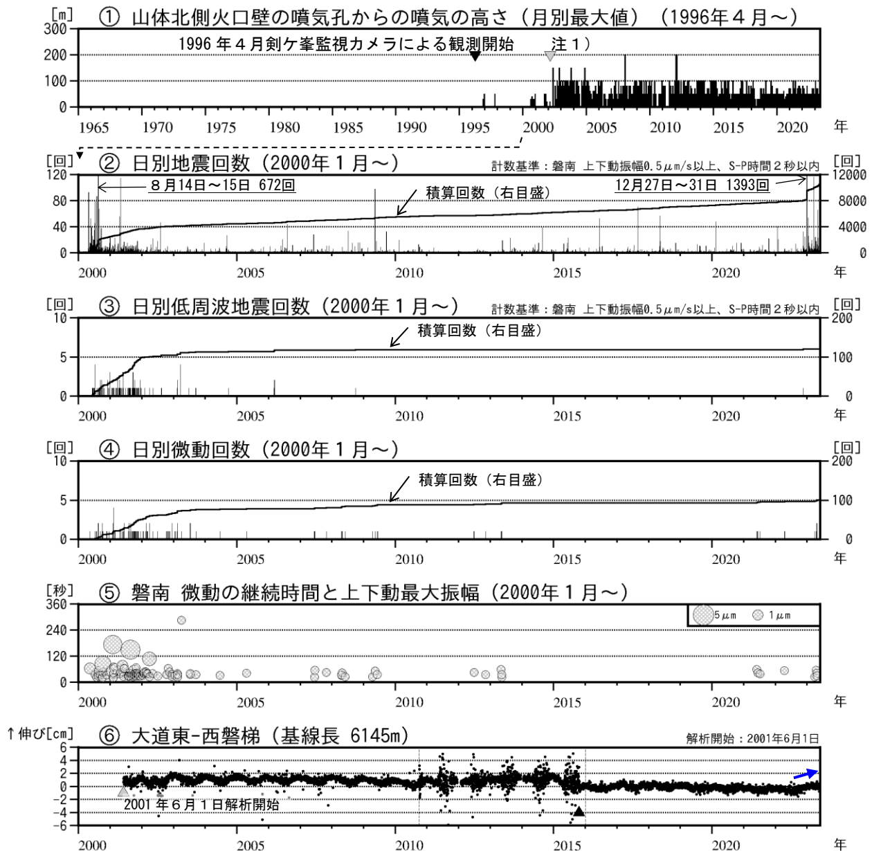
図3 磐梯山 火山活動経過図（1965年7月～2023年5月）
