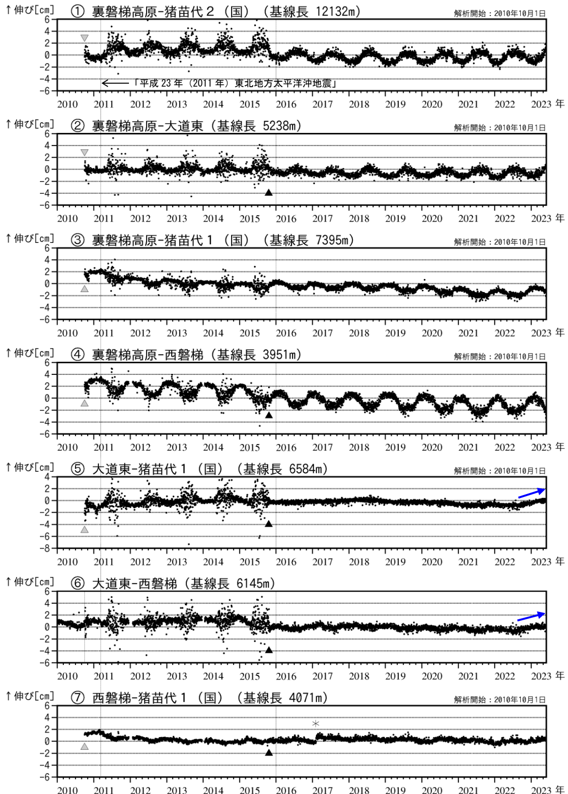
図6 磐梯山 GNSS 基線長変化図（2010年1月～2023年5月）
