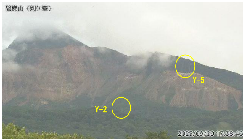
図1 磐梯山 山体北側火口壁の噴気の状況（9月9日）
