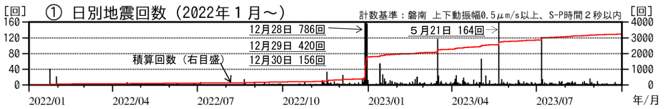
図4 磐梯山 地震回数（2022年1月～2023年9月）
