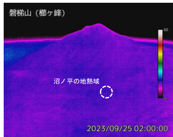
図2 磐梯山 沼ノ平周辺の状況と地表面温度分布（9月25日）
