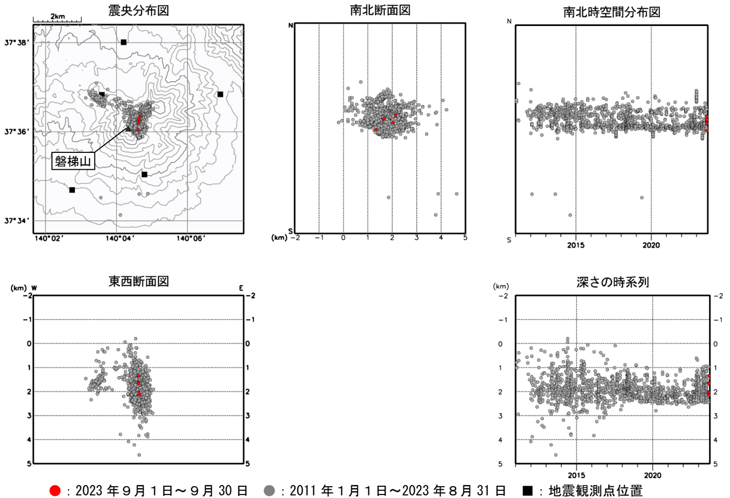
図5 磐梯山 震源分布図（2011年1月～2023年9月）
