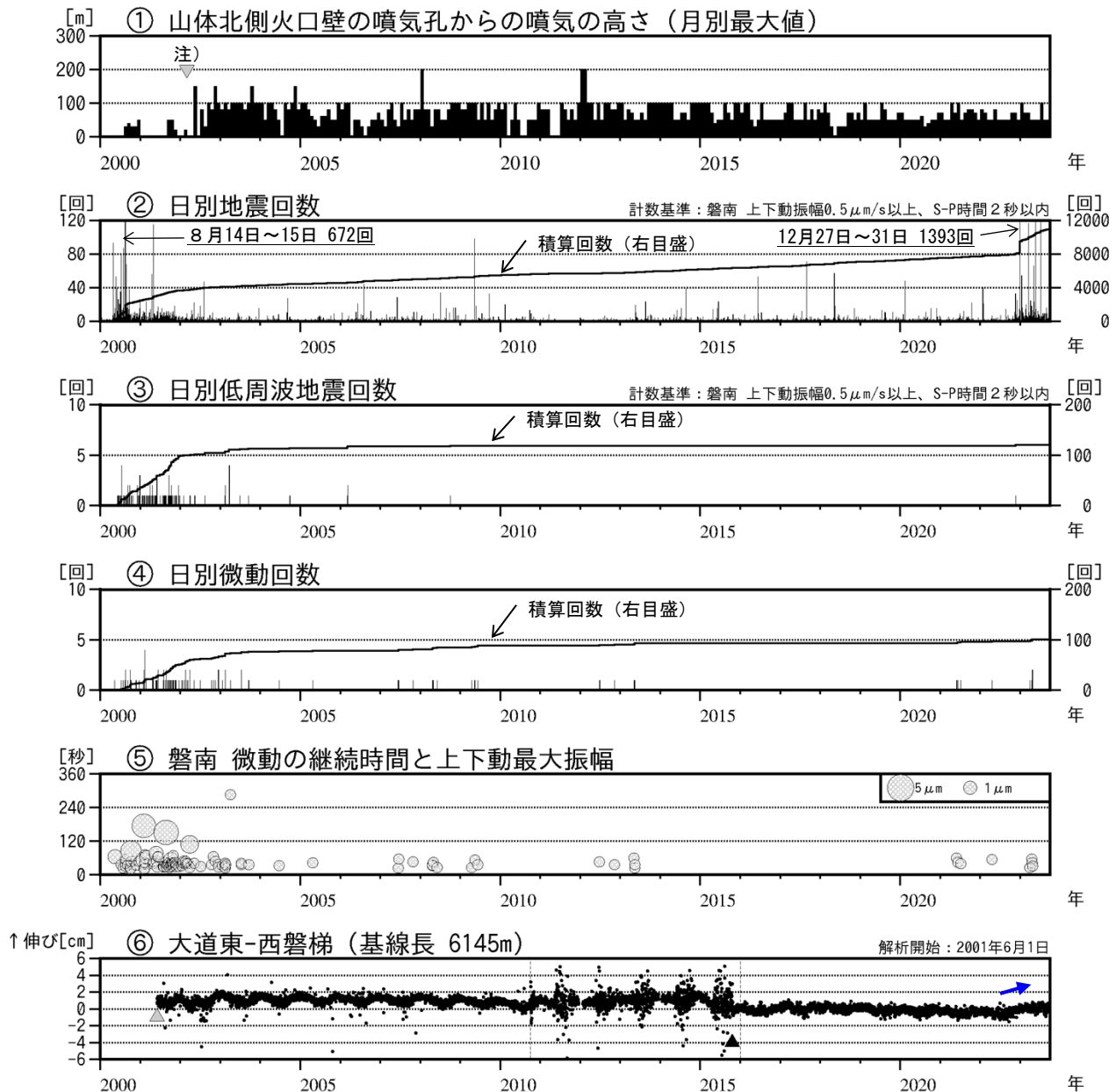
図3 磐梯山 火山活動経過図（2000年1月～2023年9月）
