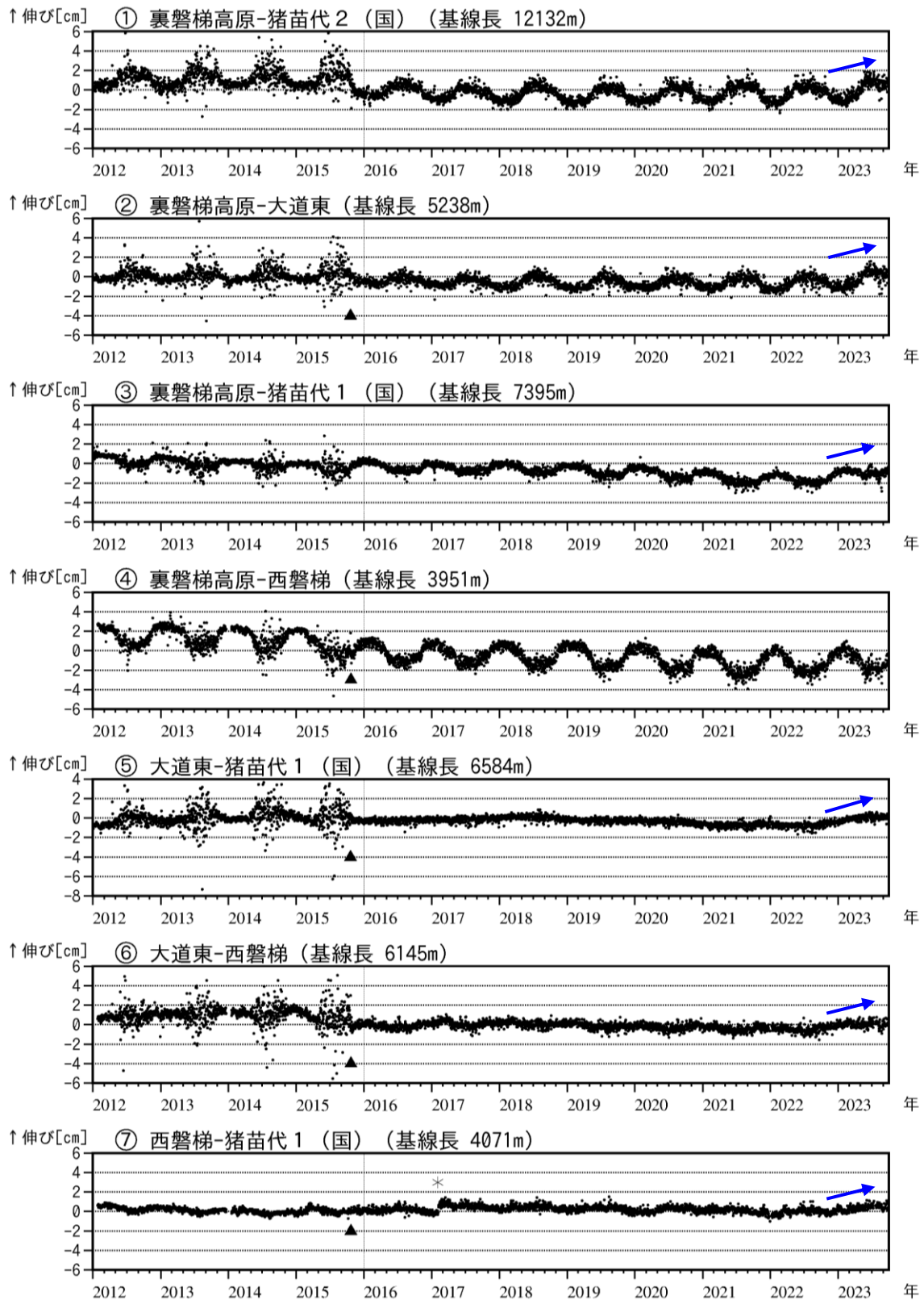
図6 磐梯山 GNSS 基線長変化図 (2012年1月～2023年9月)
