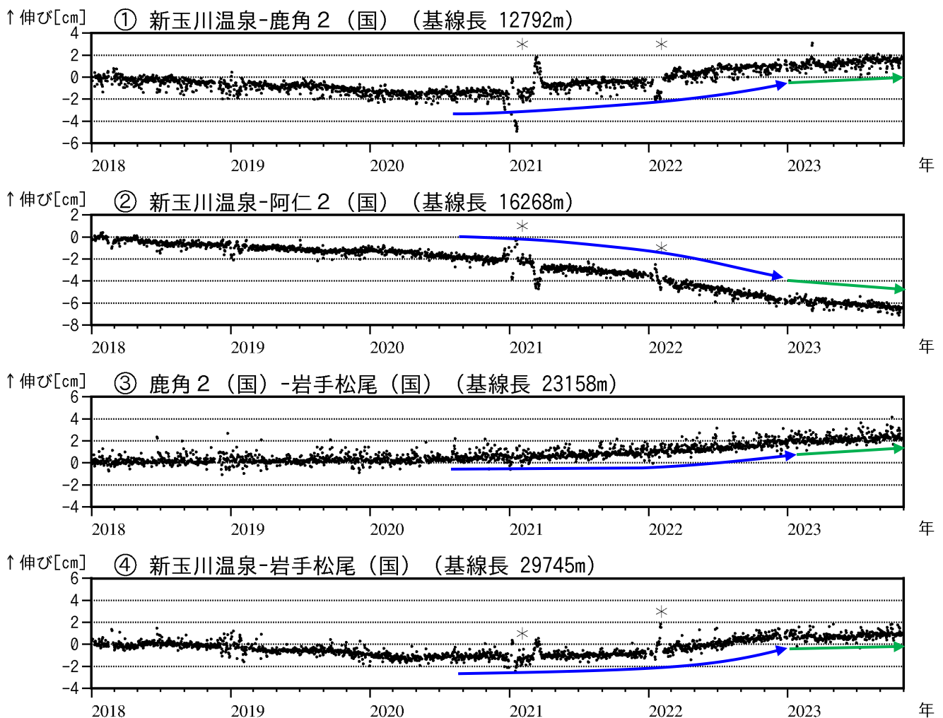
図4 秋田焼山 GNSS 基線長変化図（2018年1月～2023年10月）
