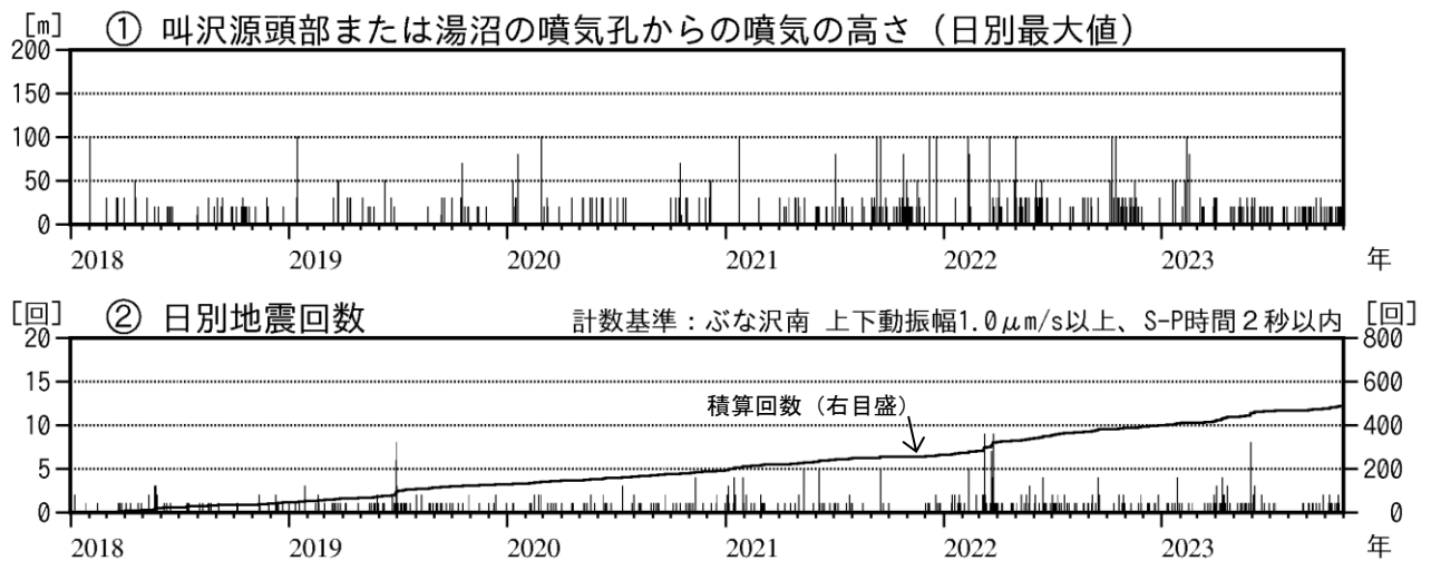
図3 秋田焼山 火山活動経過図（2018年1月～2023年10月）
