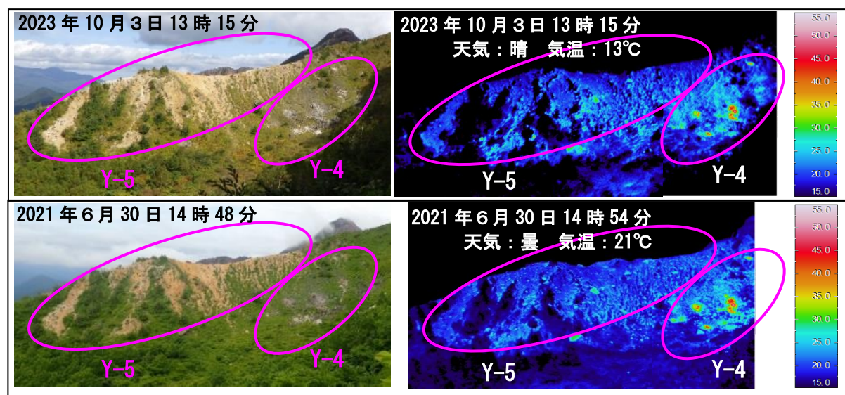
図6 磐梯山 山体北側火口壁噴気地帯（Y-4、Y-5）の状況（左）と地表面温度分布（右） ※日射の影響により、裸地等では表面温度が高めに表示されています。
