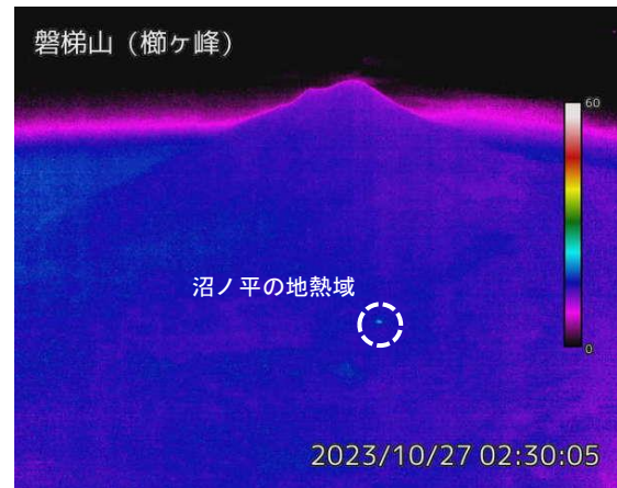
図2 磐梯山 沼ノ平周辺の状況と地表面温度分布（10月27日）
