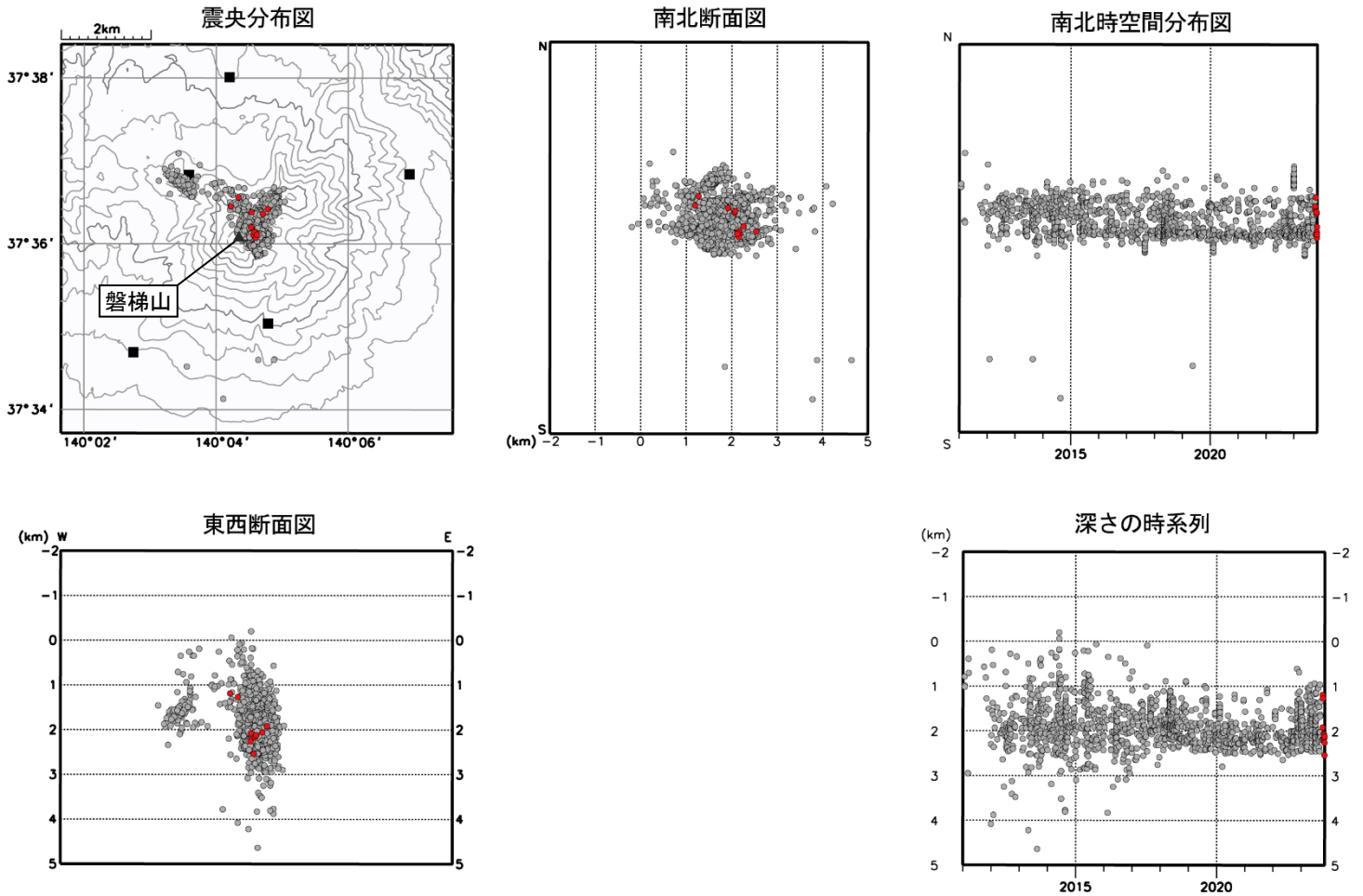
図9 磐梯山 震源分布図（2011年1月～2023年10月）
