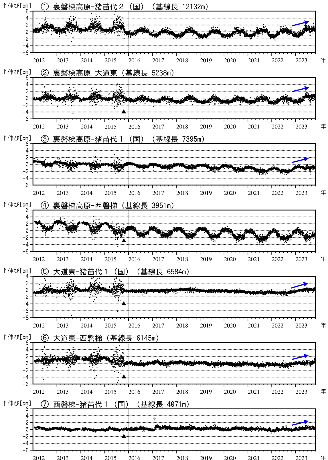
図10 磐梯山 GNSS基線長変化図（2012年1月～2023年10月）
