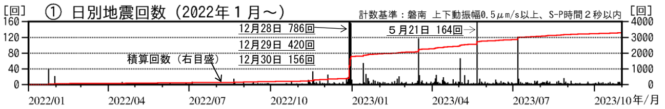
図8 磐梯山 地震回数（2022年1月～2023年10月）
