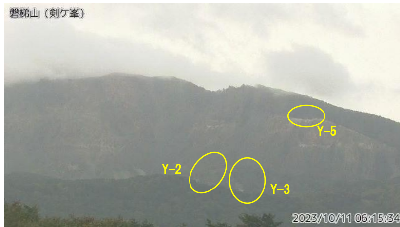
図1 磐梯山 山体北側火口壁の噴気の状態（10月11日）
