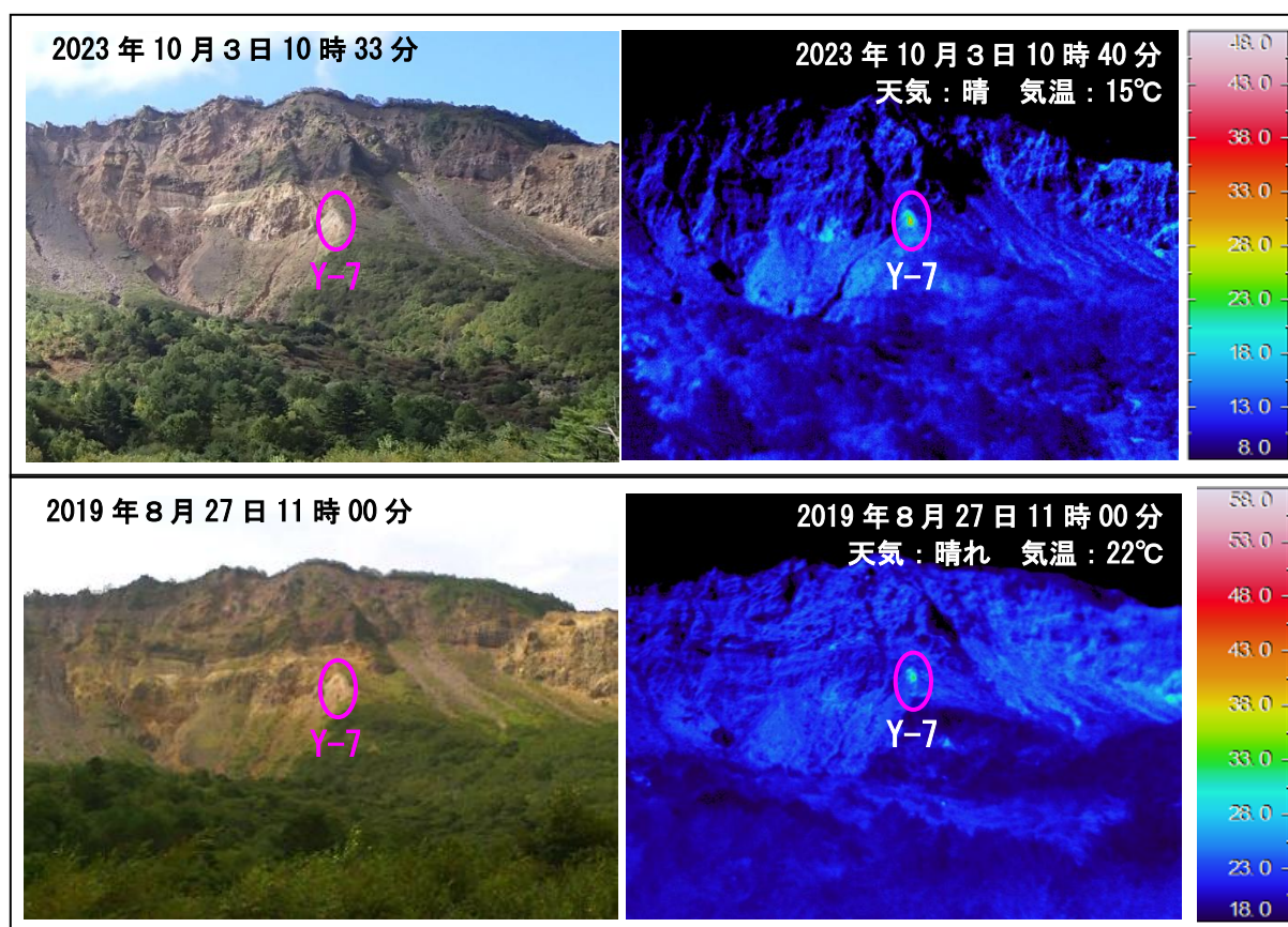
図5 磐梯山 山体北側火口壁噴気地帯（Y-7）の状況（左）と地表面温度分布（右） ※日射の影響により、裸地等では表面温度が高めに表示されています。
