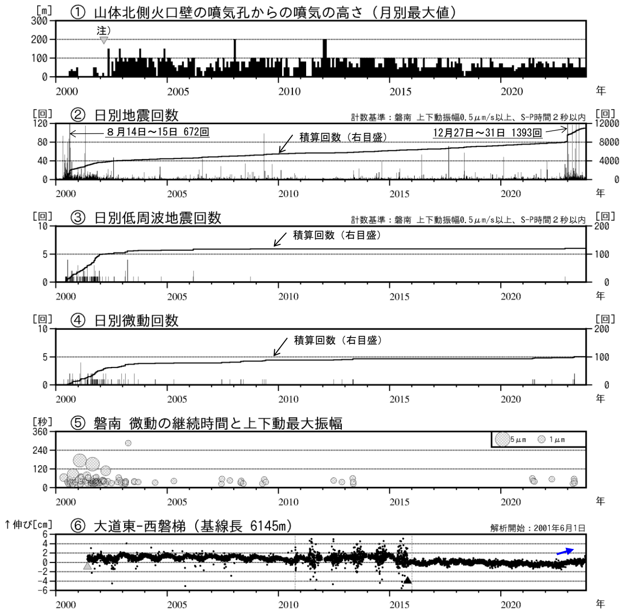
図7 磐梯山 火山活動経過図（2000年1月～2023年10月）
