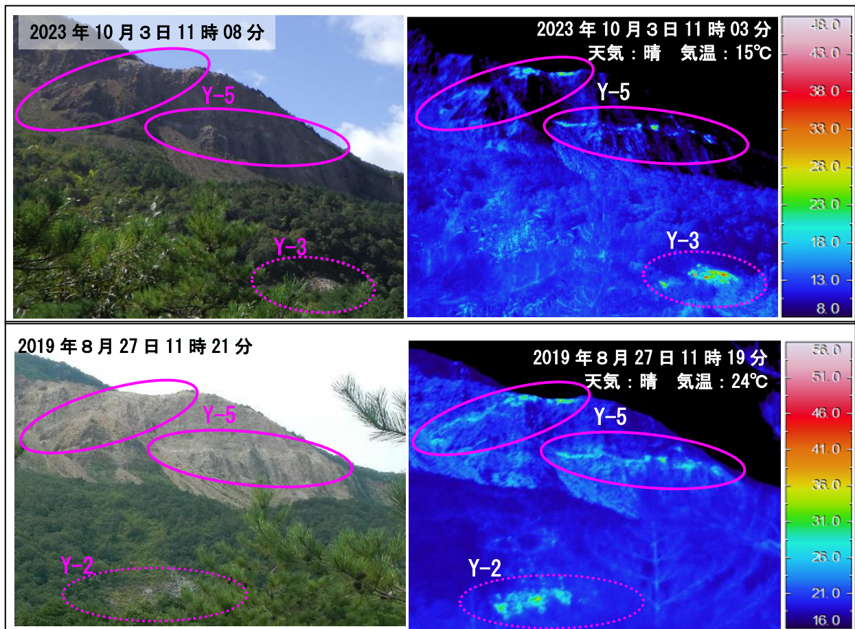
図4 磐梯山 山体北側火口壁噴気地帯（Y-2、3及びY-5）の状況（左）と地表面温度分布（右）
