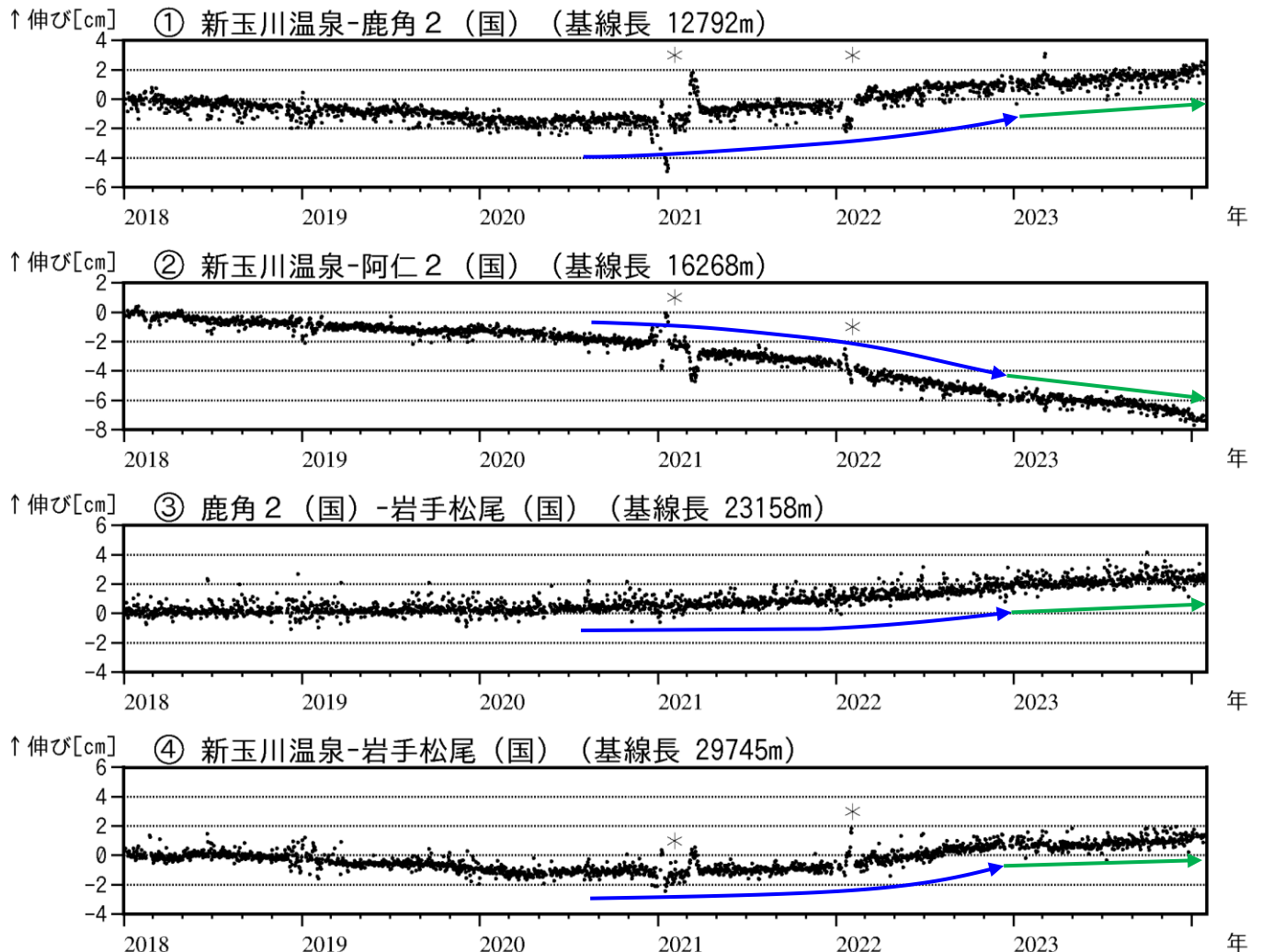
図4 秋田焼山 GNSS 基線長変化図（2018年1月～2024年1月）
