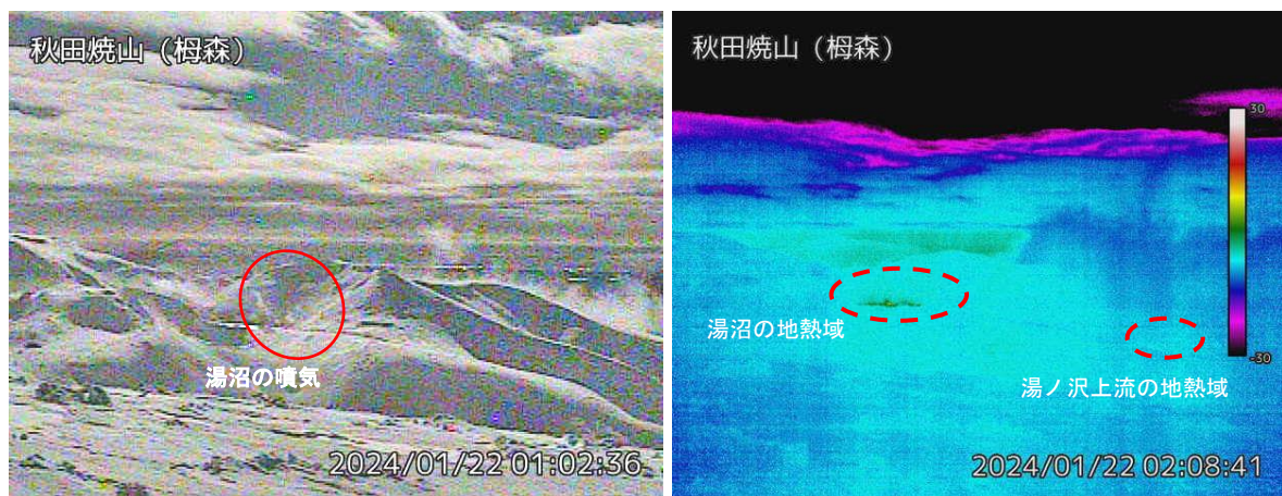
図2 秋田焼山 湯沼と湯ノ沢上流の状況と地表面温度分布（1月22日）
