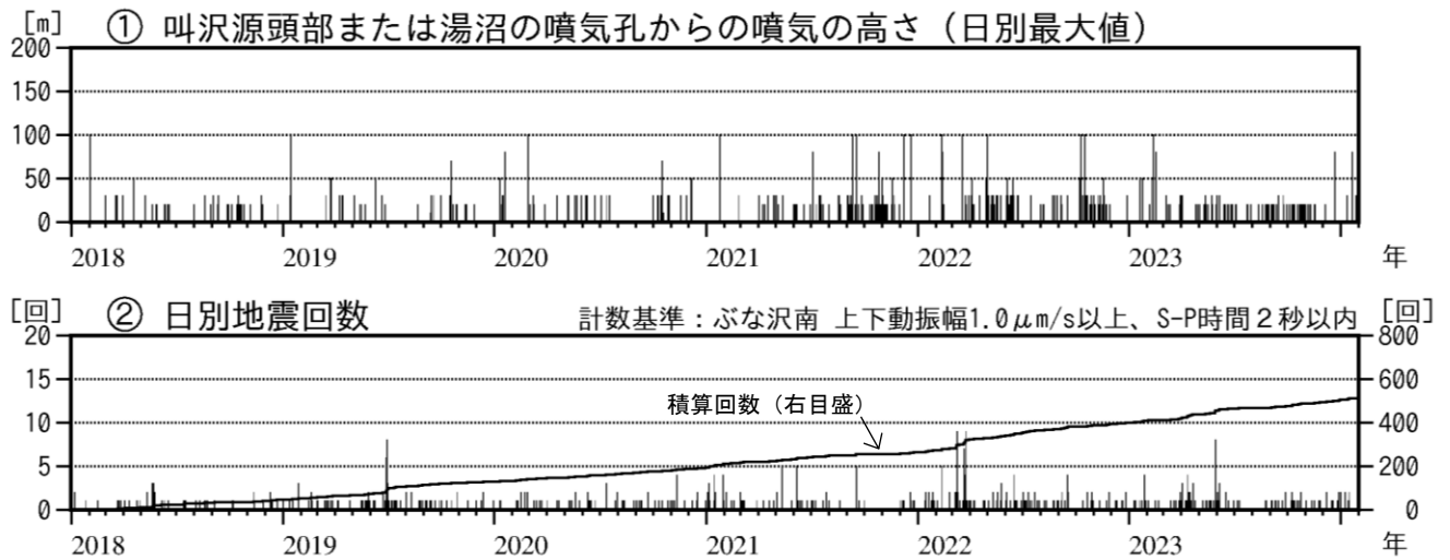
図3 秋田焼山 火山活動経過図（2018年1月～2024年1月）
