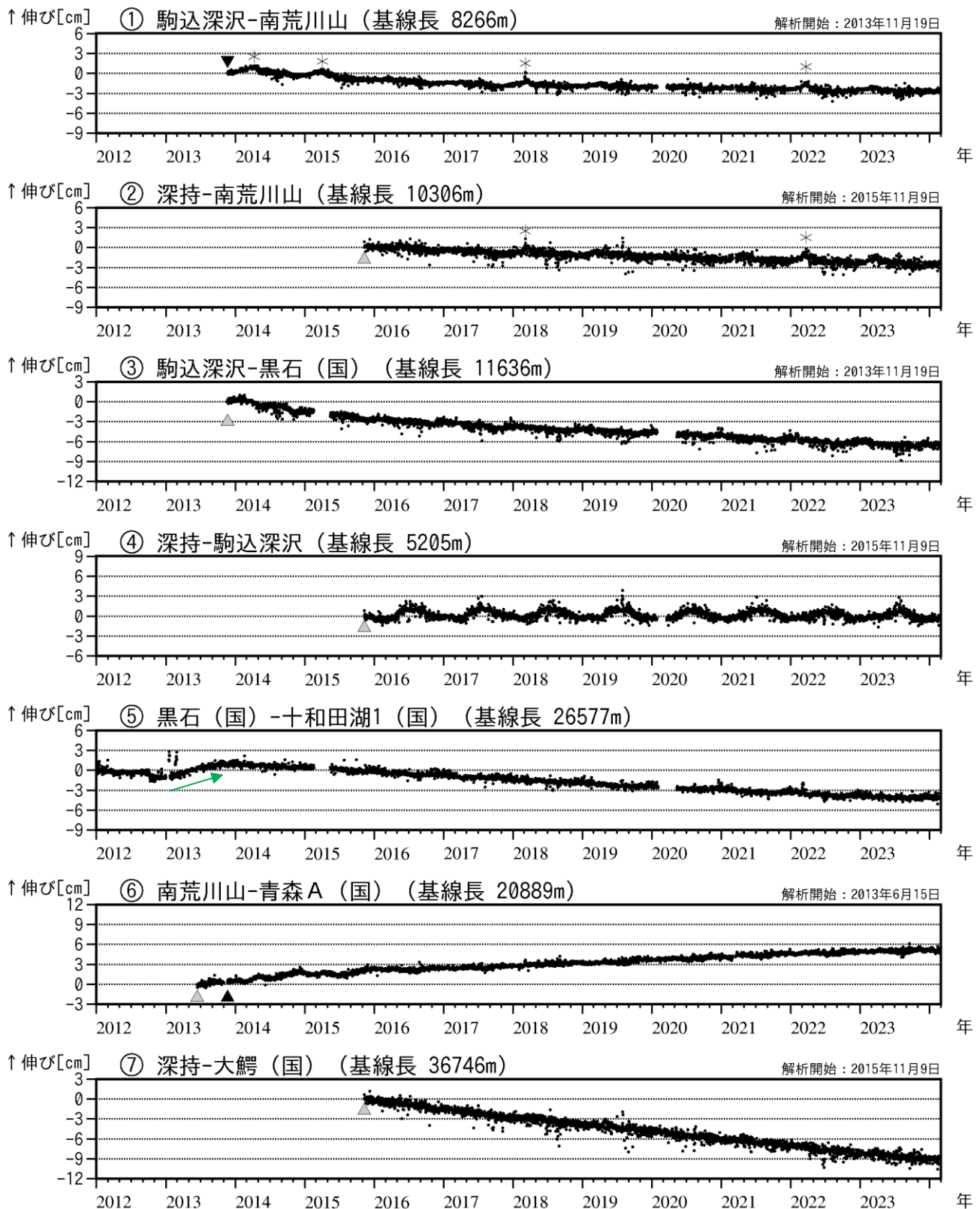
図3 八甲田山 GNSS 基線長変化図（2012年1月～2024年2月）
