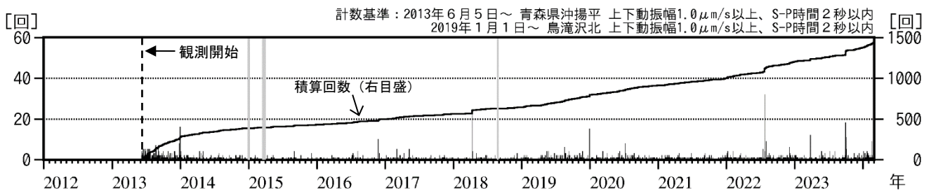
図2 八甲田山 日別地震回数（2013年6月～2024年2月）
