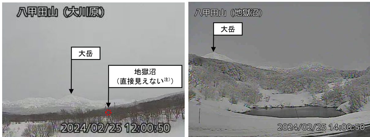
図1 八甲田山 山頂部及び地獄沼周辺の状況（2月25日）
