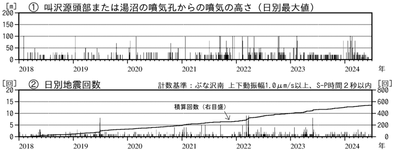
図3 秋田焼山 火山活動経過図（2018年1月～2024年6月）
