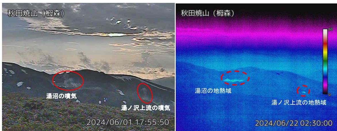
図2 秋田焼山 湯沼と湯ノ沢上流の様（6月1日）と地表面温度分布（6月22日）
