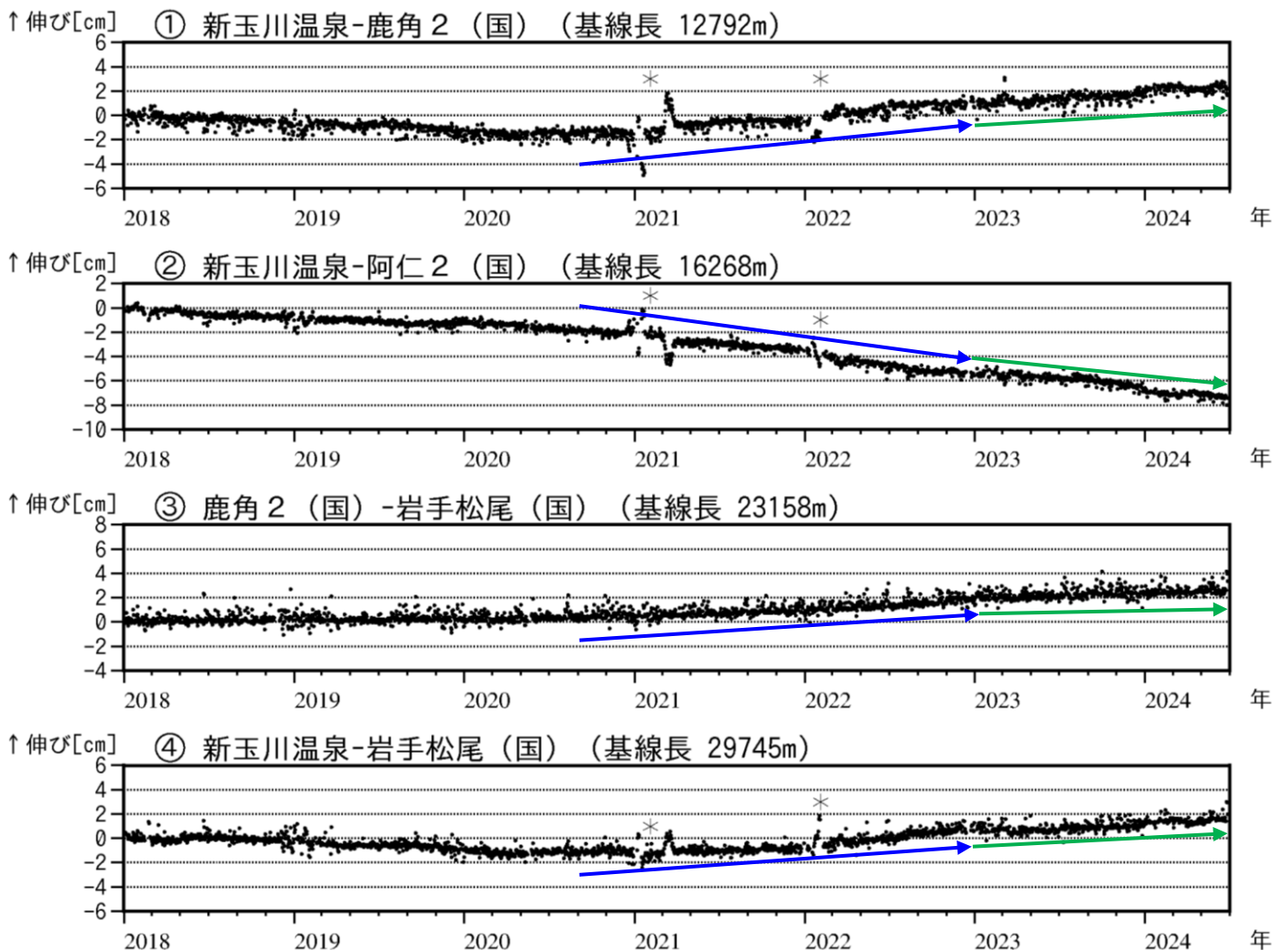
図4 秋田焼山 GNSS 基線長変化図（2018年1月～2024年6月）
