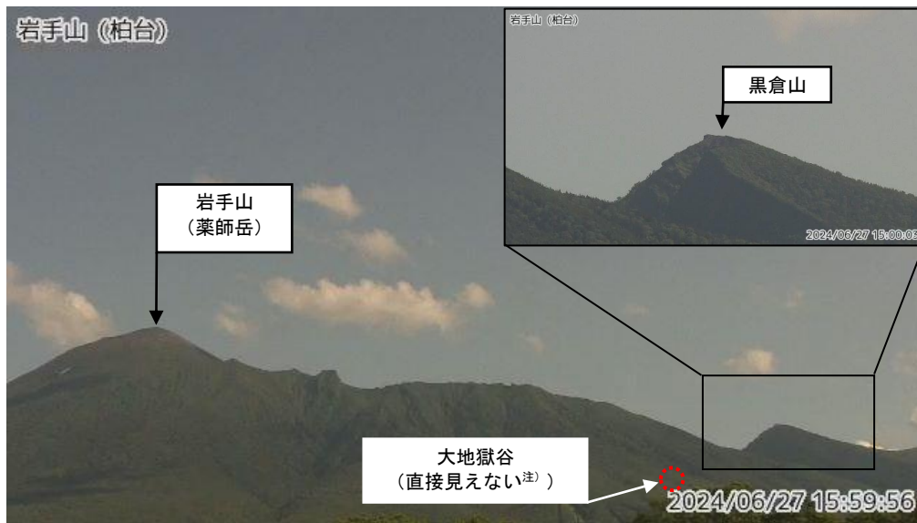
図1 岩手山 山頂部から黒倉山周辺の状況（6月27日）
