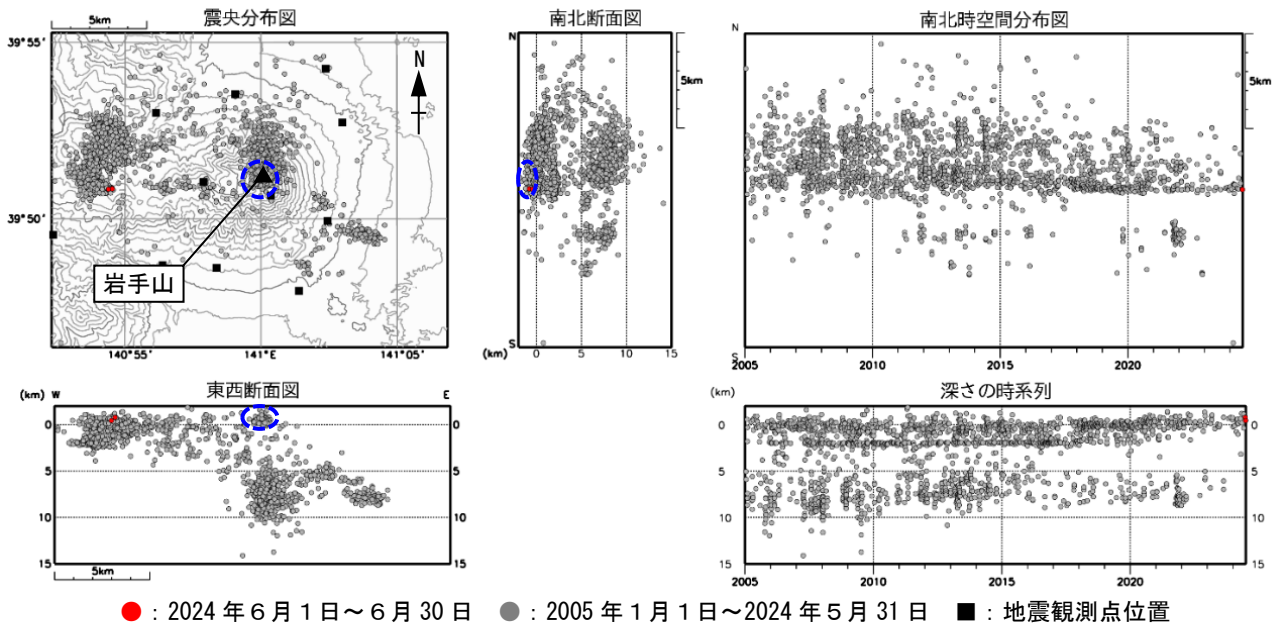
図4 岩手山 地震活動（2005 年 1 月～2024 年 6 月）
