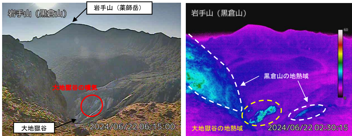
図2 岩手山 黒倉山監視カメラからの状況と地表面温度分布（6月22日）
