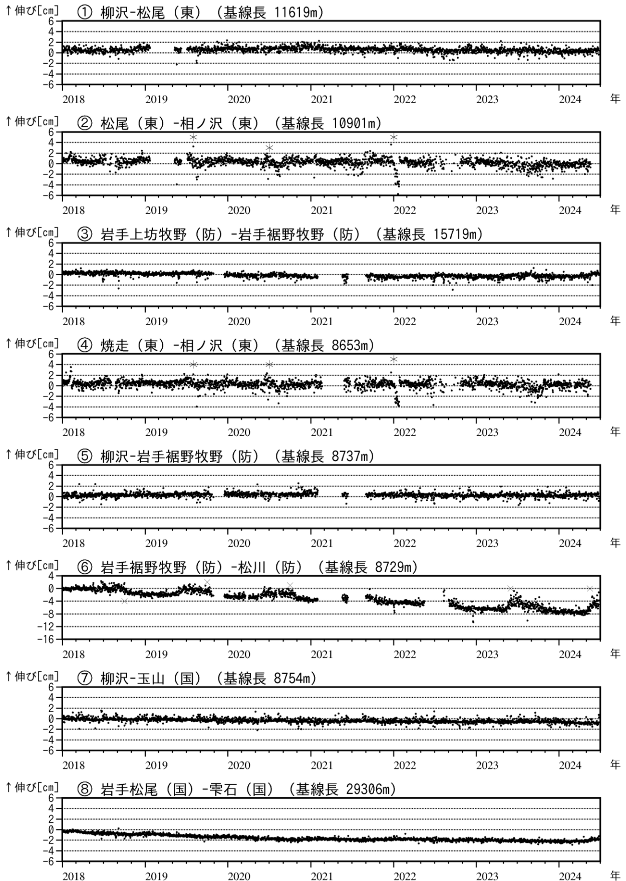
図5 岩手山 GNSS 基線長変化図（2018年1月～2024年6月）
