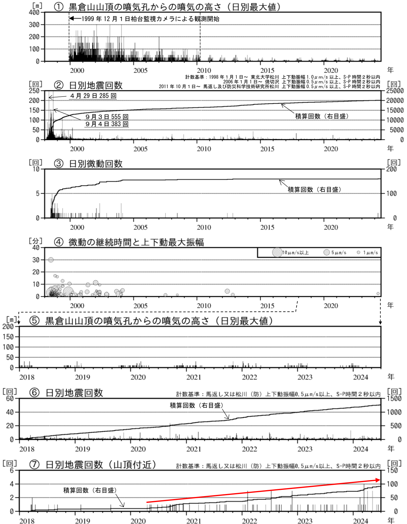
図3 岩手山 火山活動経過図（1998年1月～2024年6月）
