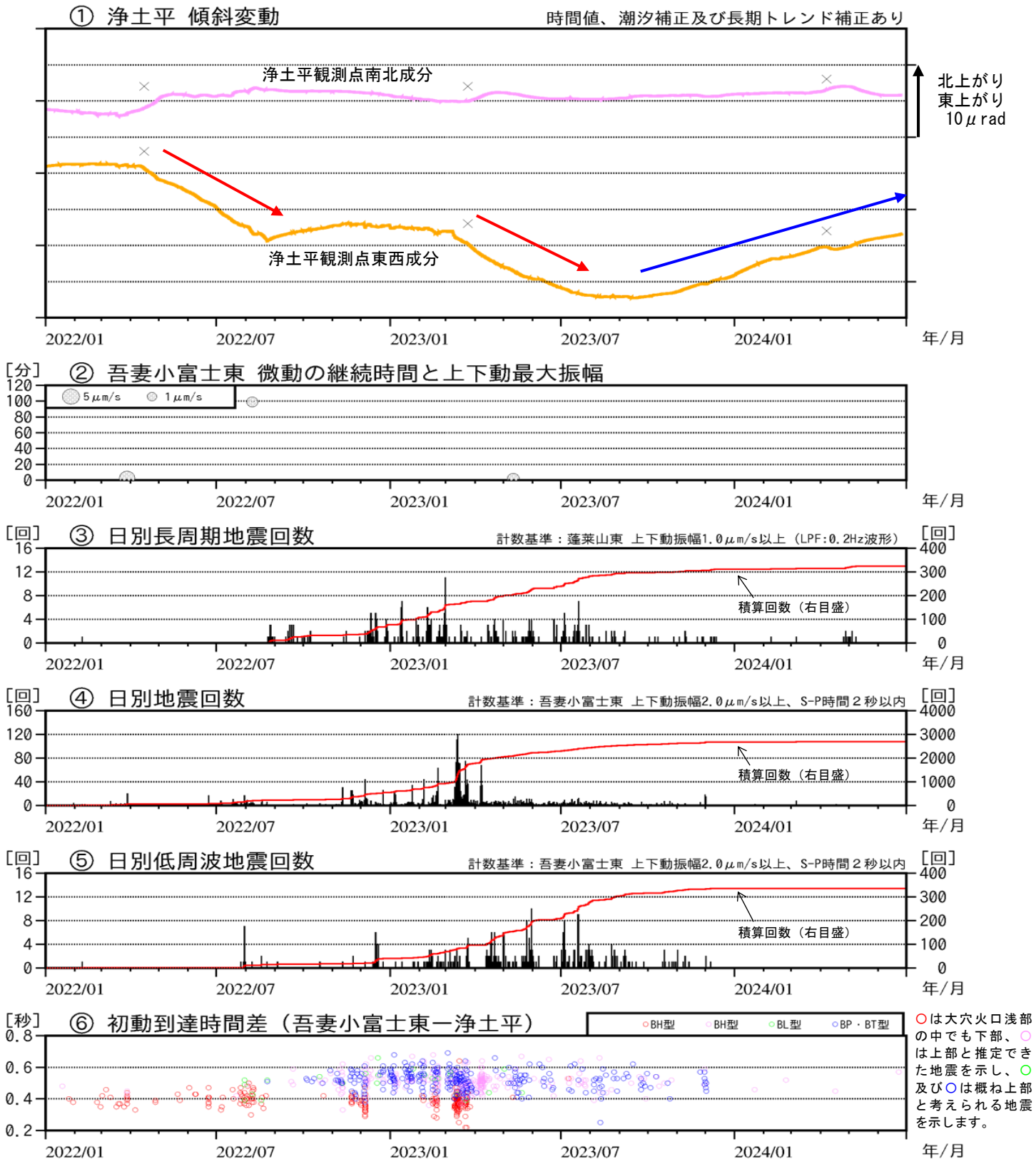
図3 吾妻山 火山活動経過図（2022年1月～2024年6月）
