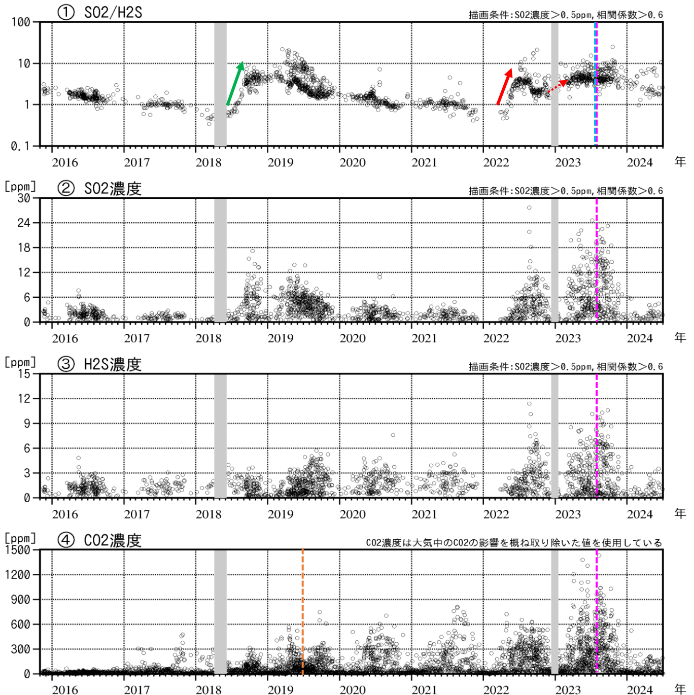
図10 吾妻山 火山ガス観測装置による観測（2015年11月～2024年6月）
