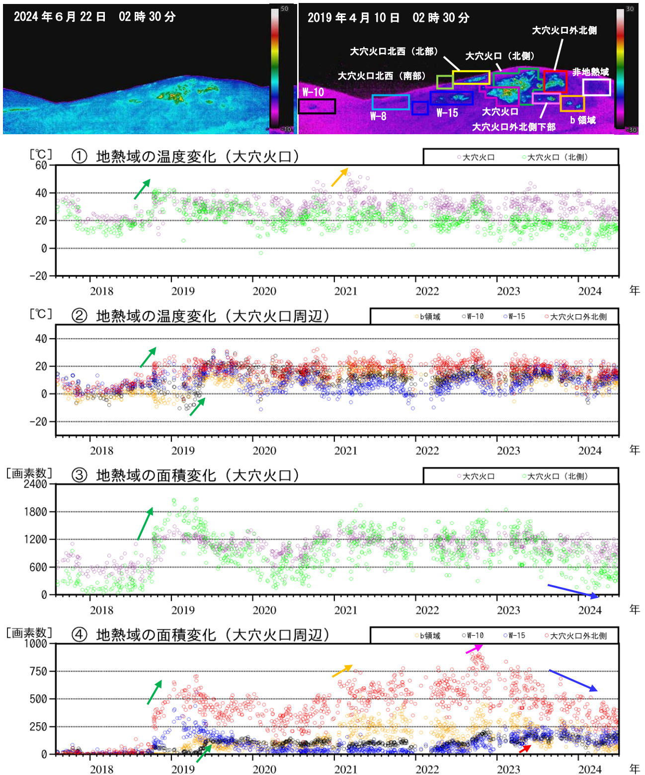
図5 吾妻山 監視カメラによる大穴火口周辺の地熱域の経過（2017年8月～2024年6月）
