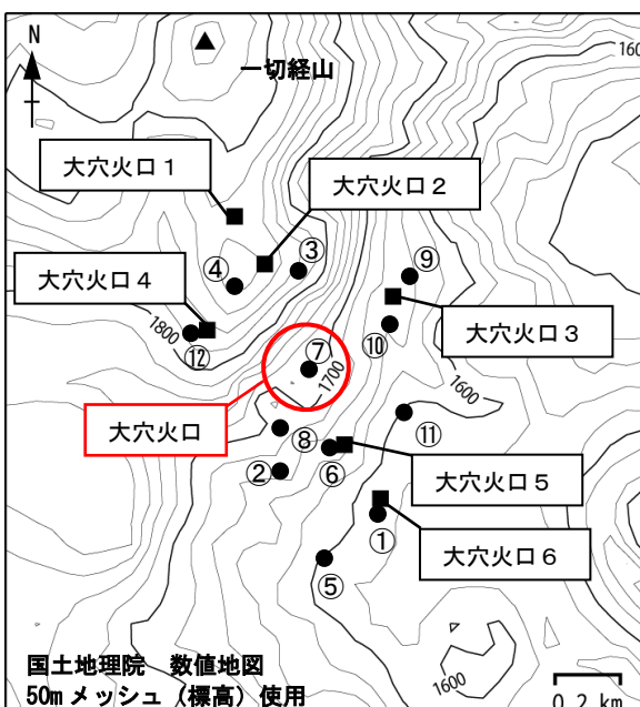
図 15 吾妻山 全磁力観測点配置図
