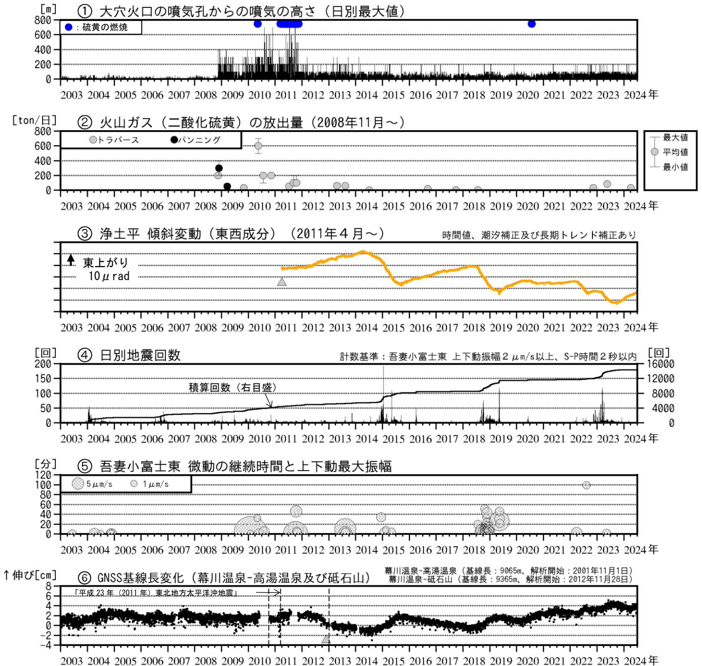
図2 吾妻山 中期的な火山活動の経過（2003年1月～2024年6月）
