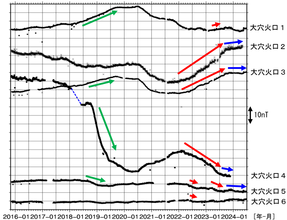
図 11 吾妻山 全磁力連続観測点の全磁力値変化（2015 年 11 月～2024 年 6 月）
