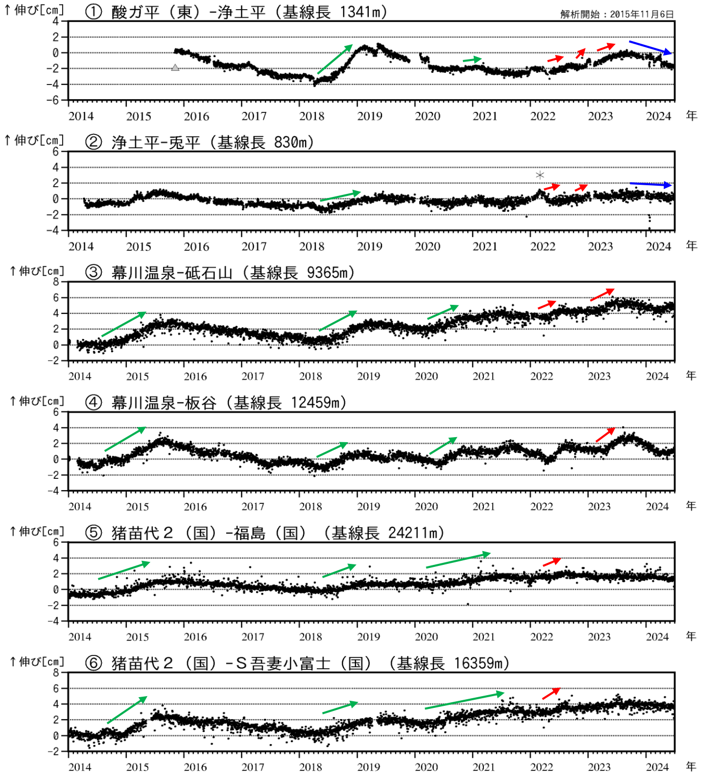
図4 吾妻山 吾妻山浅部・深部の地殻変動（2014年1月～2024年6月）
