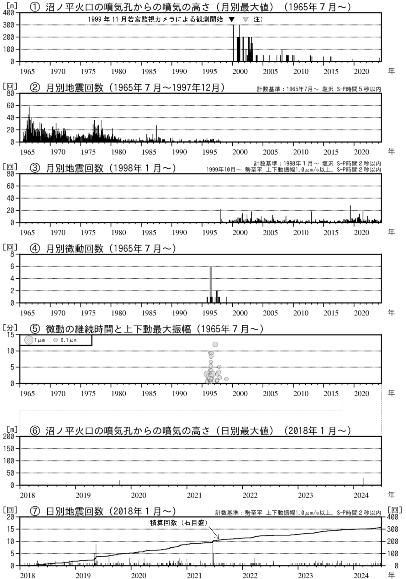
図5 安達太良山 火山活動経過図（1965年7月～2024年6月）
