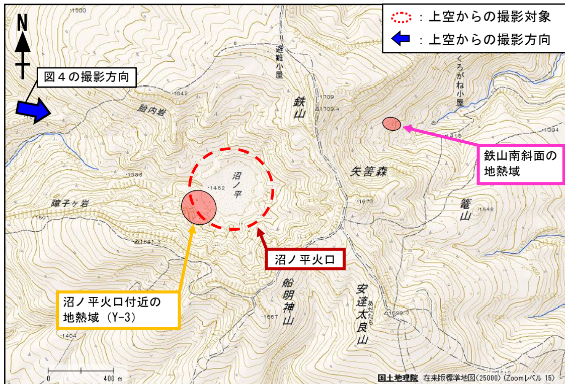
図3 安達太良山 地熱域の分布及び写真撮影方向
