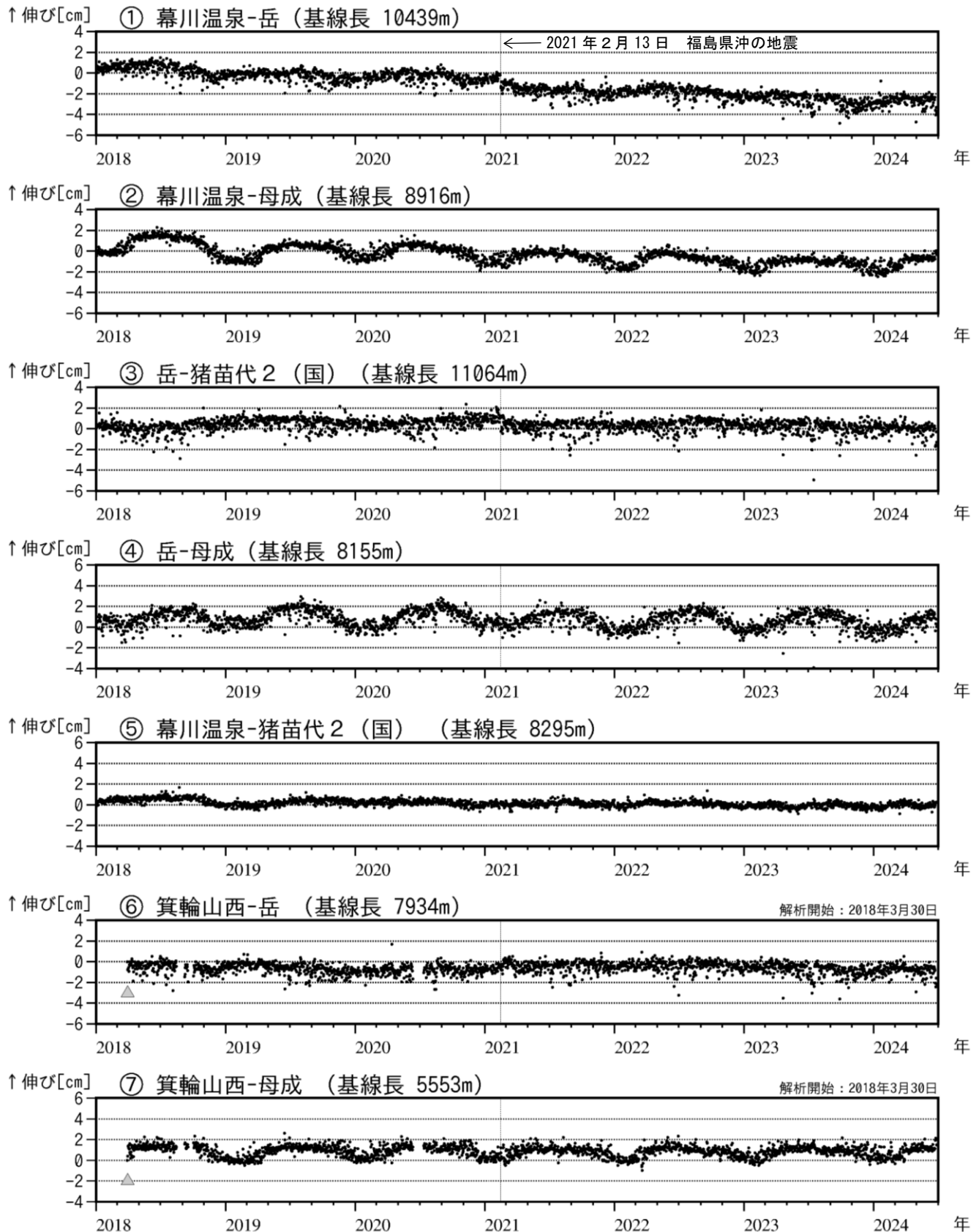
図6 安達太良山 GNSS 基線長変化図 (2018年1月～2024年6月)
