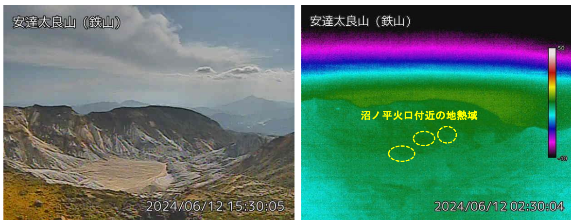
図2 安達太良山 沼ノ平火口周辺の状況と地表面温度分布の状況（6月12日） ・鉄山監視カメラ（沼ノ平火口の北東約700m）の映像です。
