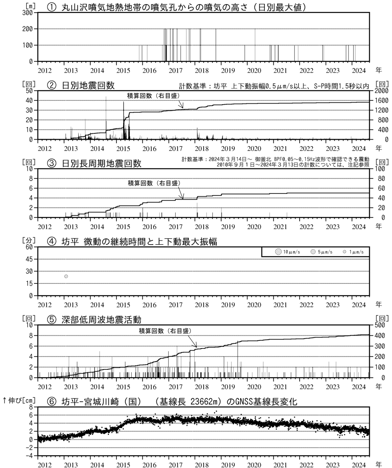
図4 蔵王山 火山活動経過図（2012年1月～2024年8月）
