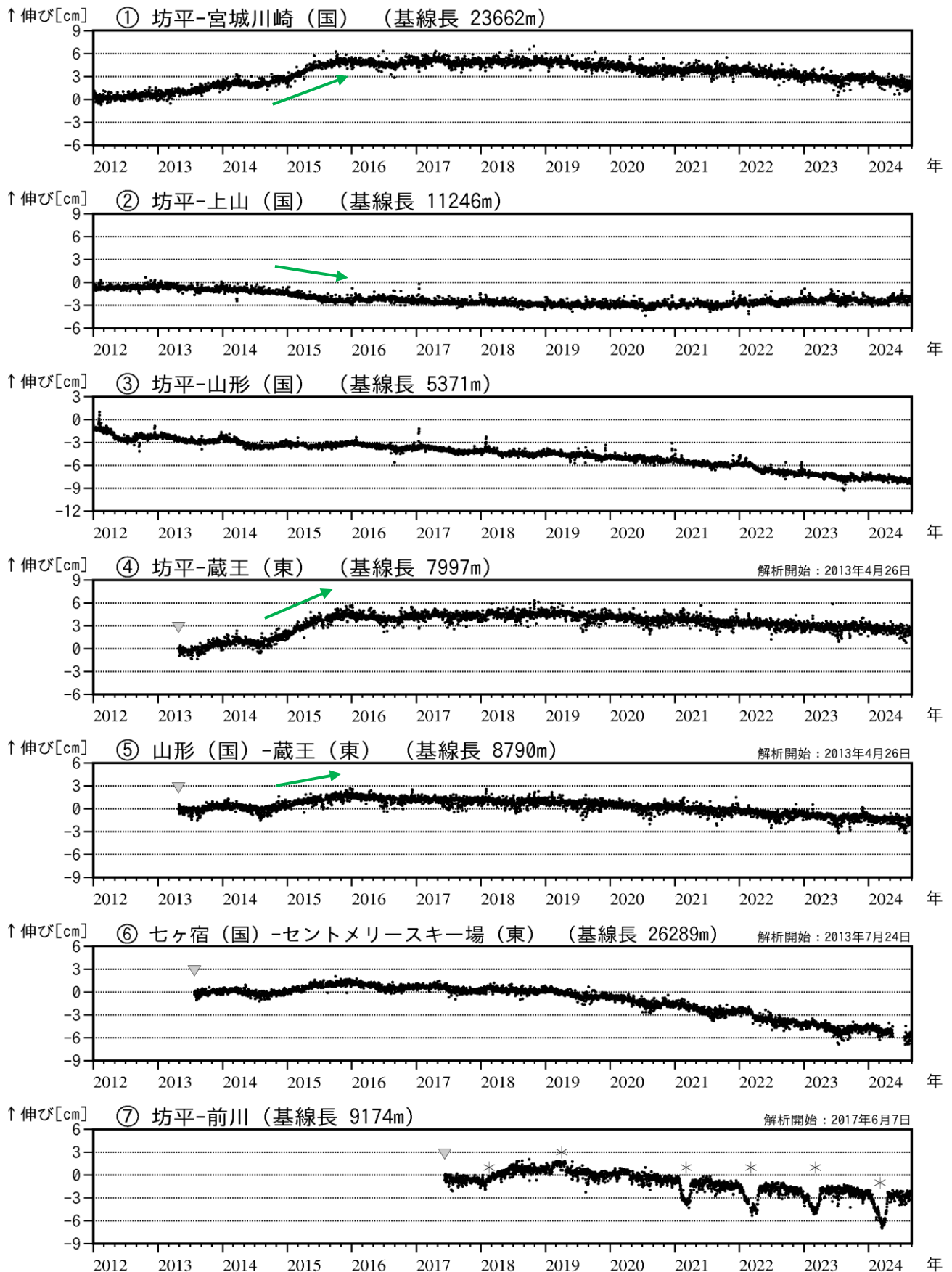
図5 蔵王山 GNSS 基線長変化図 (2012年1月~2024年8月)
