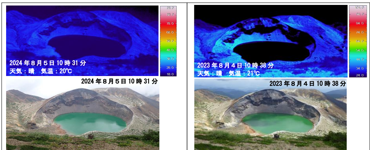
図3 蔵王山 西から撮影した御釜周辺の状況（下段）と地表面温度分布（上段）
