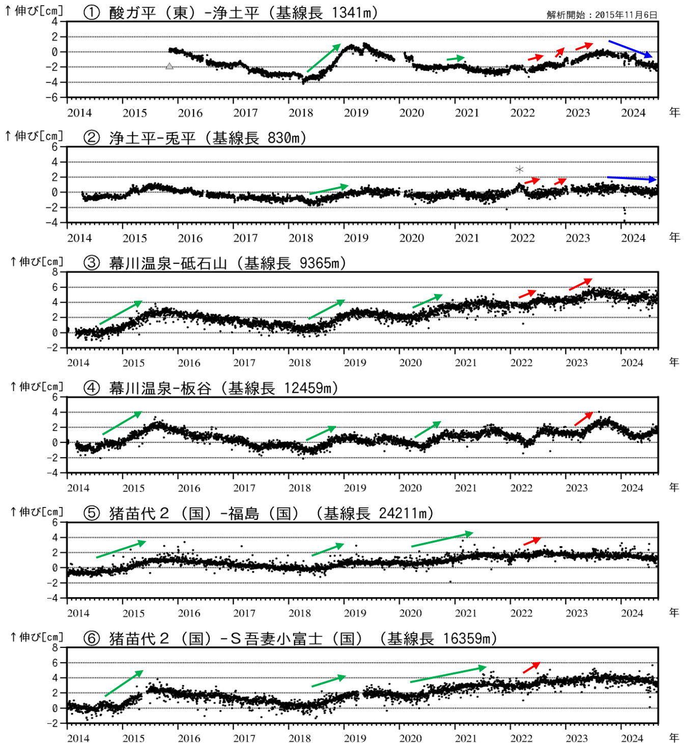
図4 吾妻山 吾妻山浅部・深部の地殻変動（2014年1月～2024年8月）
