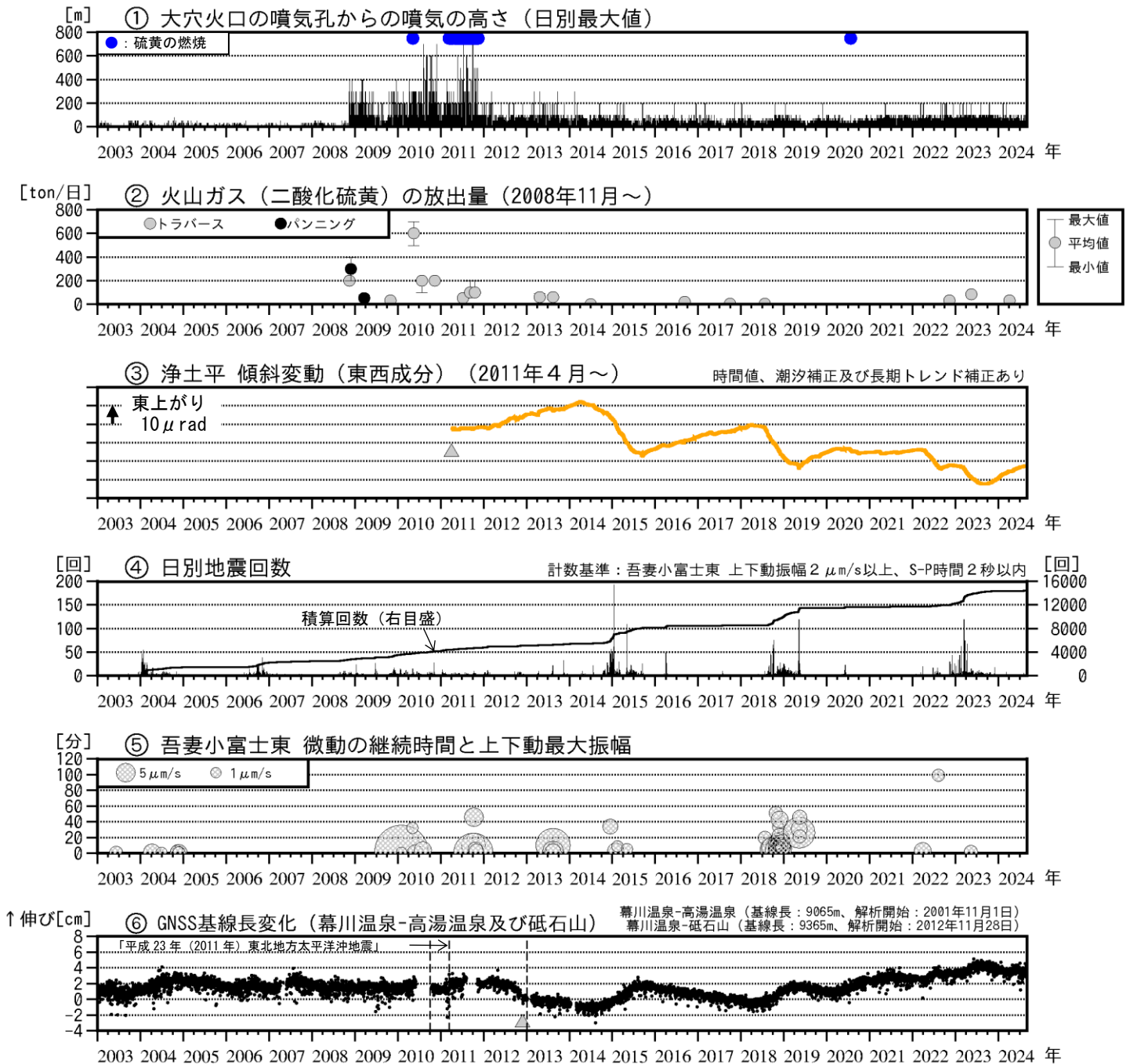
図2 吾妻山 中期的な火山活動の経過（2003年1月～2024年8月）
