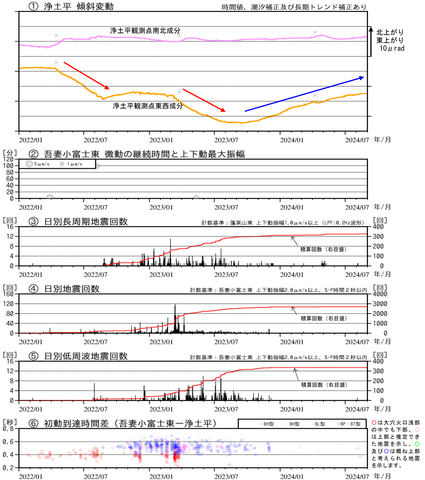
図3 吾妻山 火山活動経過図（2022年1月～2024年8月）
