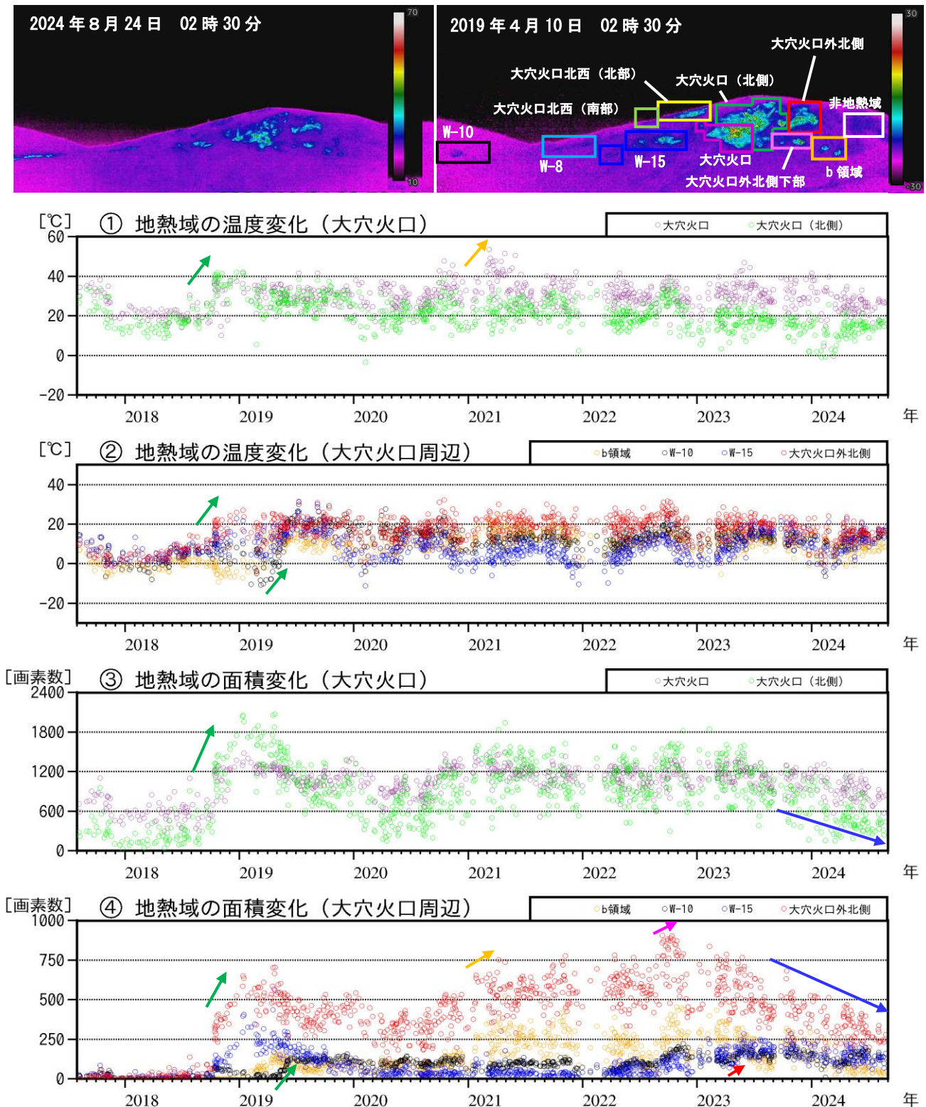
図5 吾妻山 監視カメラによる大穴火口周辺の地熱域の経過（2017年8月～2024年8月）
