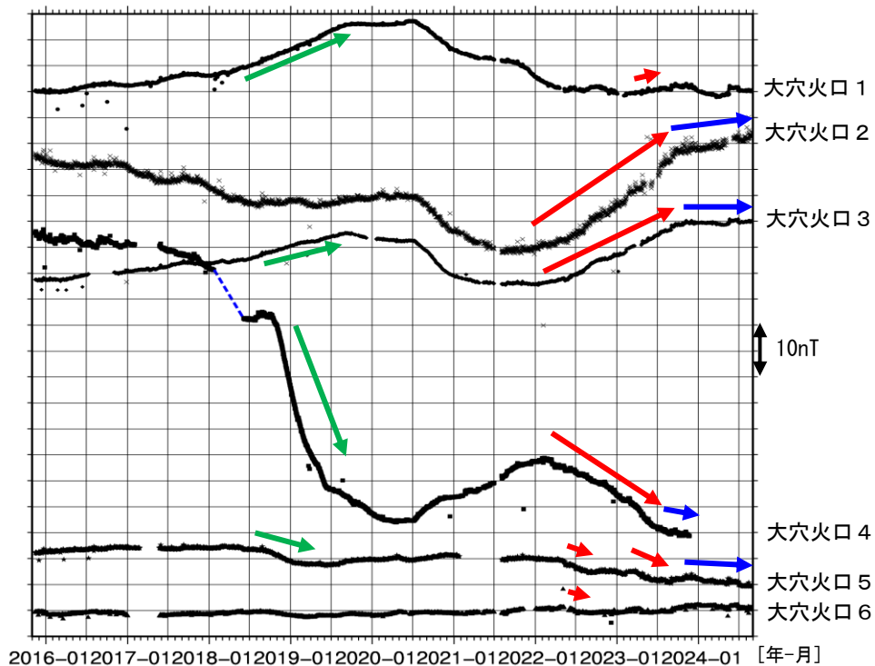
図7 吾妻山 全磁力連続観測点の全磁力値変化（2015年11月～2024年8月）
