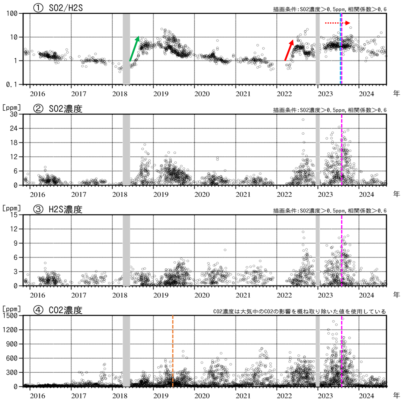
図6 吾妻山 火山ガス観測装置による観測（2015年11月～2024年8月）
