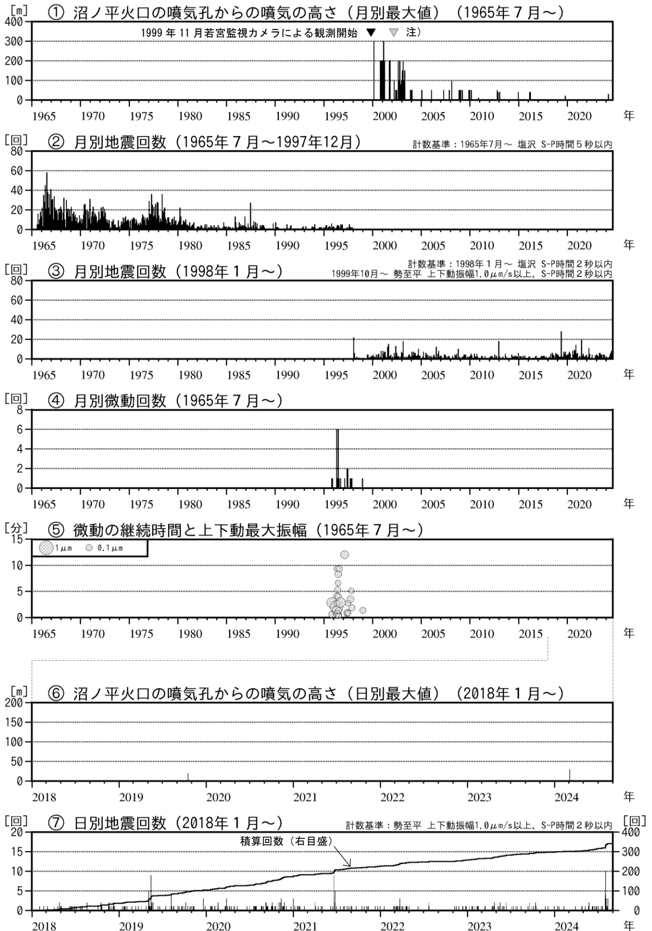
図3 安達太良山 火山活動経過図（1965年7月～2024年8月）
