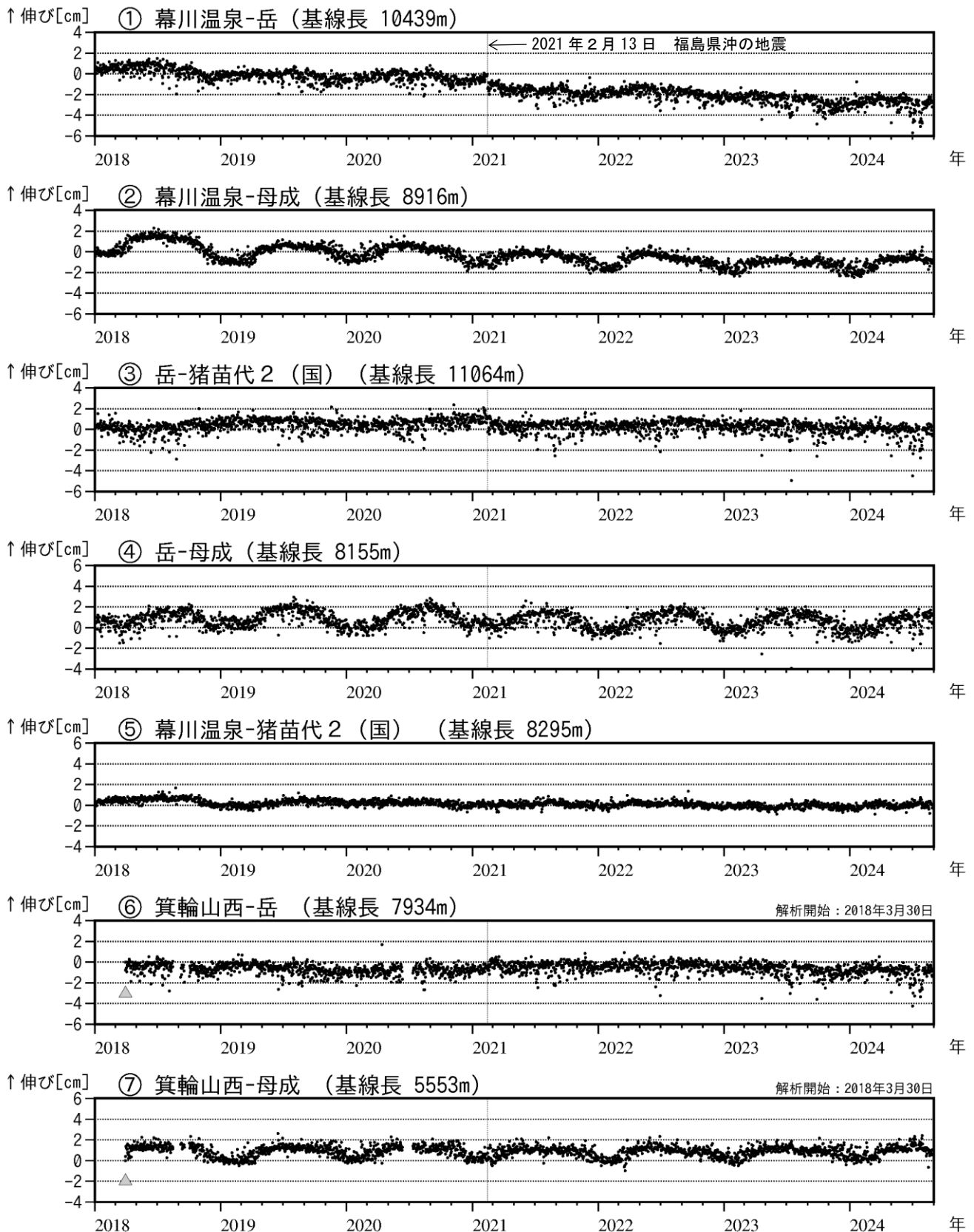
図4 安達太良山 GNSS 基線長変化図（2018年1月～2024年8月）
