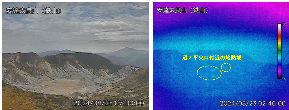
図2 安達太良山 沼ノ平火口周辺の状況（8月25日）と地表面温度分布の状況（8月23日）
