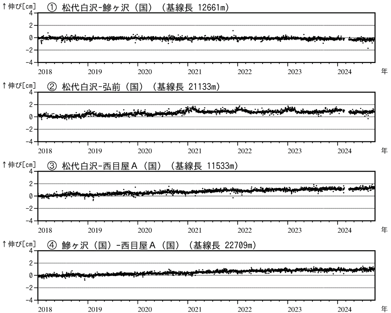
図3 岩木山 GNSS 基線長変化図（2018年1月～2024年9月）
