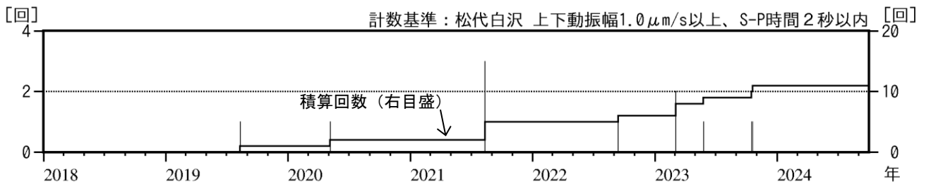
図2 岩木山 日別地震回数（2018年1月～2024年9月）
