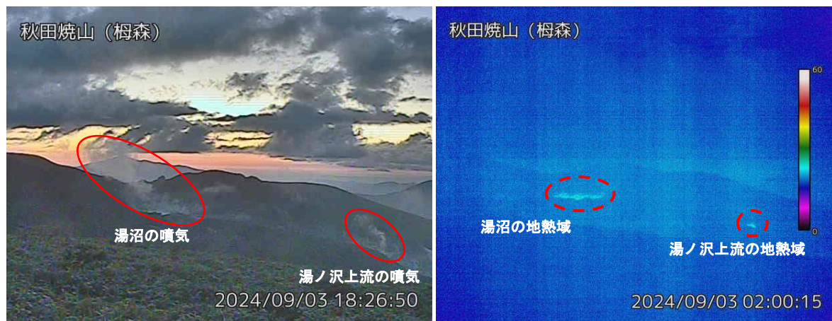
図2 秋田焼山 湯沼と湯ノ沢上流の様相と地表面温度分布（9月3日） ・柵森監視カメラ（湯沼の東約1km）の映像です。
