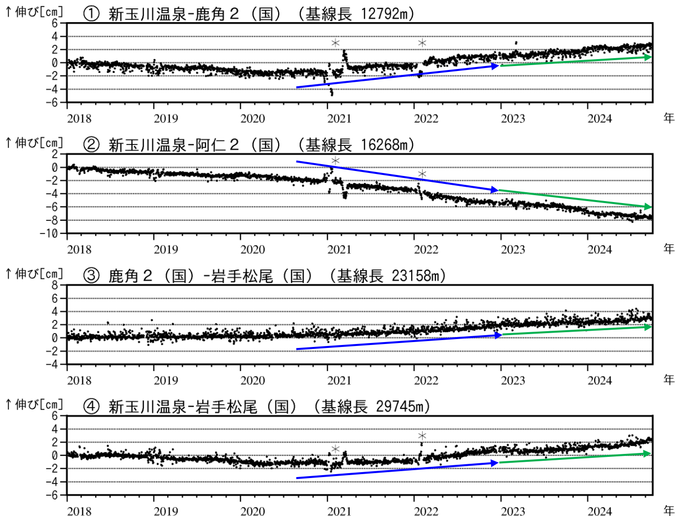
図4 秋田焼山 GNSS 基線長変化図（2018年1月～2024年9月）
