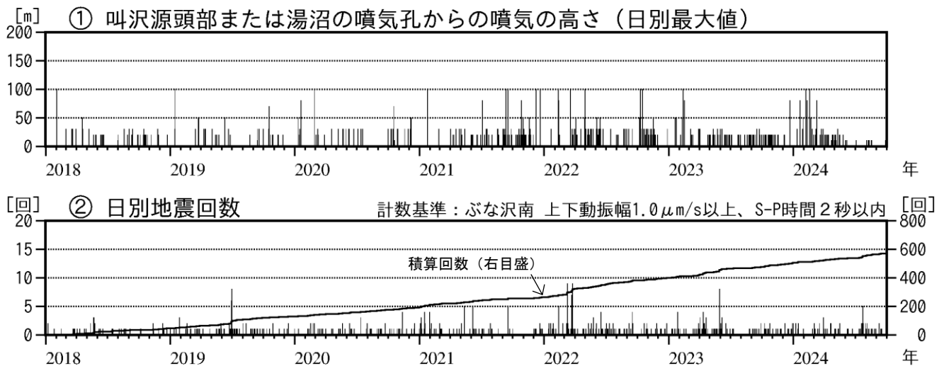
図3 秋田焼山 火山活動経過図（2018年1月～2024年9月）
