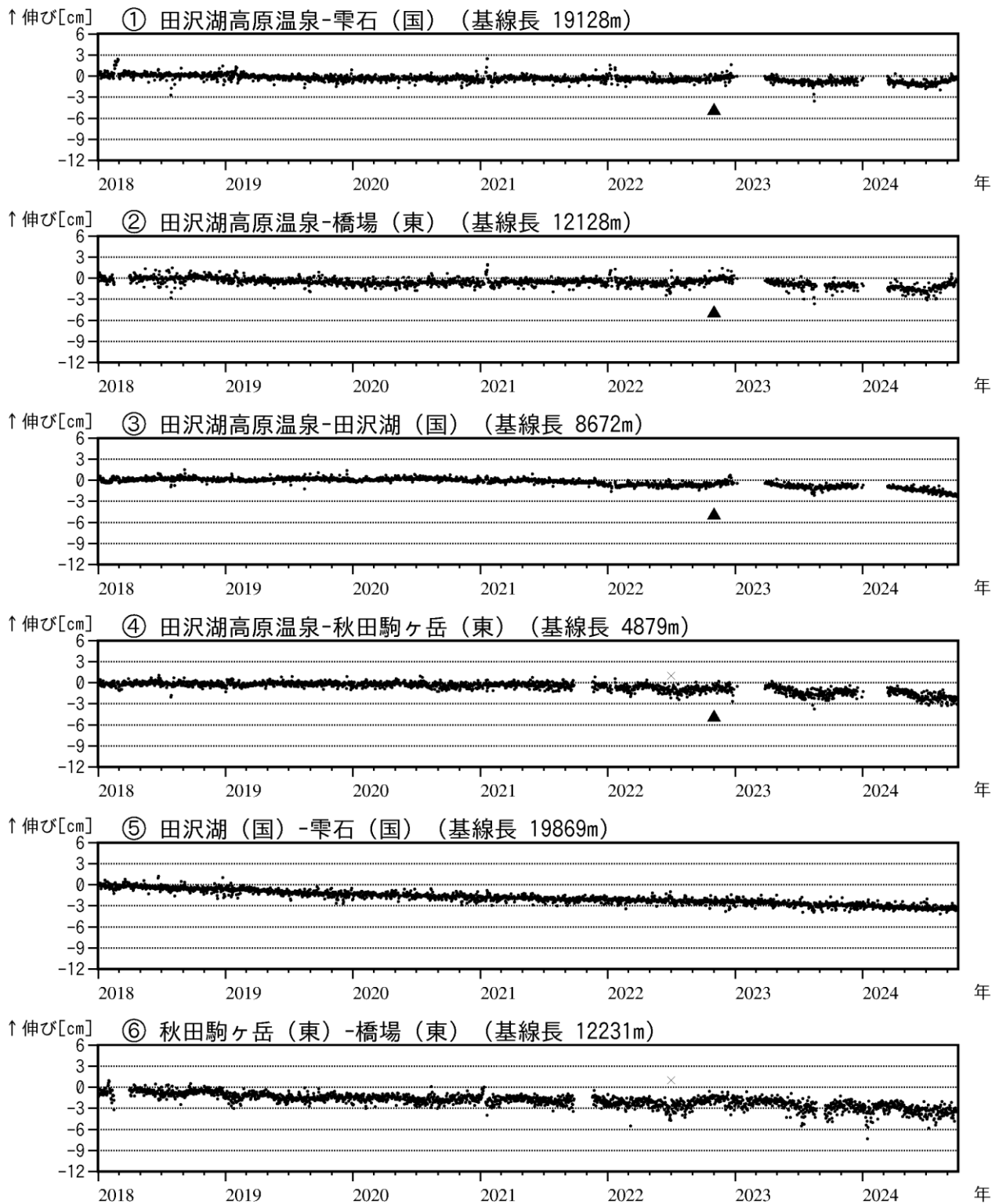
図5 秋田駒ヶ岳 GNSS 基線長変化図（2018年1月～2024年9月）
