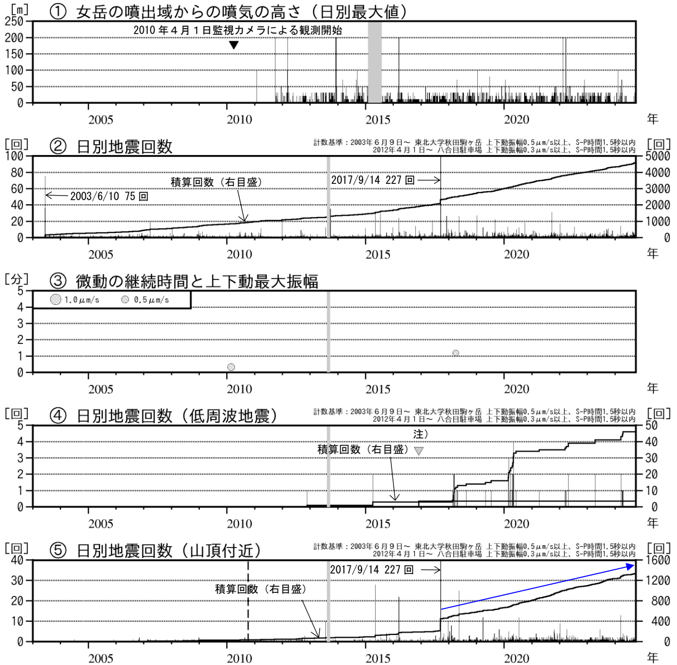
図2 秋田駒ヶ岳 火山活動経過図（2003年6月～2024年9月）
