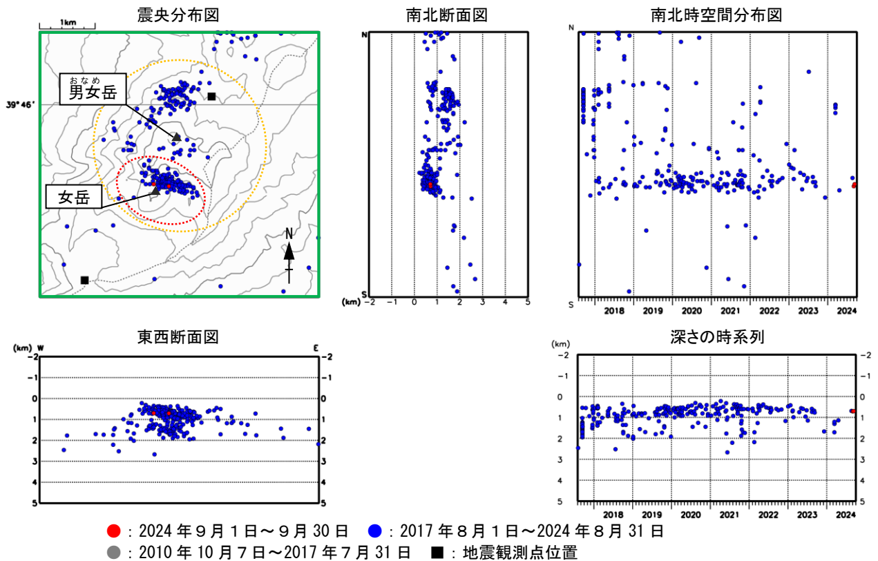
図4 秋田駒ヶ岳 地震活動（2010年10月7日～2024年9月）
