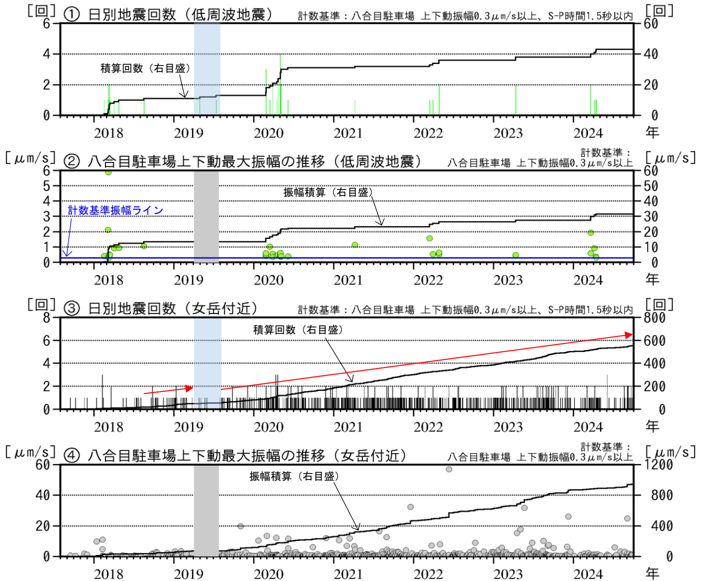
図3 秋田駒ヶ岳 低周波地震及び女岳付近の日別回数と最大振幅（2017年8月～2024年9月）
