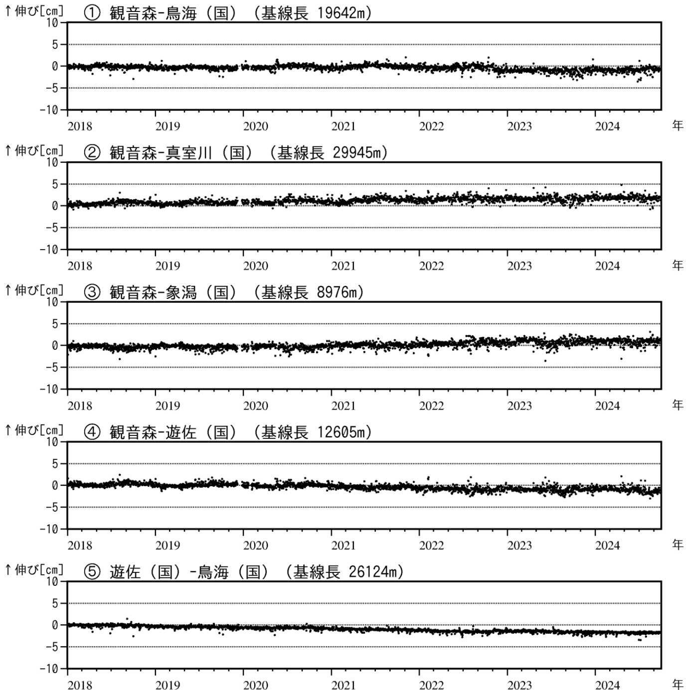
図4 鳥海山 GNSS 基線長変化図（2018年1月～2024年9月）
