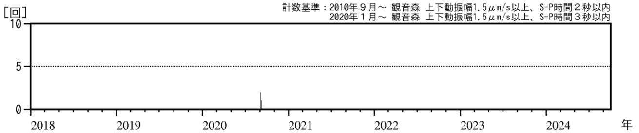
図3 鳥海山 火山性地震の日別回数（2018年1月～2024年9月）
