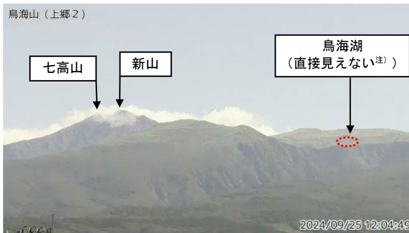
図1 鳥海山 山頂周辺の状況（9月25日）
