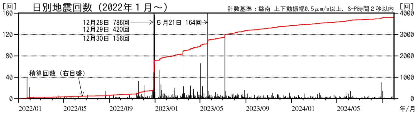
図4 磐梯山 地震回数（2022年1月～2024年9月）
