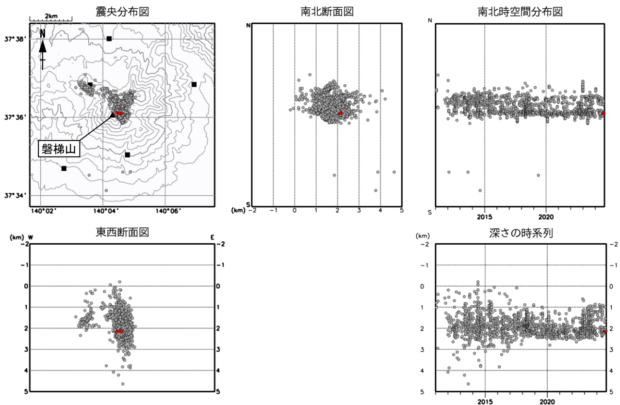
図5 磐梯山 震源分布図（2011年1月～2024年9月）
