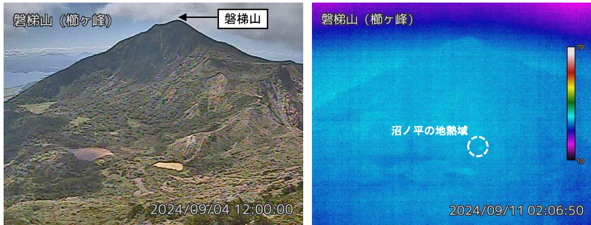
図2 磐梯山 沼ノ平周辺の状況（9月4日）と地表面温度分布（9月11日）
