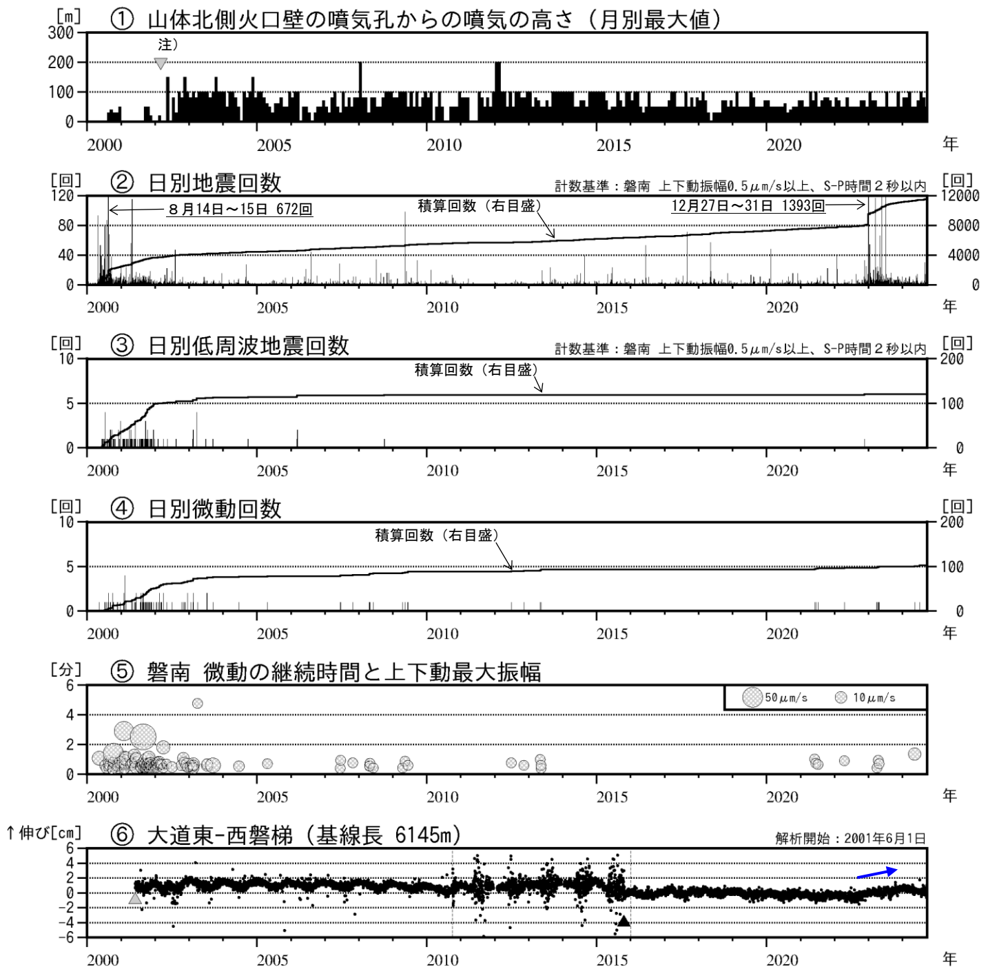
図3 磐梯山 火山活動経過図（2000年1月～2024年9月）
