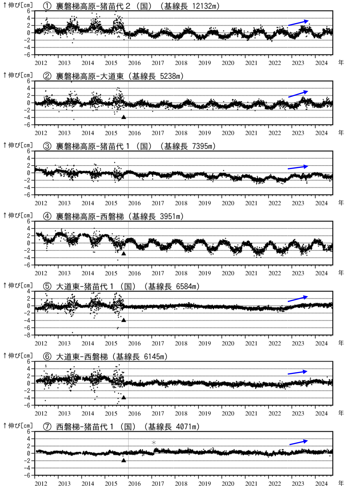
図6 磐梯山 GNSS 基線長変化図 (2012年1月～2024年9月)
