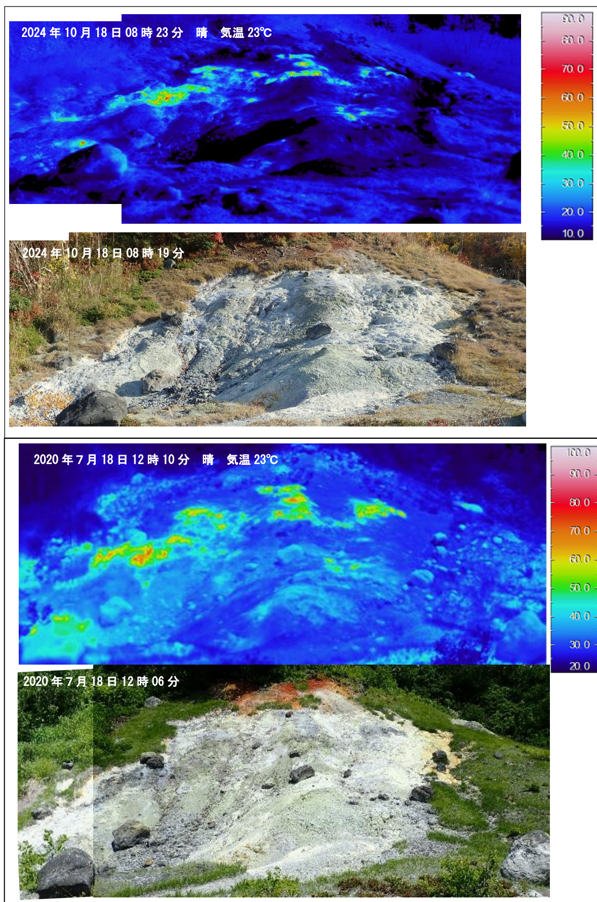
図3 八甲田山 南西方向から撮影した地獄沼北西の地熱域の状況と地表面温度分布 ・前回（2020年7月）と比較して、地熱域の分布に特段の変化は認められませんでした。 ※地熱域以外で温度の高い部分は、岩等が日射により温められたことによるものです。
