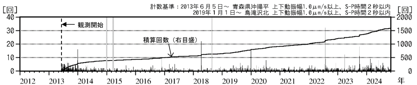
図7 八甲田山 日別地震回数（2013年6月～2024年10月）
