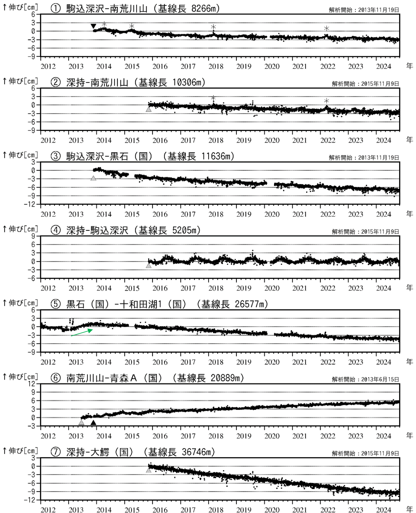
図8 八甲田山 GNSS 基線長変化図（2012年1月～2024年10月）
