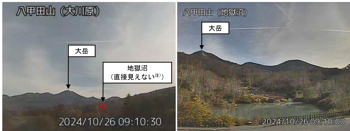
図6 八甲田山 山頂部及び地獄沼周辺の状況（10月26日）
