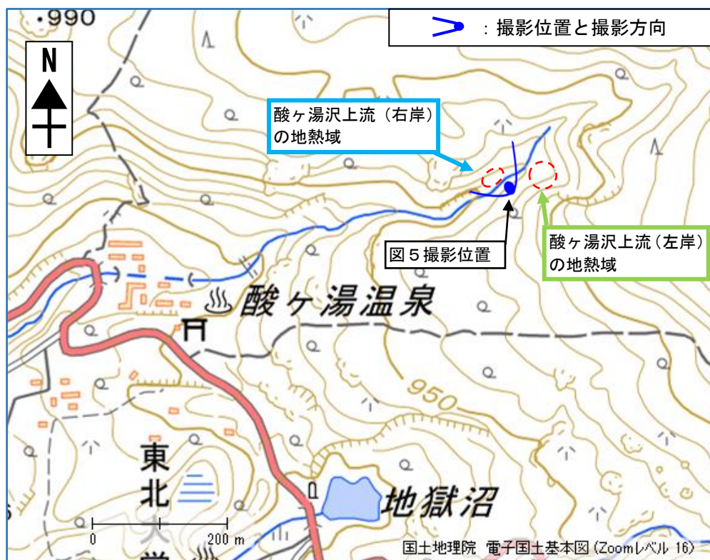
図4 八甲田山 酸ヶ湯沢上流の写真と地表面温度分布撮影位置及び撮影方向
