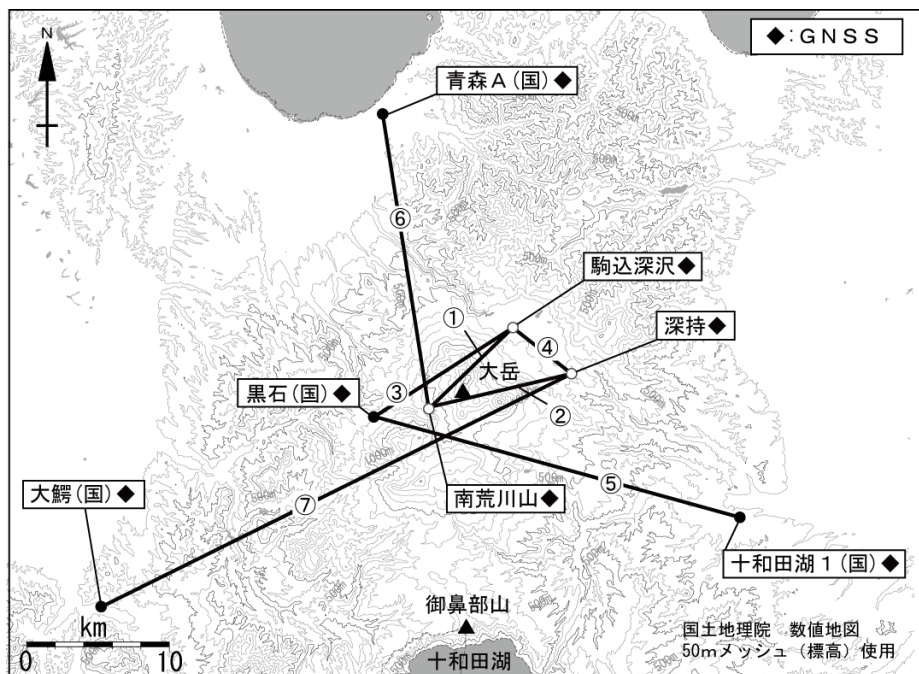
図10 八甲田山 GNSS 観測基線図
