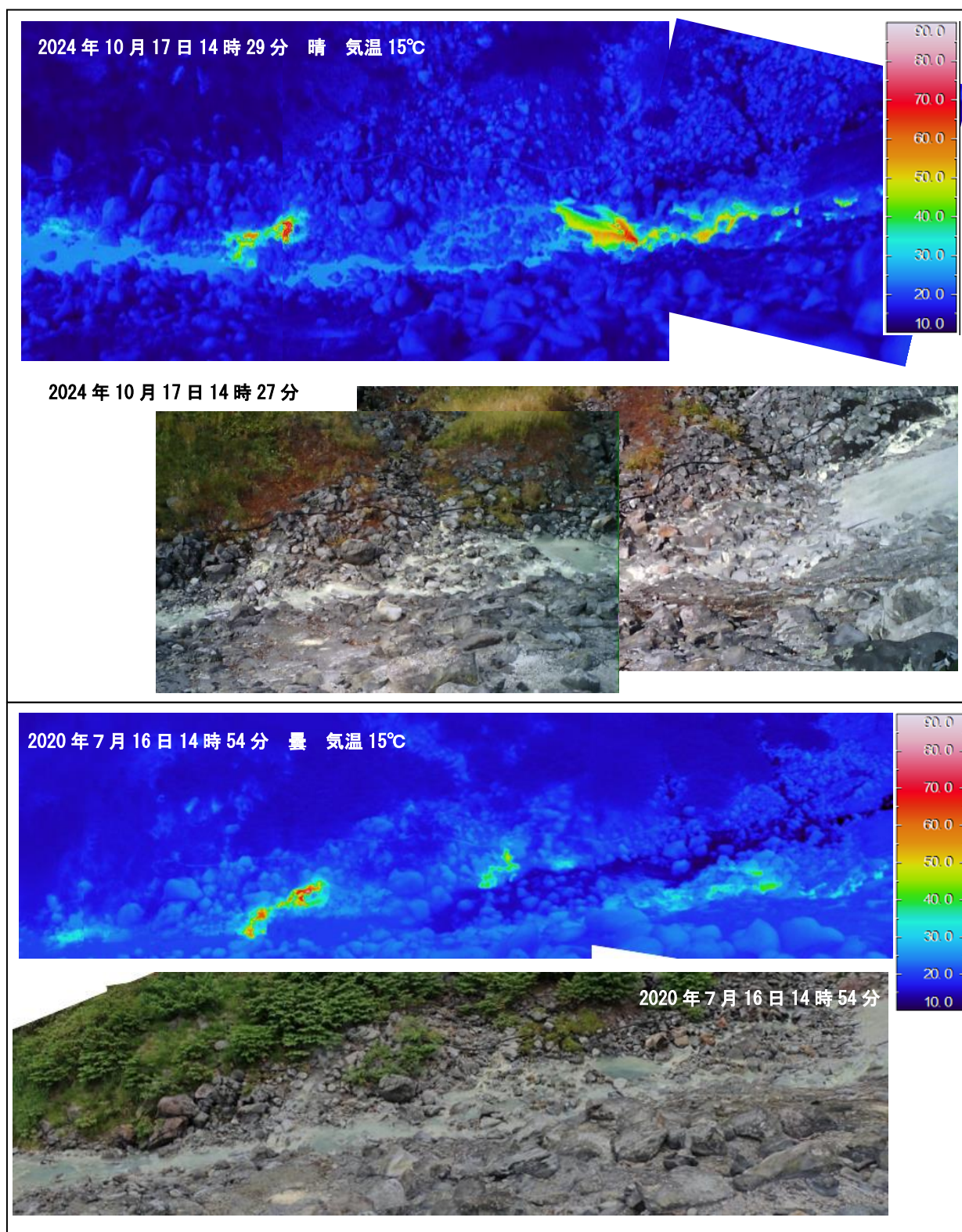
図5 八甲田山 南東方向から撮影した酸ヶ湯沢上流（右岸）の状況と地表面温度分布
