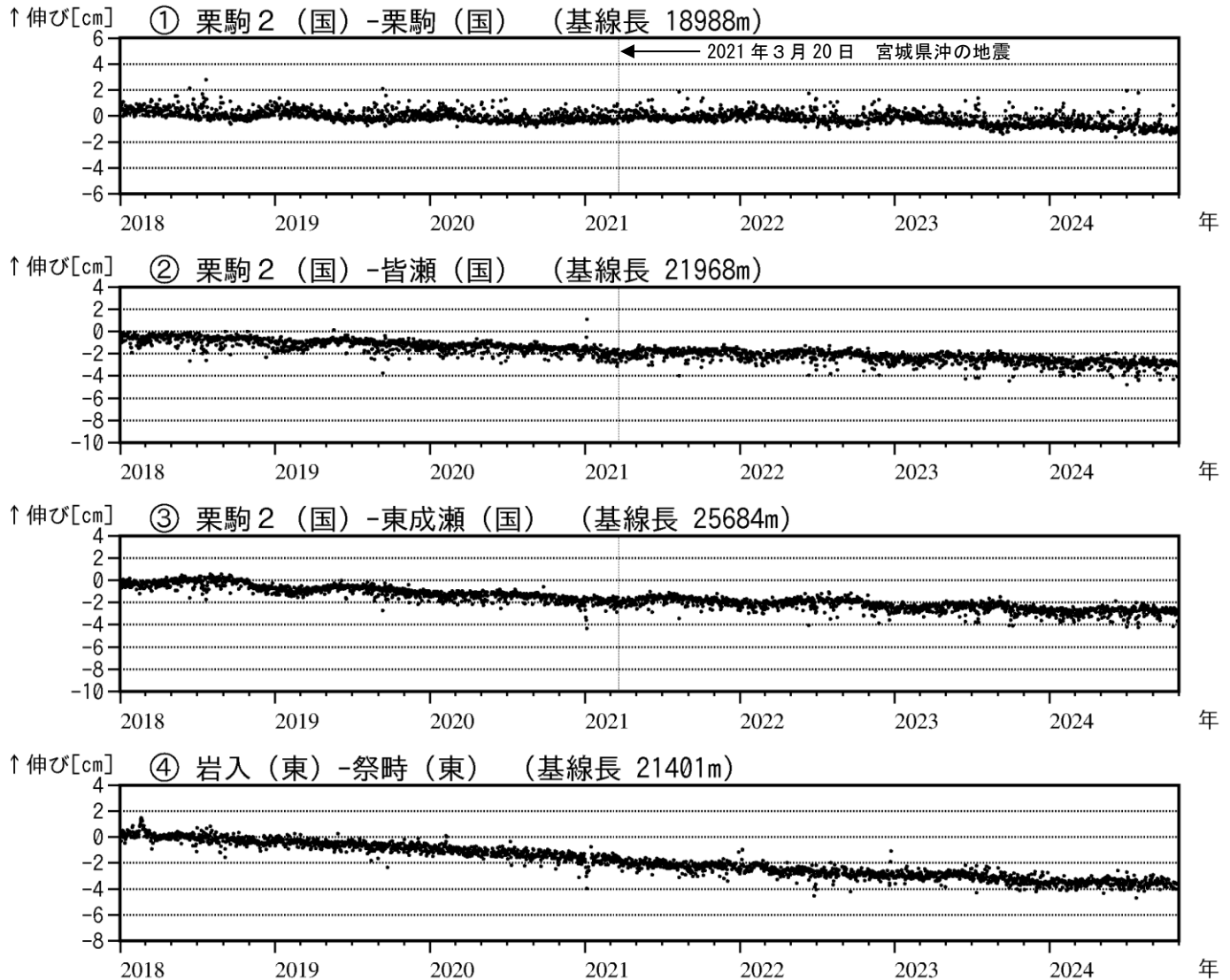
図4 栗駒山 GNSS 基線長変化図（2018年1月～2024年10月）
