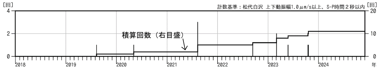
図2 岩木山 日別地震回数（2018年1月～2024年11月）
