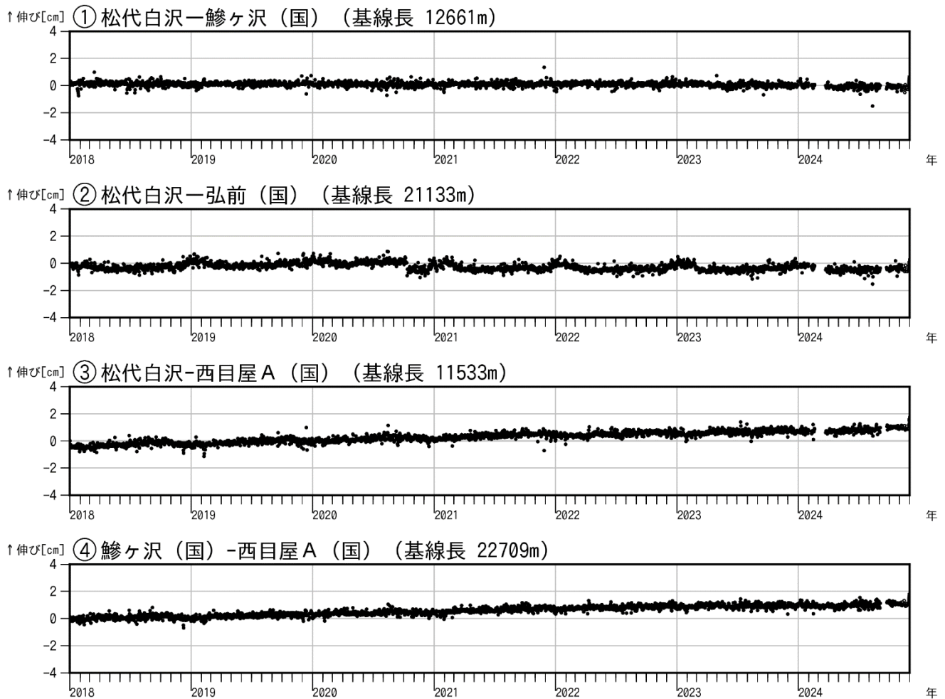
図3 岩木山 GNSS 基線長変化図（2018年1月～2024年11月）
