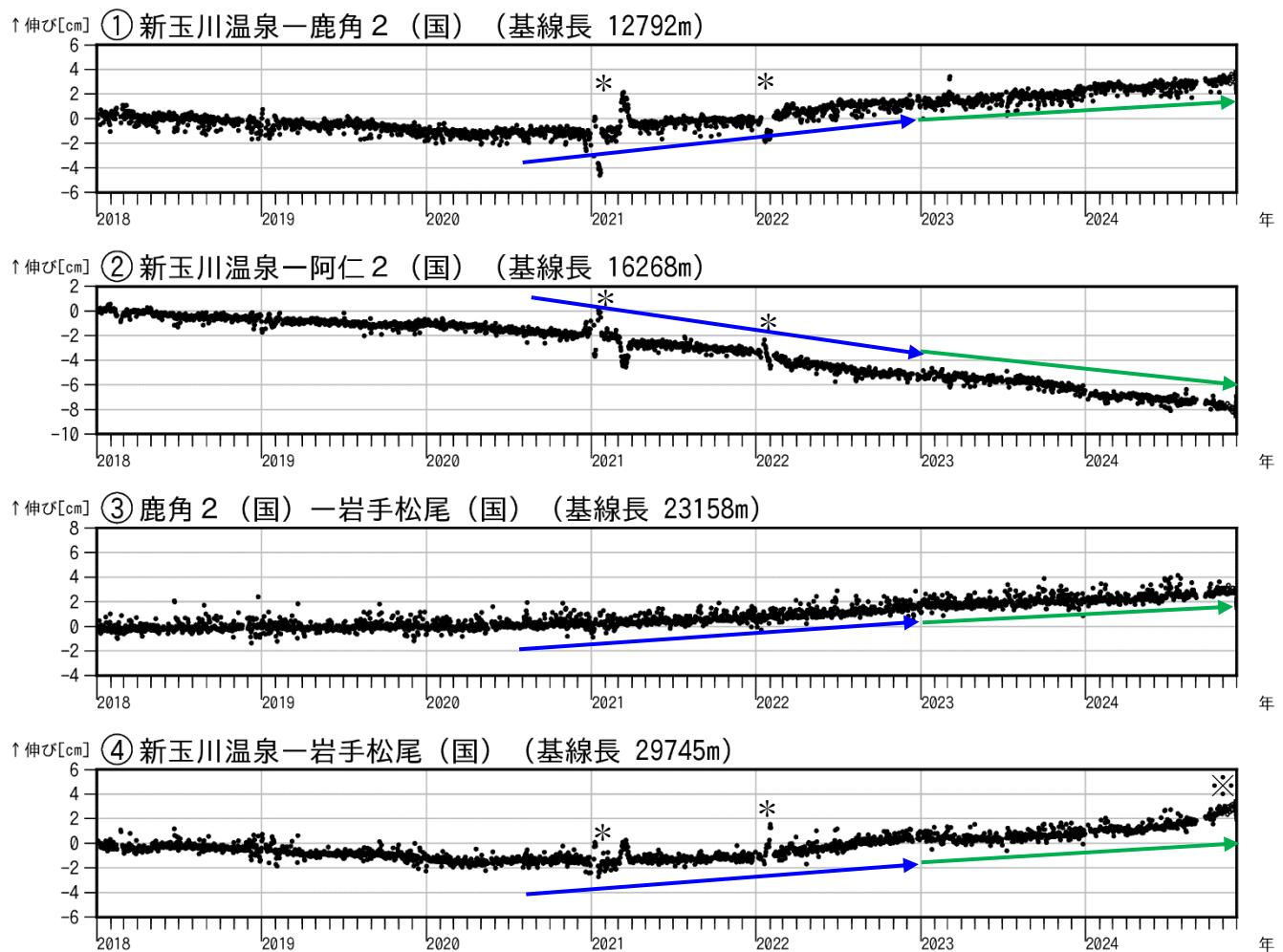
図4 秋田焼山 GNSS 基線長変化図（2018年1月～2024年11月）
