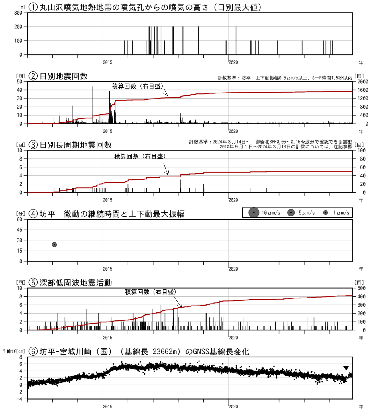
図2 蔵王山 火山活動経過図（2012年1月～2024年11月）
