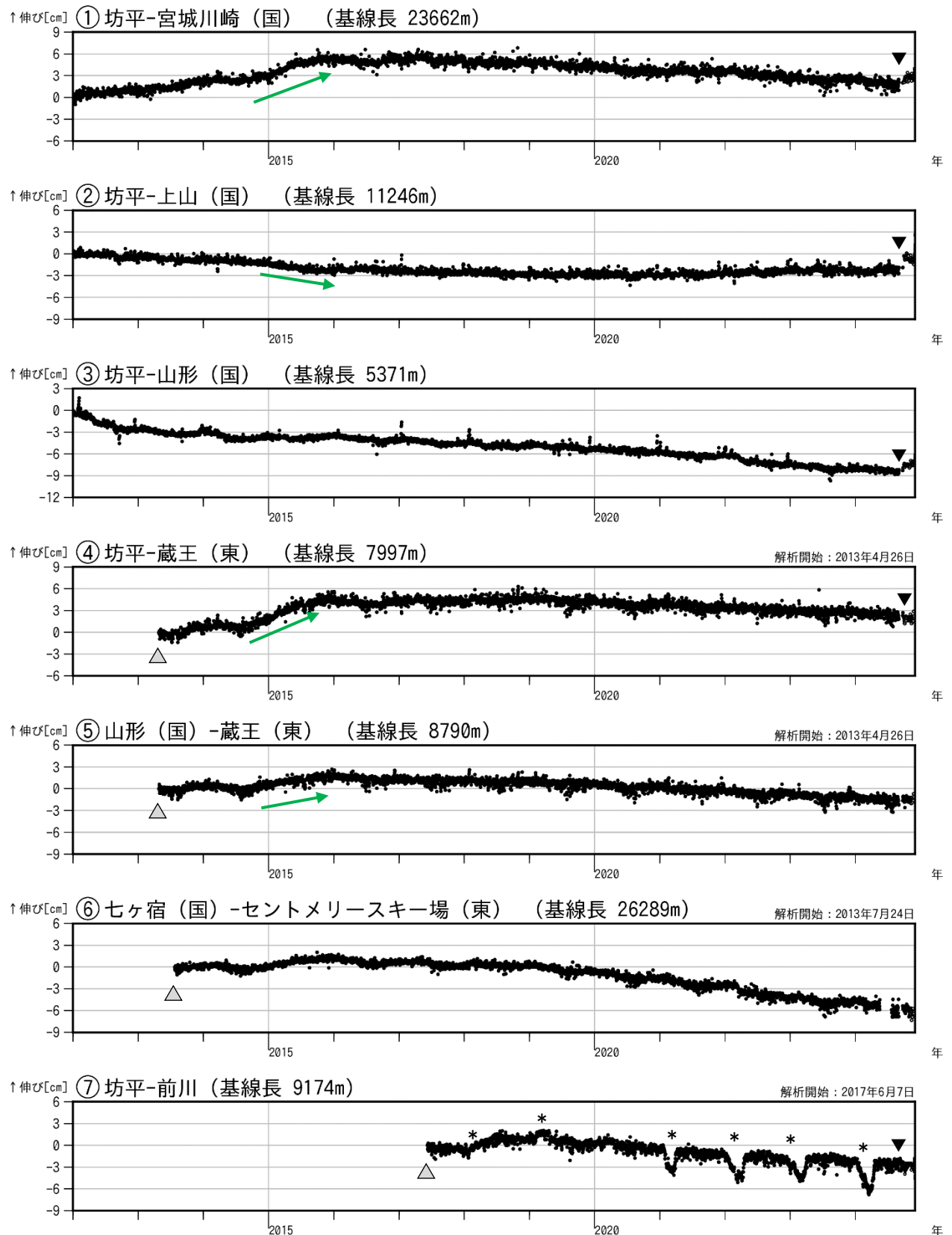
図3 蔵王山 GNSS 基線長変化図（2012年1月～2024年11月）
