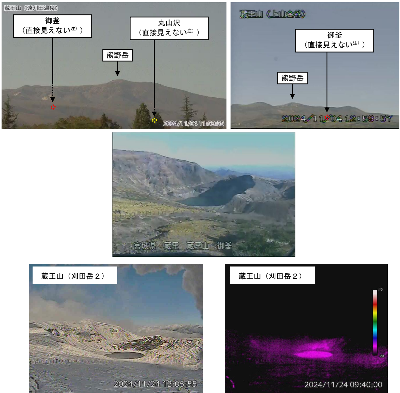
図1 蔵王山 山頂部の状況
