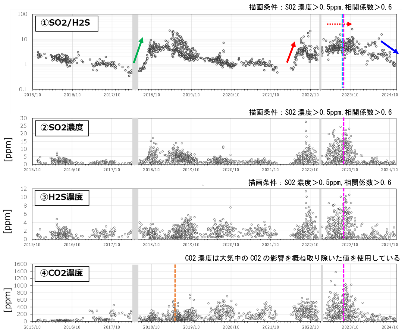
図6 吾妻山 火山ガス観測装置による観測（2015年11月～2024年11月）
