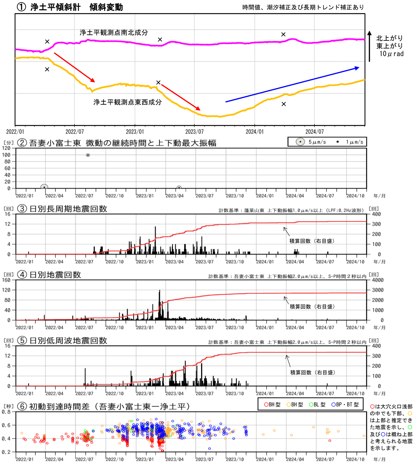
図3 吾妻山 火山活動経過図（2022年1月～2024年11月）
