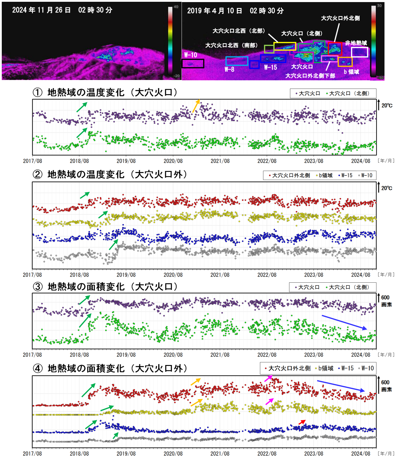
図5 吾妻山 監視カメラによる大穴火口周辺の地熱域の経過（2017年8月～2024年11月）
