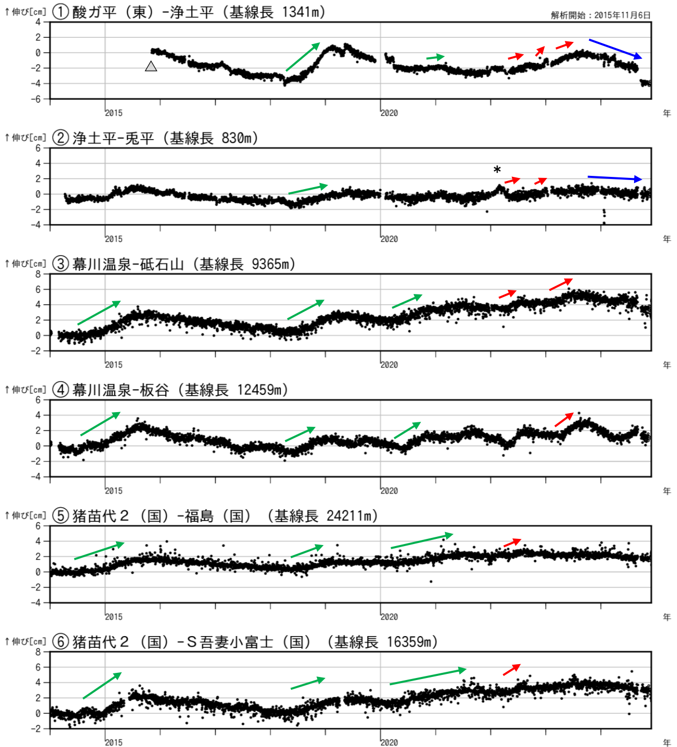
図4 吾妻山 吾妻山浅部・深部の地殻変動 (2014年1月～2024年11月)
