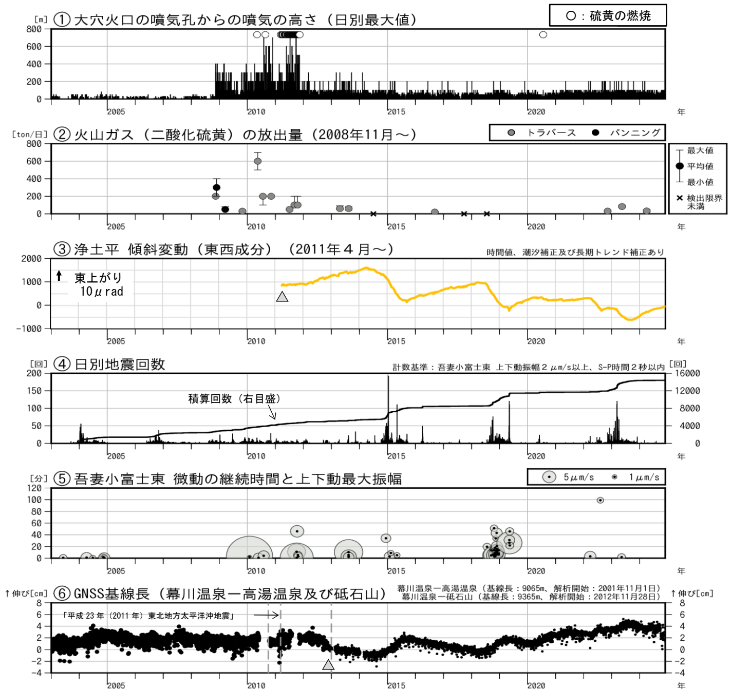
図2 吾妻山 中期的な火山活動の経過（2003年1月～2024年11月）
