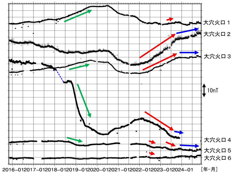
図7 吾妻山 全磁力連続観測点の全磁力値変化（2015年11月～2024年11月）
