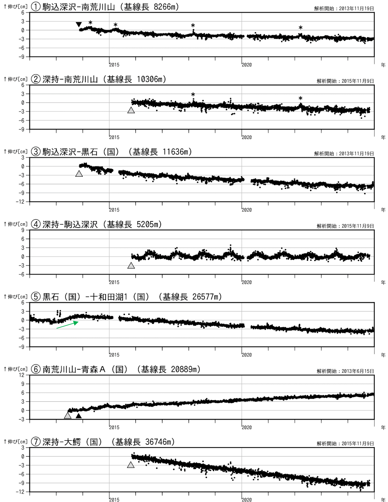
図3 八甲田山 GNSS 基線長変化図（2012年1月～2024年12月）
