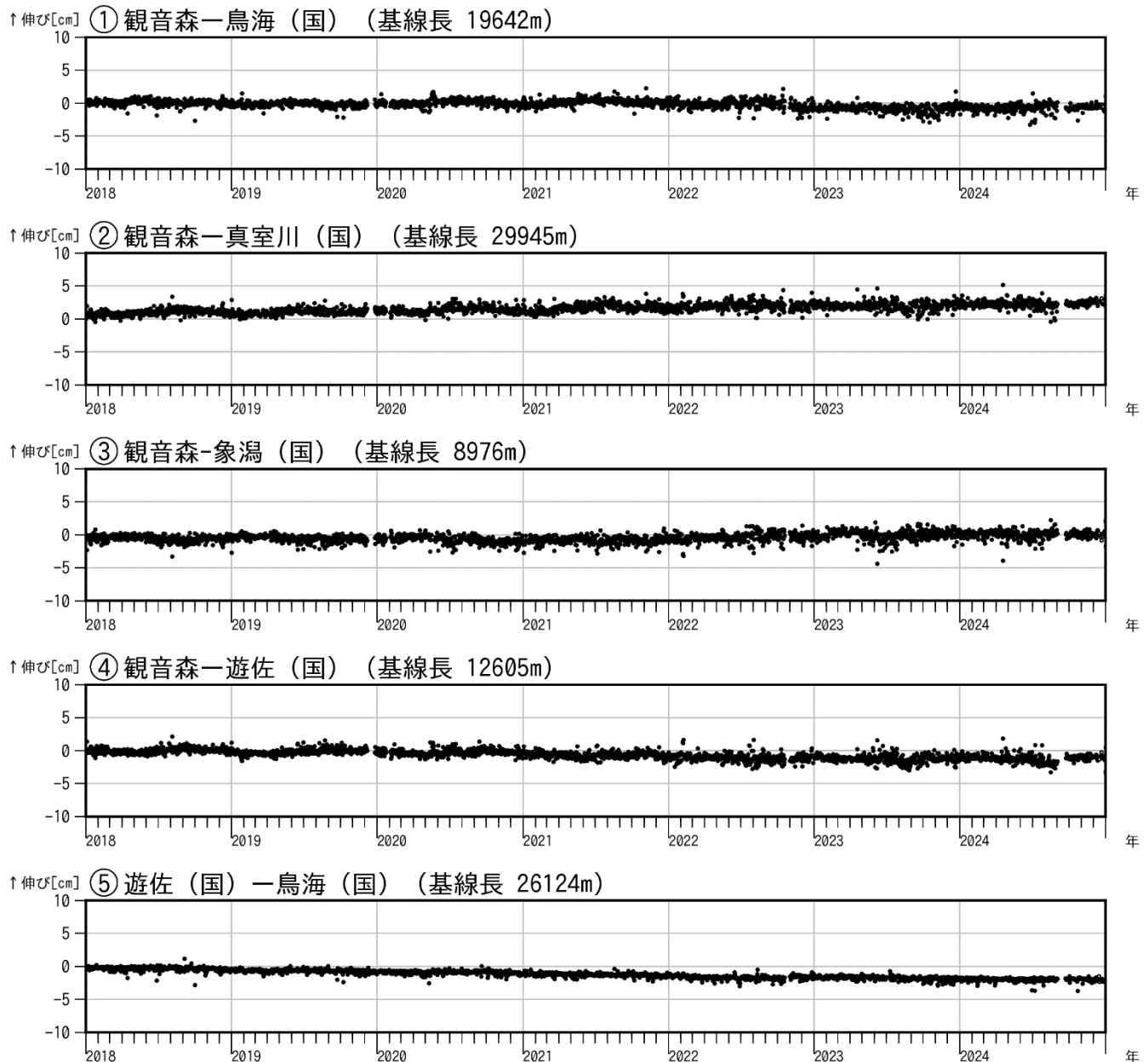
図4 鳥海山 GNSS 基線長変化図（2018年1月～2024年12月）
