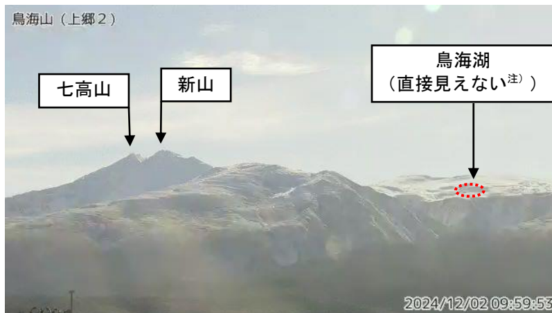
図1 鳥海山 山頂周辺の状況（12月2日）
