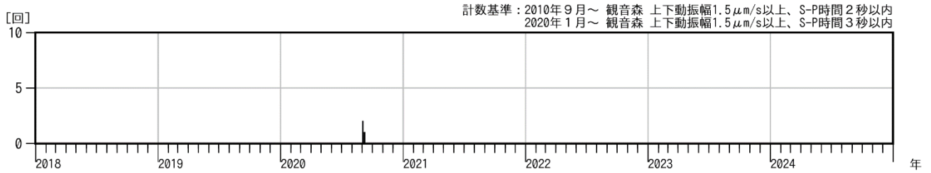
図3 鳥海山 火山性地震の日別回数（2018年1月～2024年12月）
