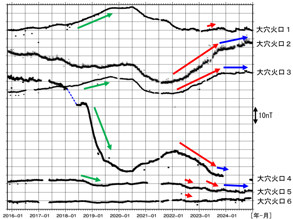
図7 吾妻山 全磁力連続観測点の全磁力値変化（2015年11月～2024年12月）
