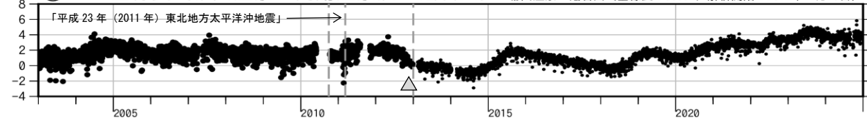
図2 吾妻山 中期的な火山活動の経過（2003年1月～2024年12月）
