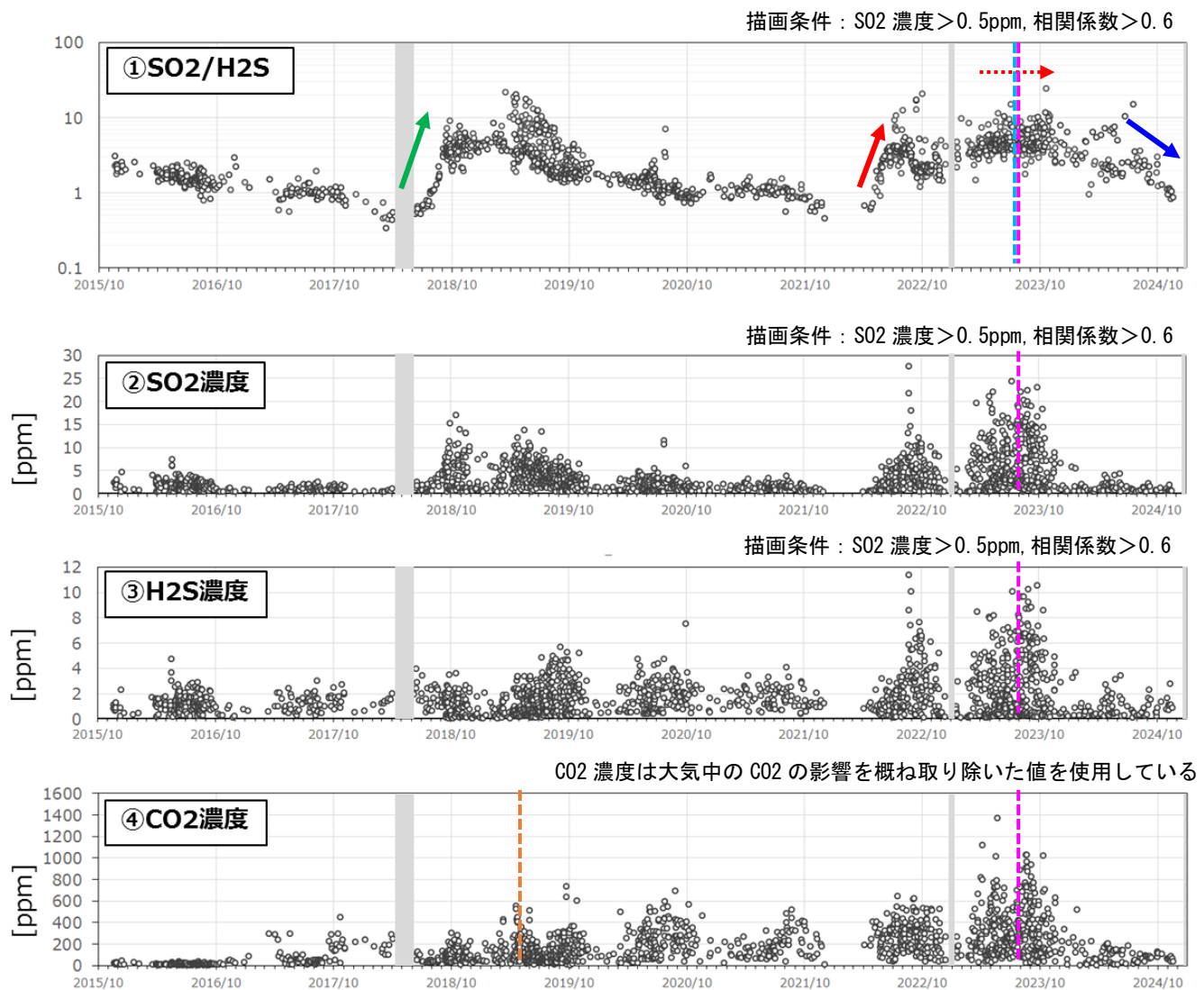
図6 吾妻山 火山ガス観測装置による観測（2015年11月～2024年12月）
