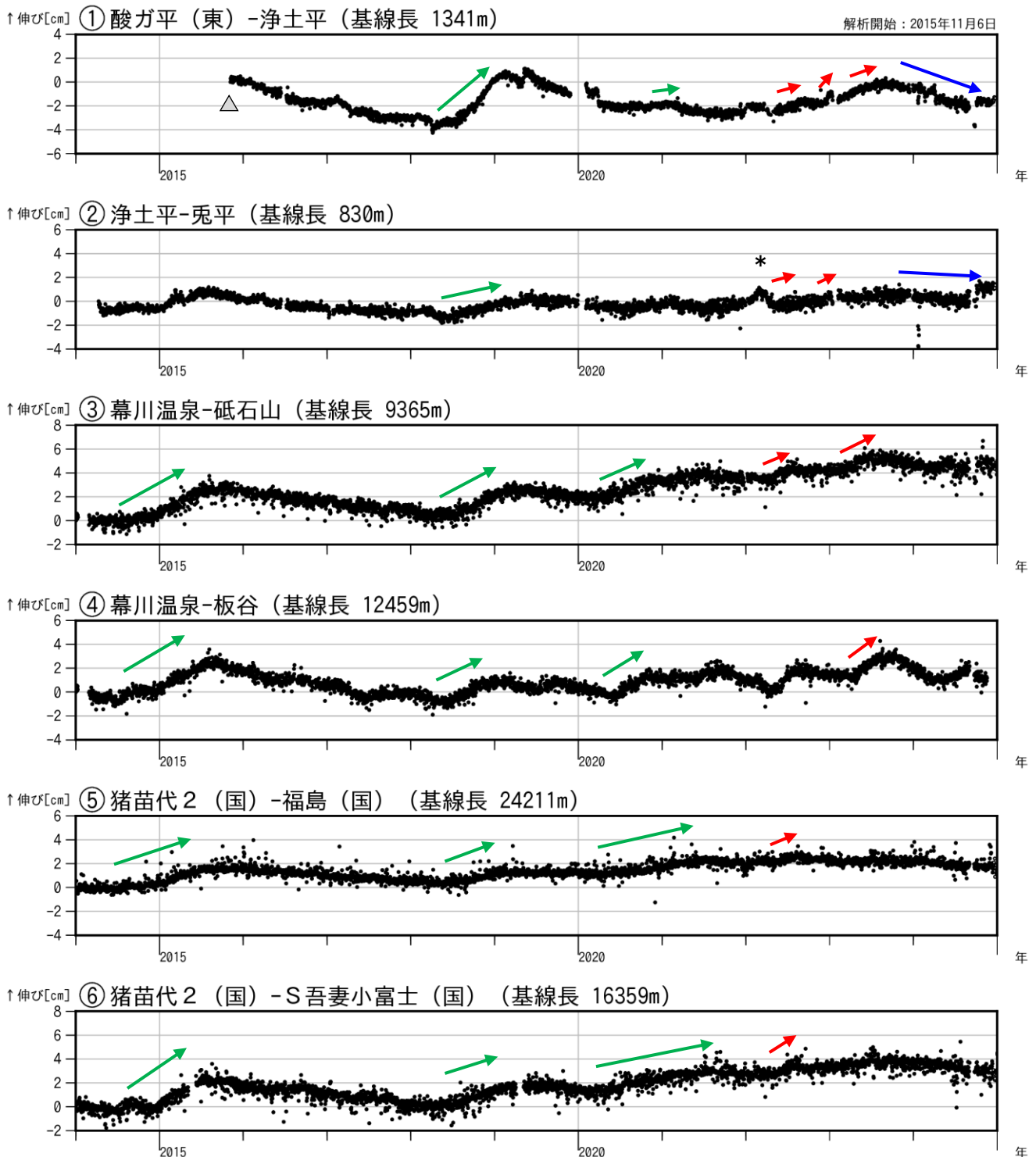
図4 吾妻山 吾妻山浅部・深部の地殻変動（2014年1月～2024年12月）
