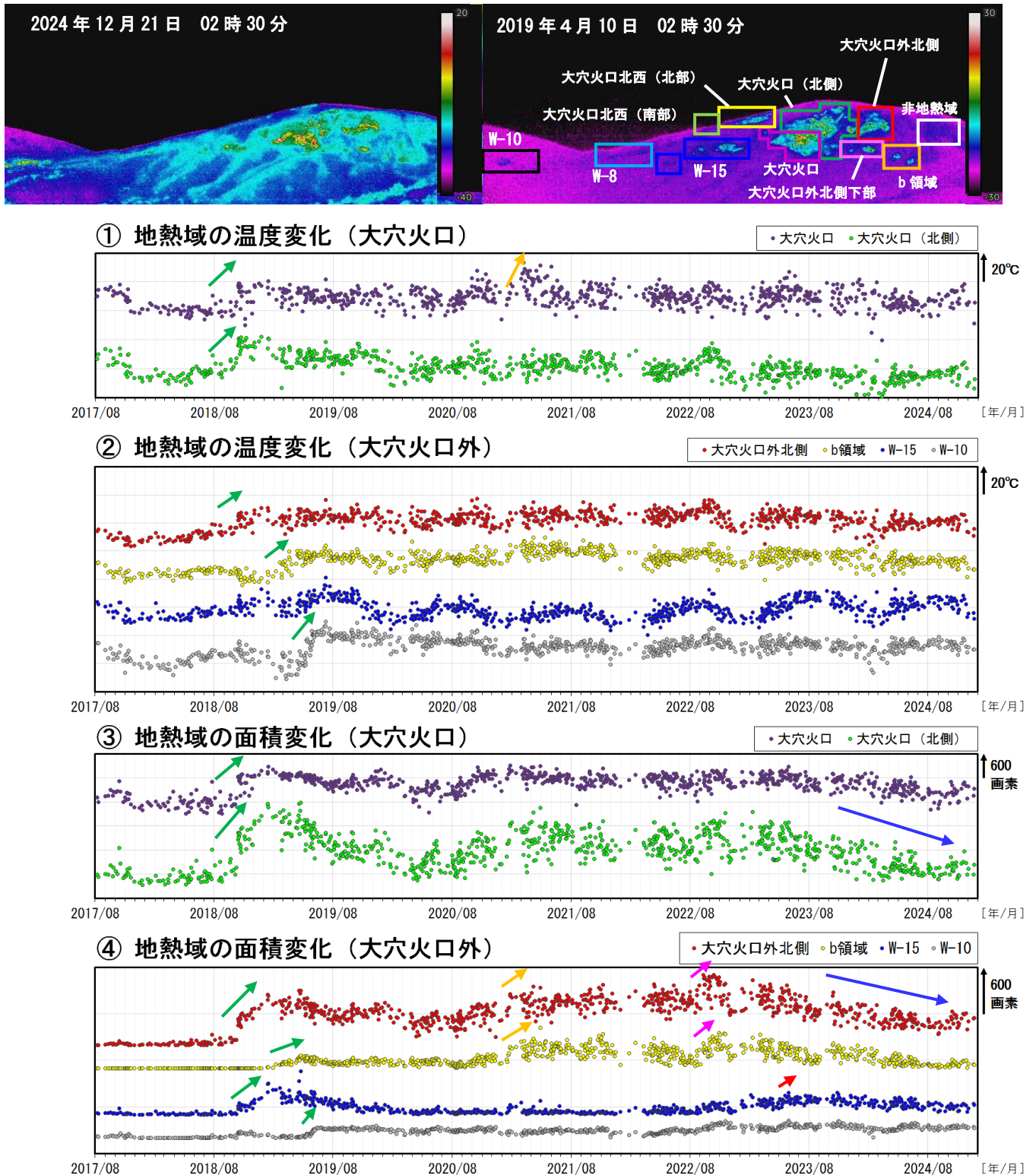
図5 吾妻山 監視カメラによる大穴火口周辺の地熱域の経過（2017年8月～2024年12月）
