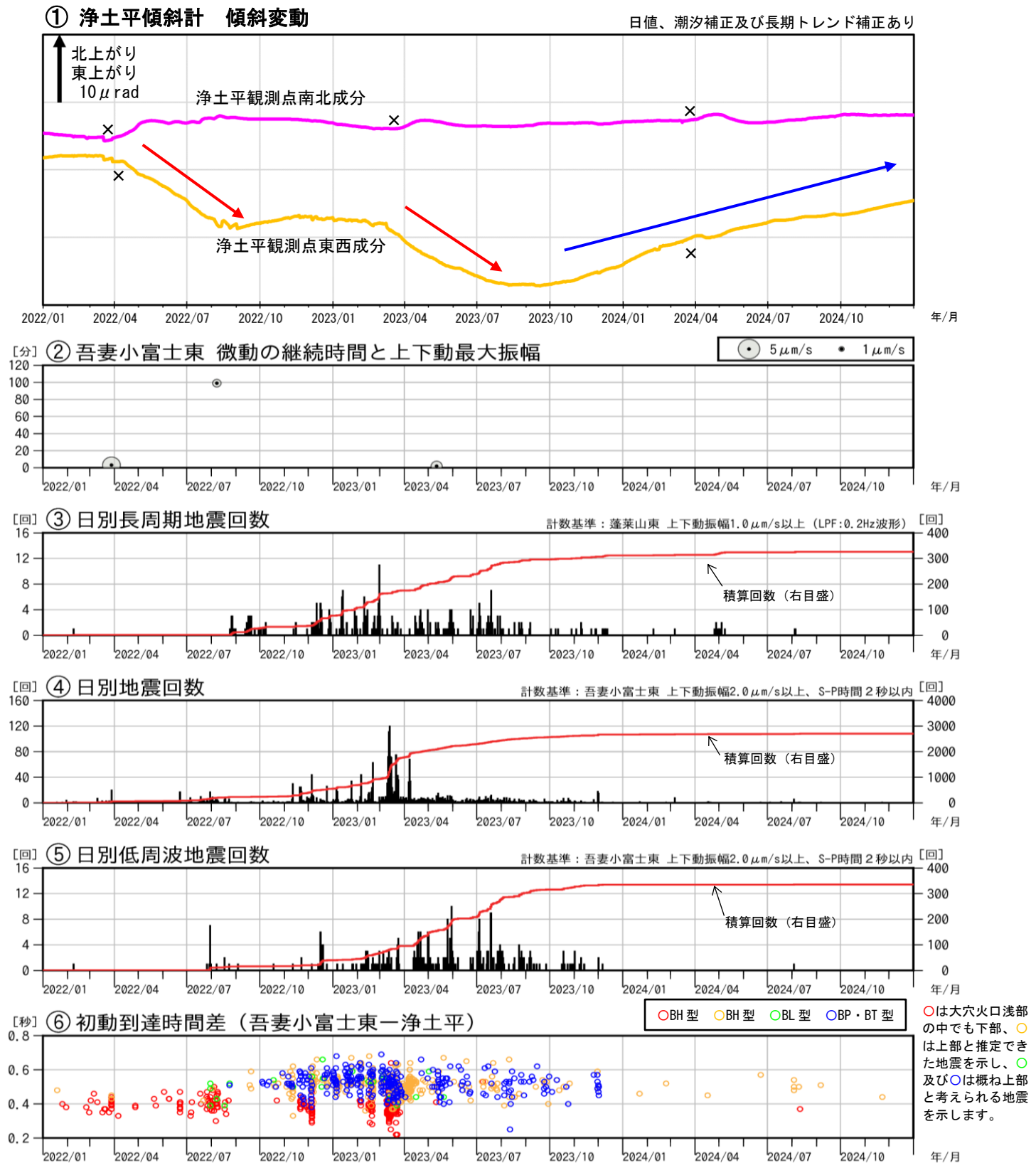
図3 吾妻山 火山活動経過図（2022年1月～2024年12月）
