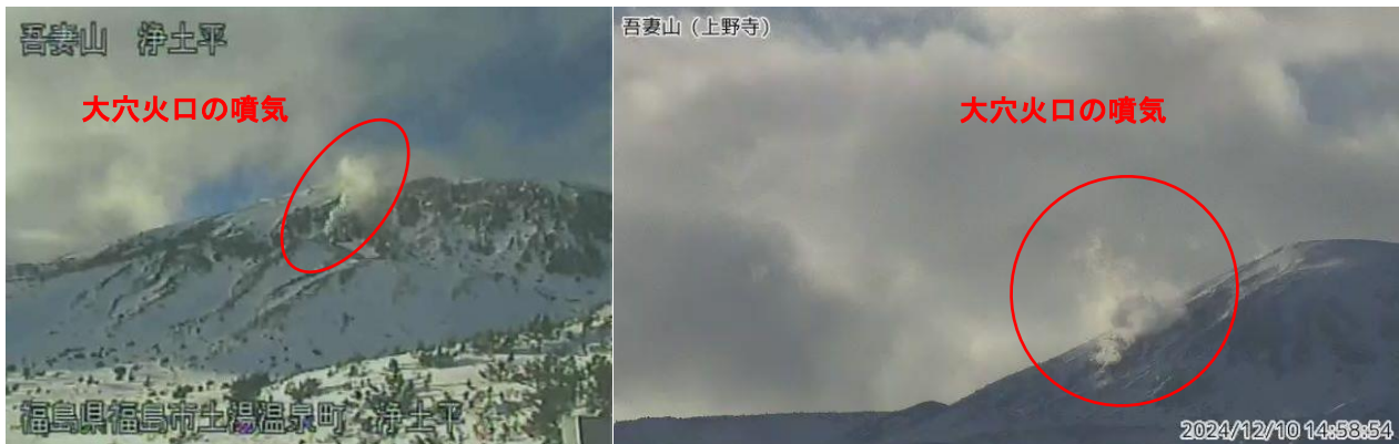
図1 吾妻山 大穴火口周辺の噴気の状態（12月10日）
