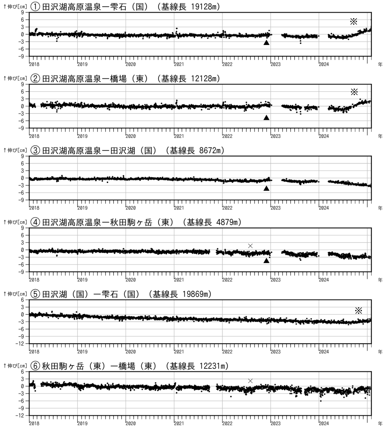
図5 秋田駒ヶ岳 GNSS 基線長変化図（2018年1月～2025年1月）
