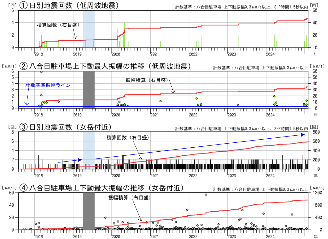
図3 秋田駒ヶ岳 低周波地震及び女岳付近の日別回数と最大振幅（2017年8月～2025年1月）
