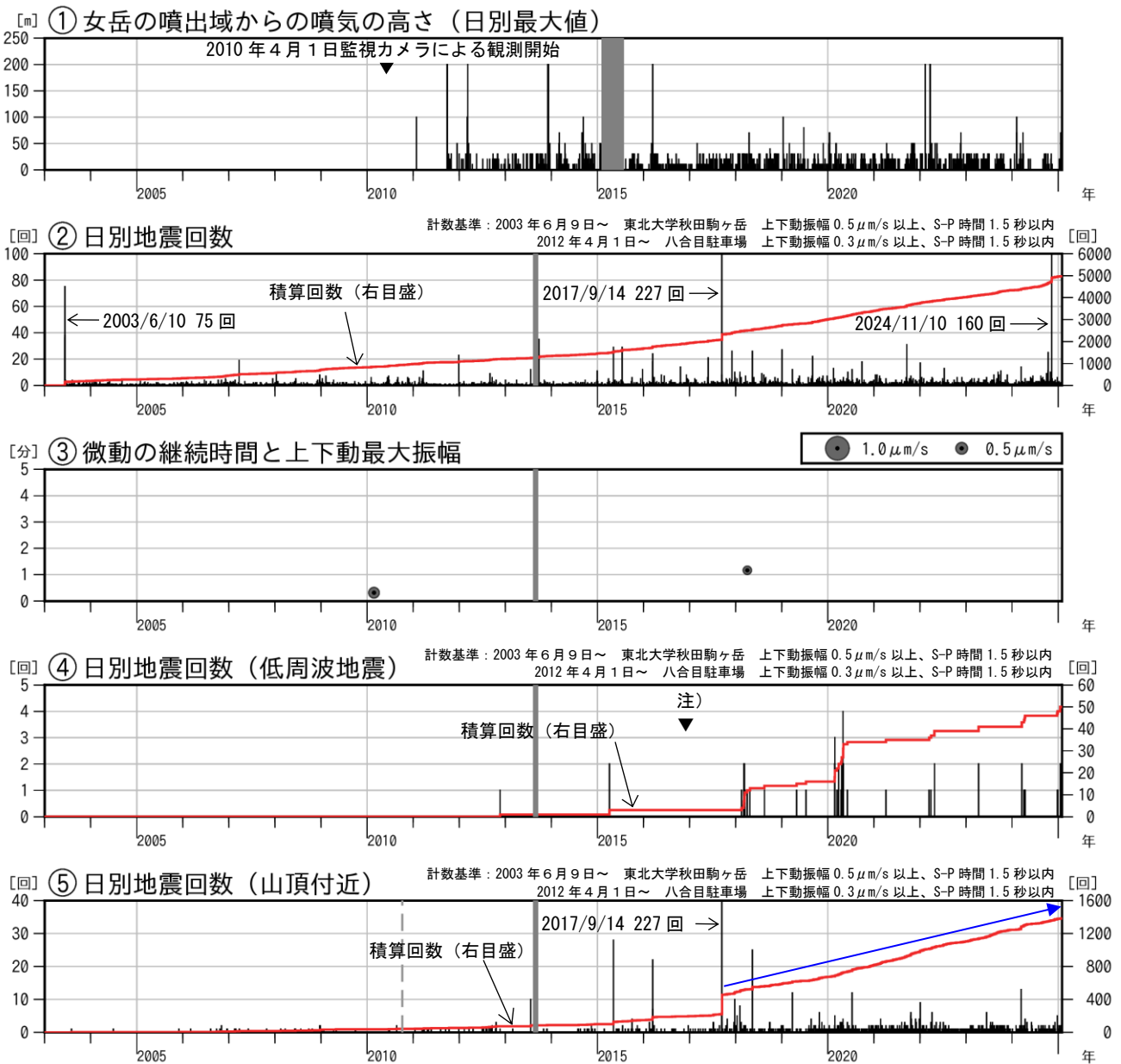
図 2 秋田駒ヶ岳 火山活動経過図（2003 年 6 月～2025 年 1 月）
