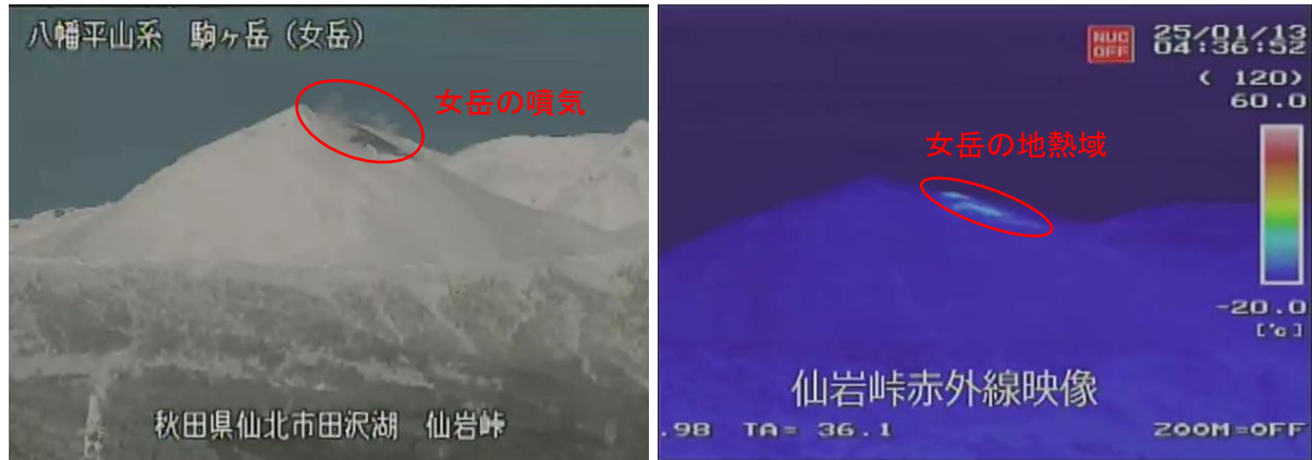
図1 秋田駒ヶ岳 女岳周辺の状況（1月19日）と地表面温度分布の状況（1月13日） ・東北地方整備局が設置している仙岩峠監視カメラ（女岳山頂の南約5km）の可視及び赤外映像です。
