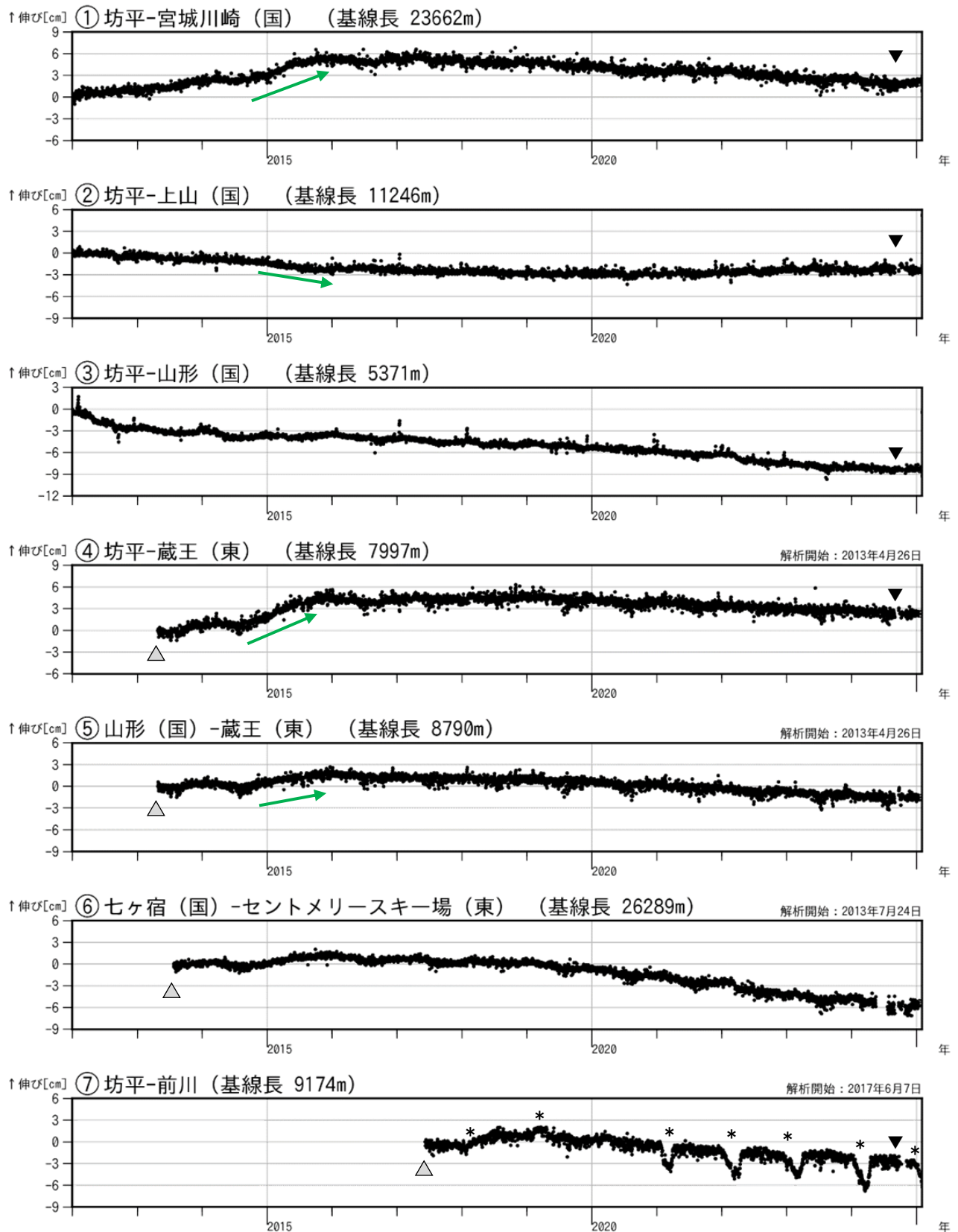
図3 蔵王山 GNSS 基線長変化図 (2012 年 1 月～2025 年 1 月)
