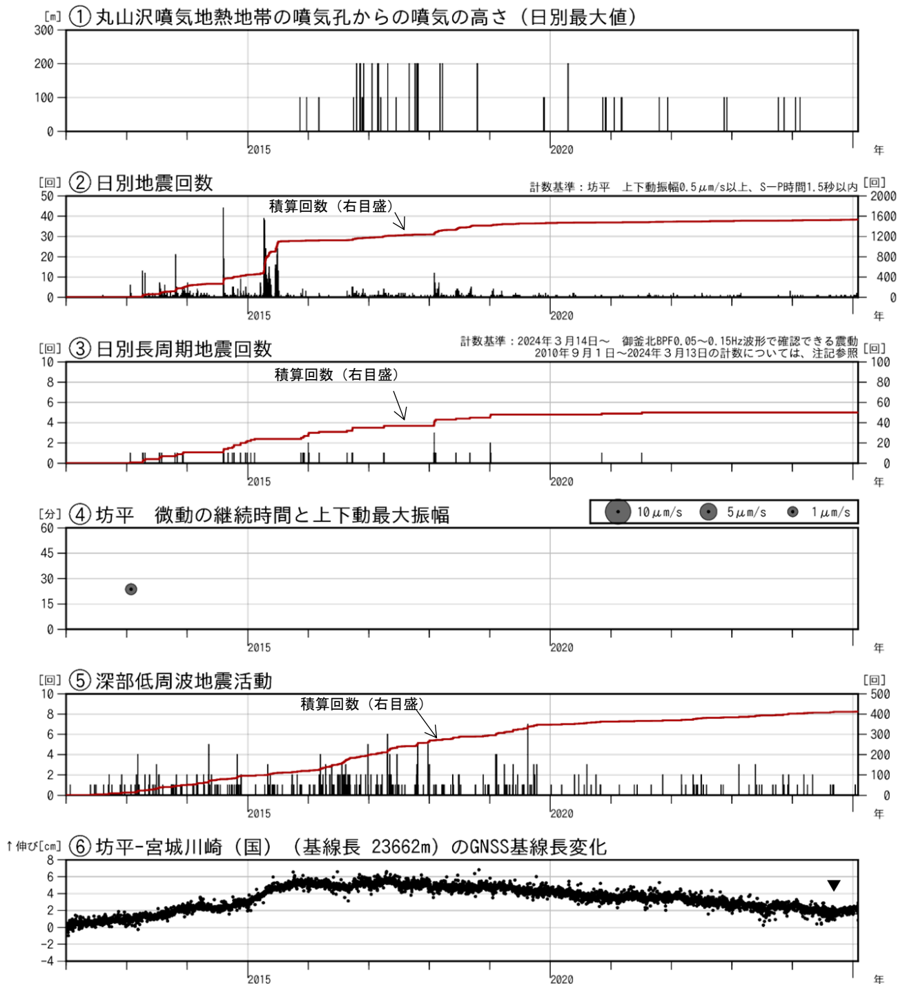
図2 蔵王山 火山活動経過図（2012年1月～2025年1月）
