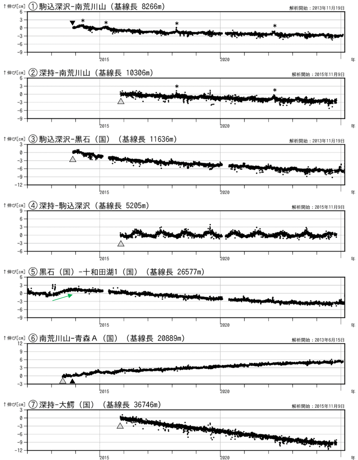
図3 八甲田山 GNSS 基線長変化図（2012年1月～2025年2月）
