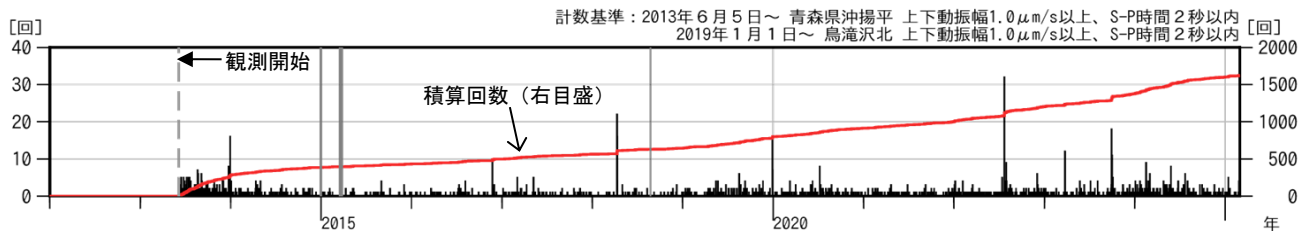
図 2 八甲田山 日別地震回数（2013 年 6 月～2025 年 2 月）
