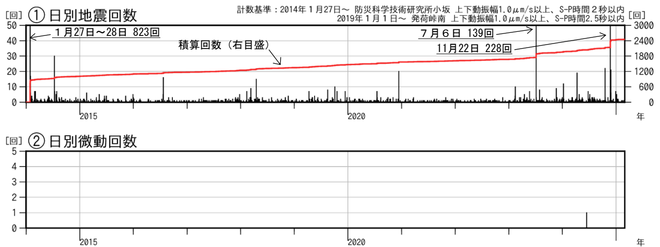
図2 十和田 活動経過図（2014年1月～2025年2月）
