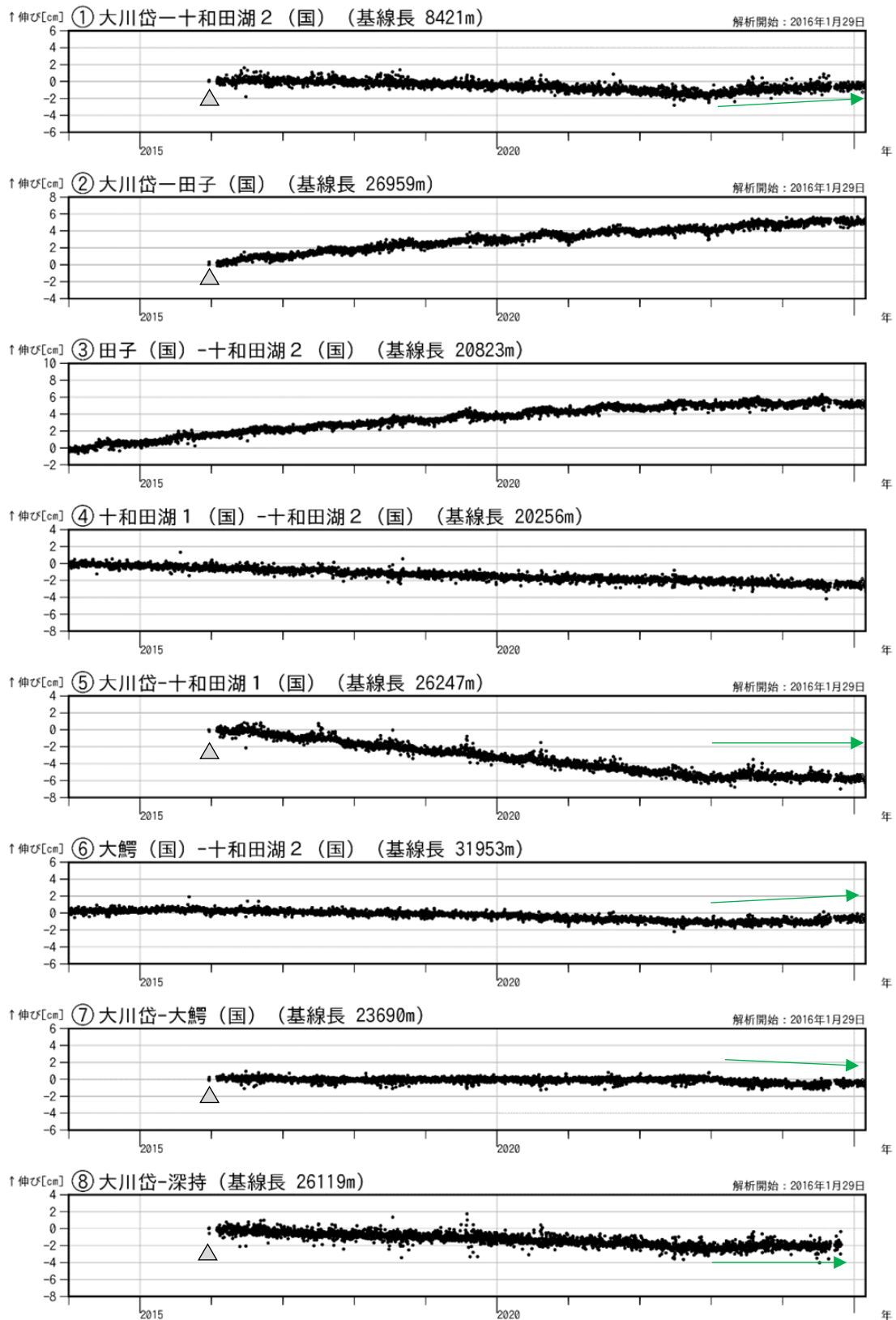
図3 十和田 GNSS 基線長変化図 (2014 年 1 月～2025 年 2 月)
