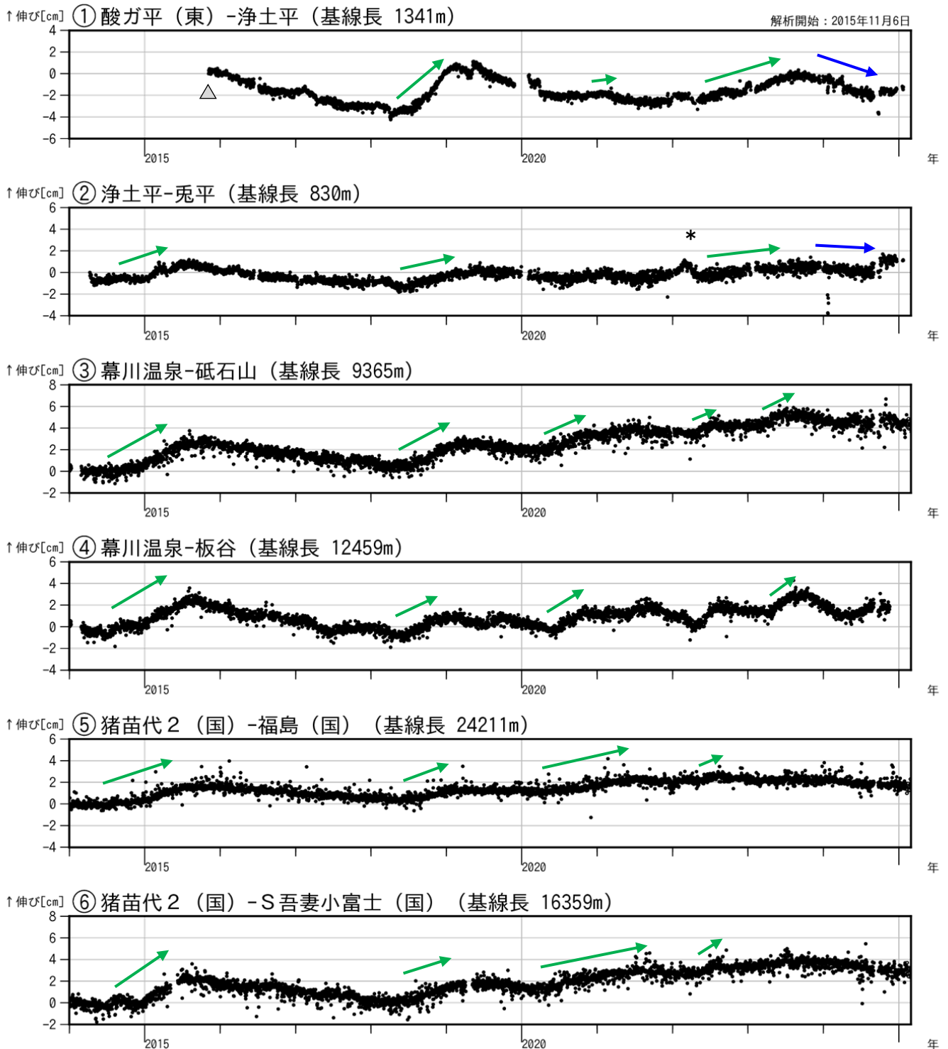
図4 吾妻山 吾妻山浅部・深部の地殻変動（2014年1月～2025年2月）
