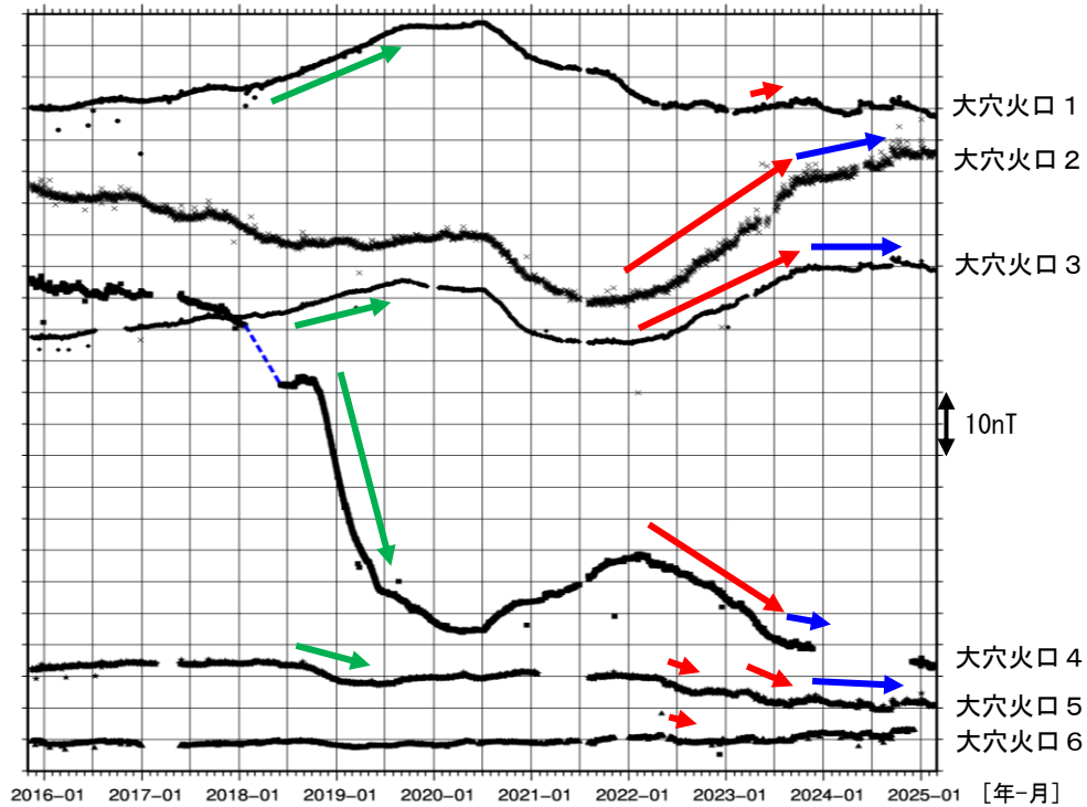
図 12 吾妻山 全磁力連続観測点の全磁力値変化（2015 年 11 月～2025 年 2 月）
