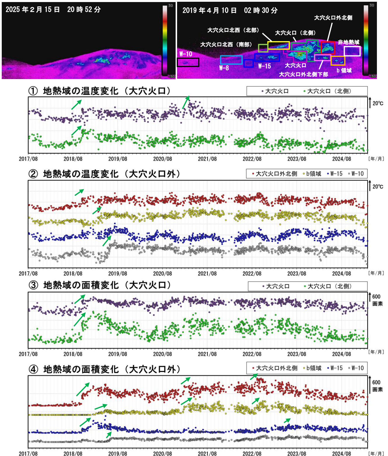
図5 吾妻山 監視カメラによる大穴火口周辺の地熱域の経過（2017年8月～2025年2月）
