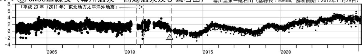
図2 吾妻山 中期的な火山活動の経過（2003年1月～2025年2月）
