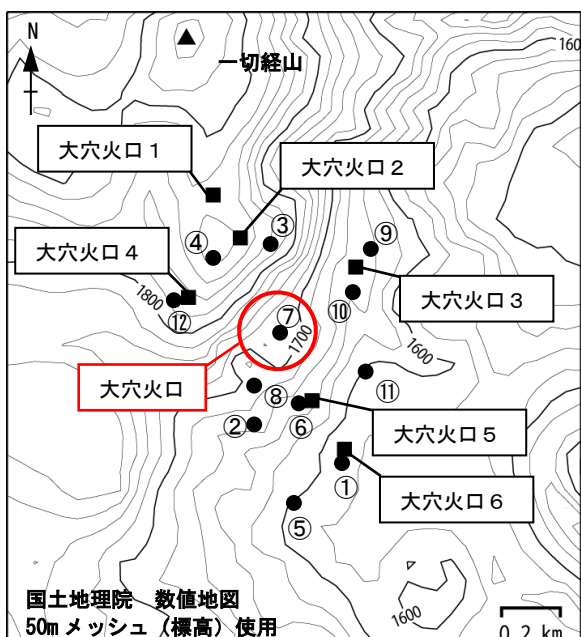
図 16 吾妻山 全磁力観測点配置図
