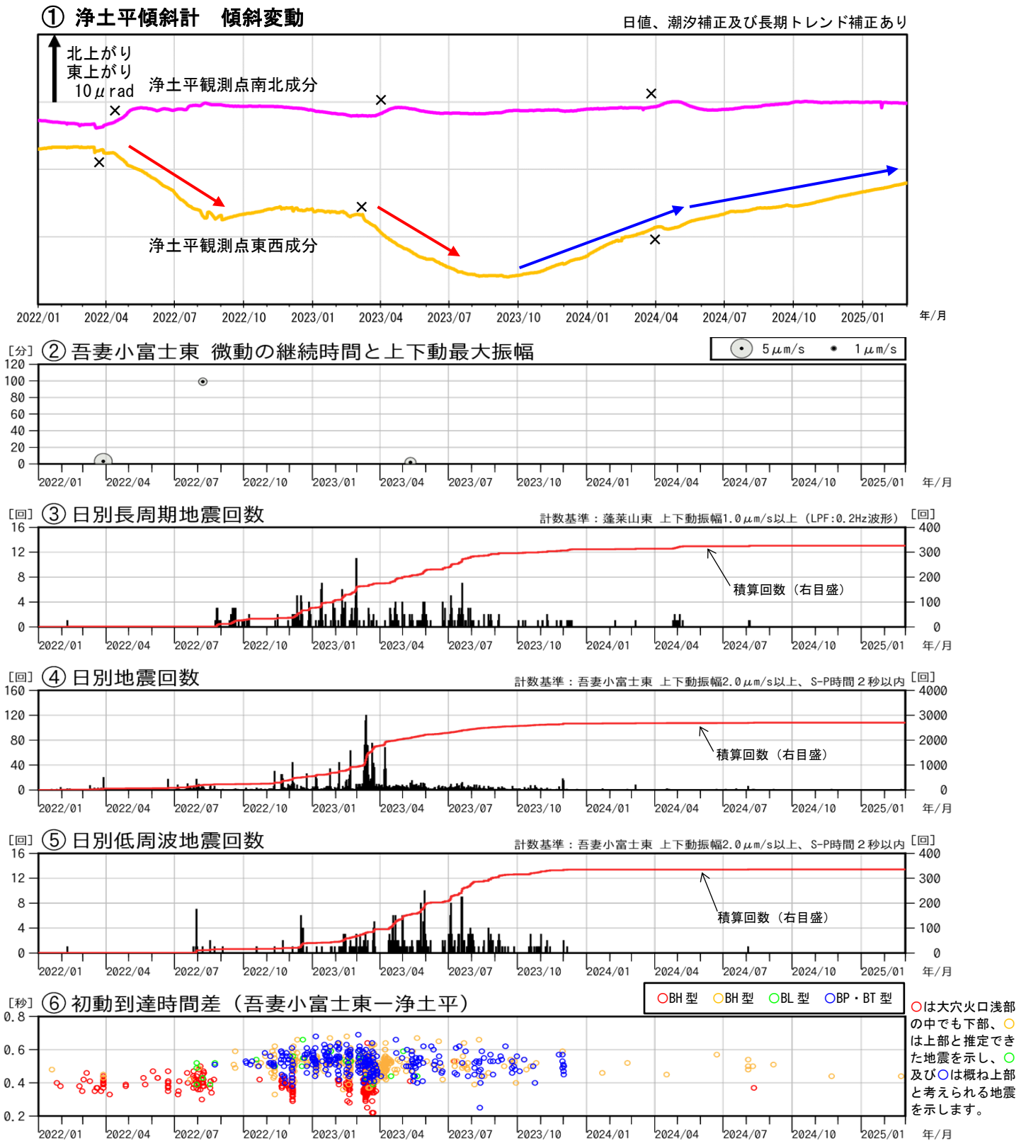
図3 吾妻山 火山活動経過図（2022年1月～2025年2月）
