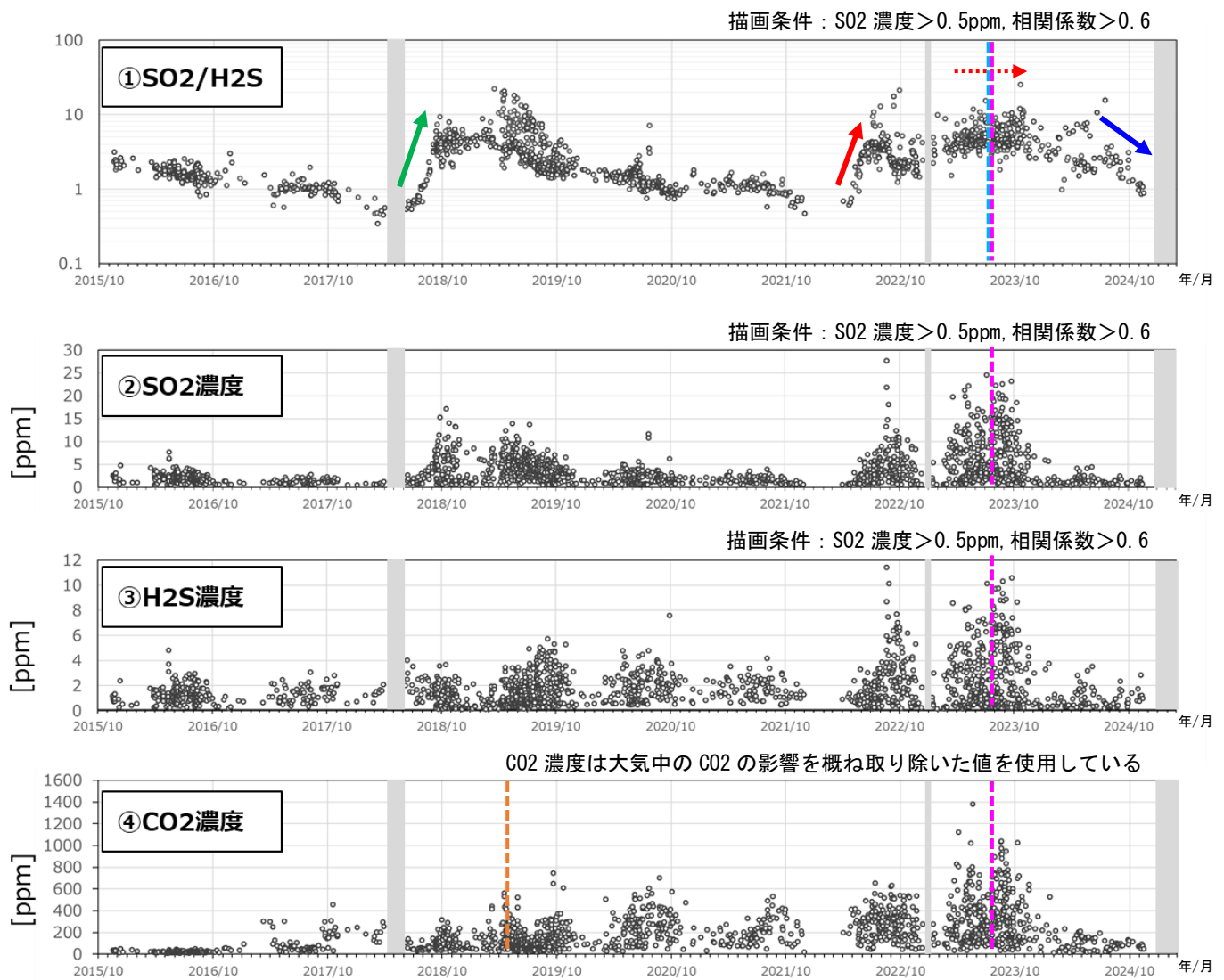
図 11 吾妻山 火山ガス観測装置による観測（2015 年 11 月～2025 年 2 月）
