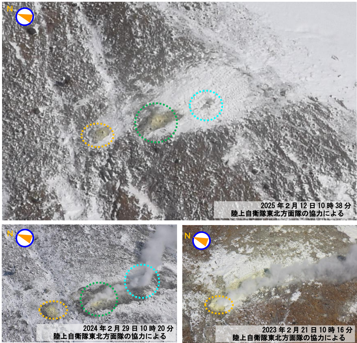
図10 上空から撮影した大穴火口北西の噴気の状況
