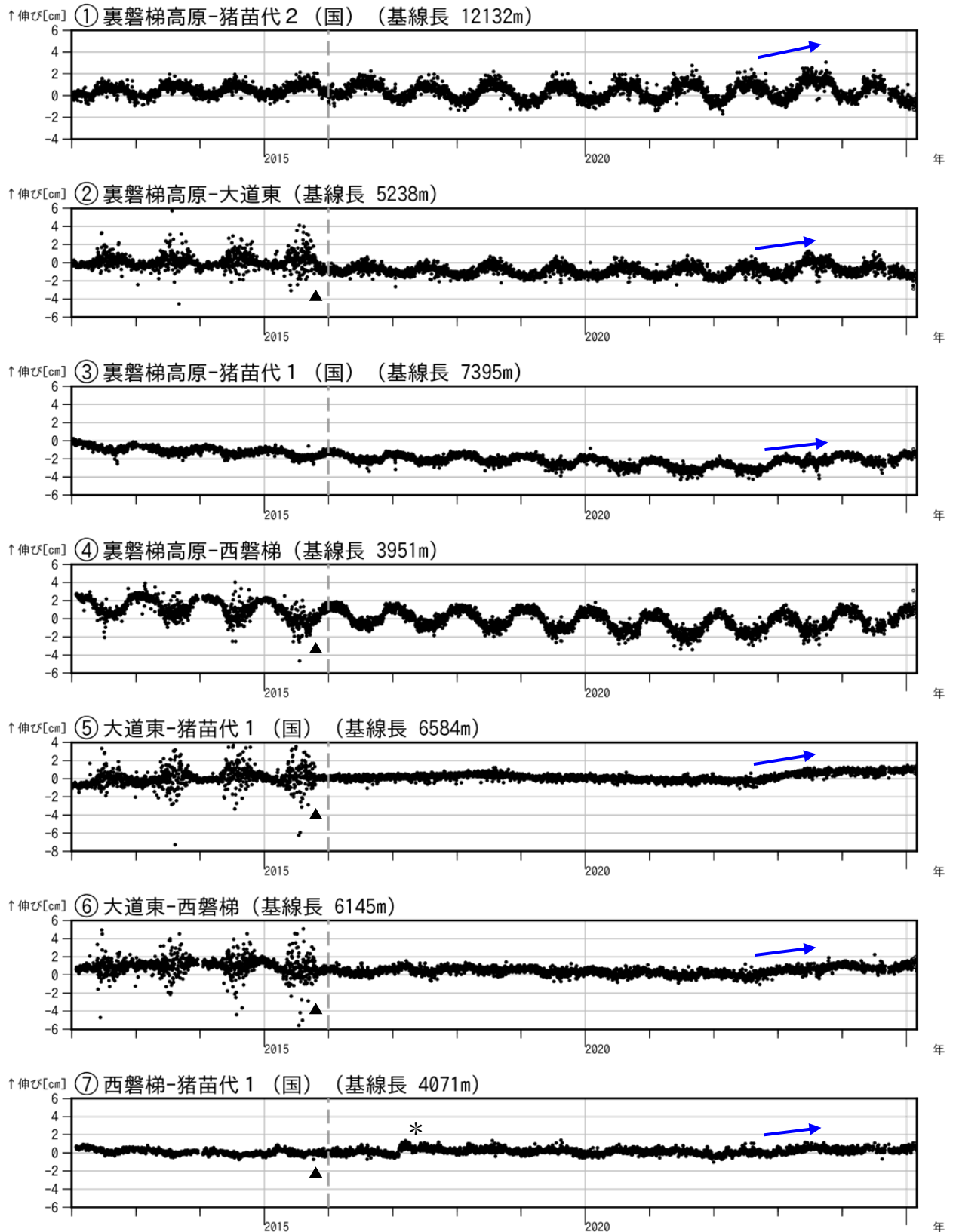
図10 磐梯山 GNSS 基線長変化図 (2012年1月～2025年2月)
