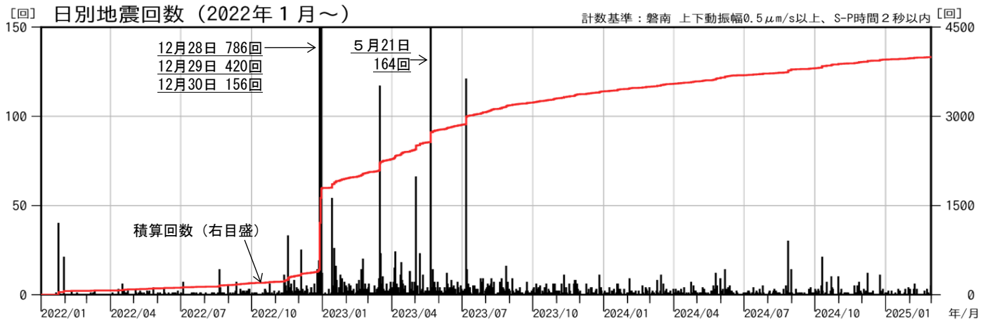
図 8 磐梯山 地震回数（2022 年 1 月～2025 年 2 月）
