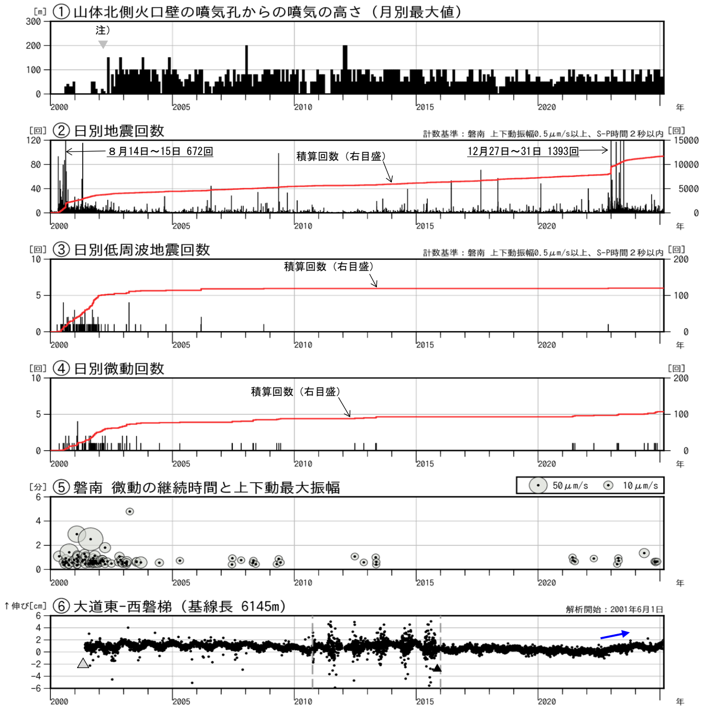
図7 磐梯山 火山活動経過図（2000年1月～2025年2月）
