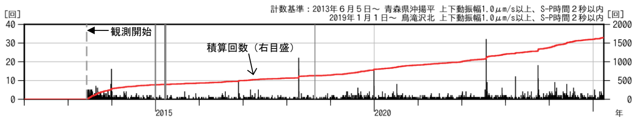
図2 八甲田山 日別地震回数（2013年6月～2025年3月）
