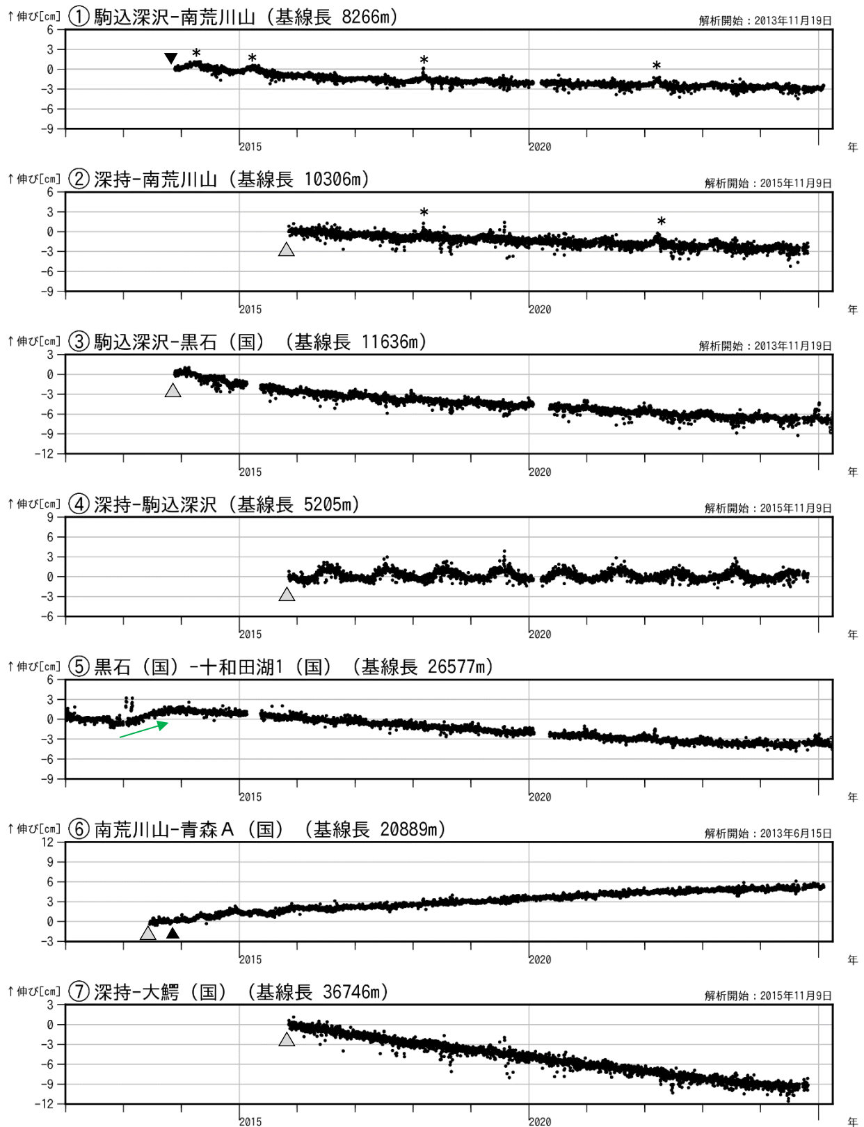
図3 八甲田山 GNSS 基線長変化図（2012年1月～2025年3月）
