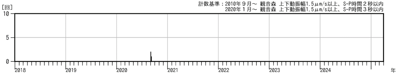
図 3 鳥海山 火山性地震の日別回数（2018 年 1 月～2025 年 3 月）
