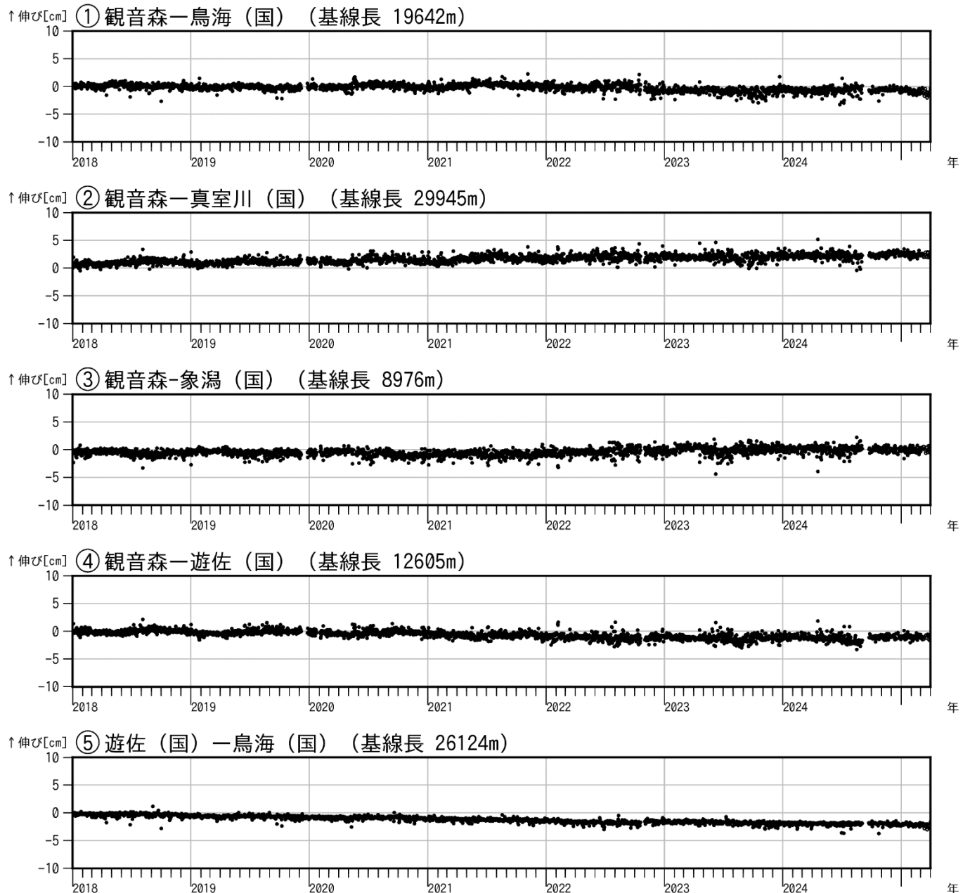
図 4 鳥海山 GNSS 基線長変化図（2018 年 1 月～2025 年 3 月）
