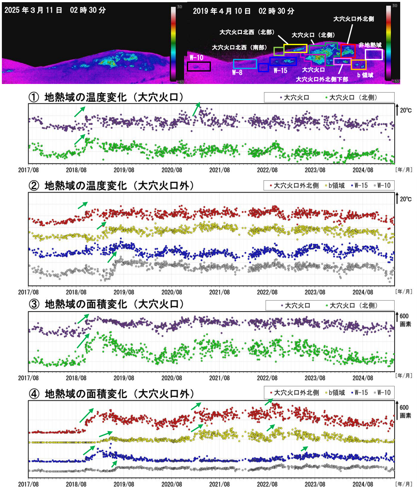
図5 吾妻山 監視カメラによる大穴火口周辺の地熱域の経過（2017 年 8 月～2025 年 3 月）
