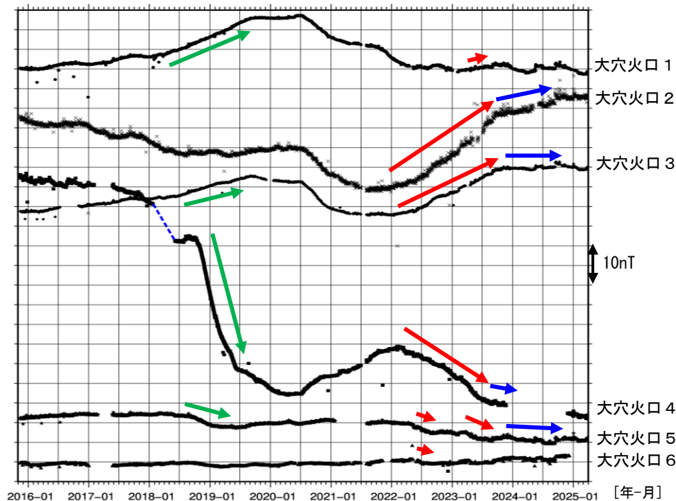
図 7 吾妻山 全磁力連続観測点の全磁力値変化（2015 年 11 月～2025 年 3 月）
