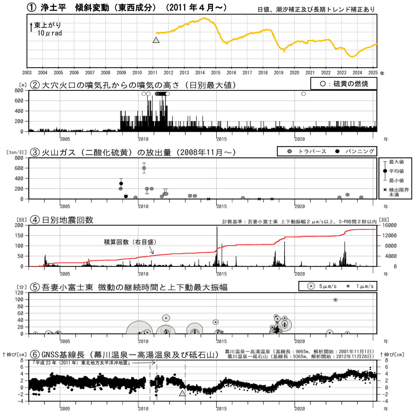
図2 吾妻山 中期的な火山活動の経過（2003年1月～2025年3月）
