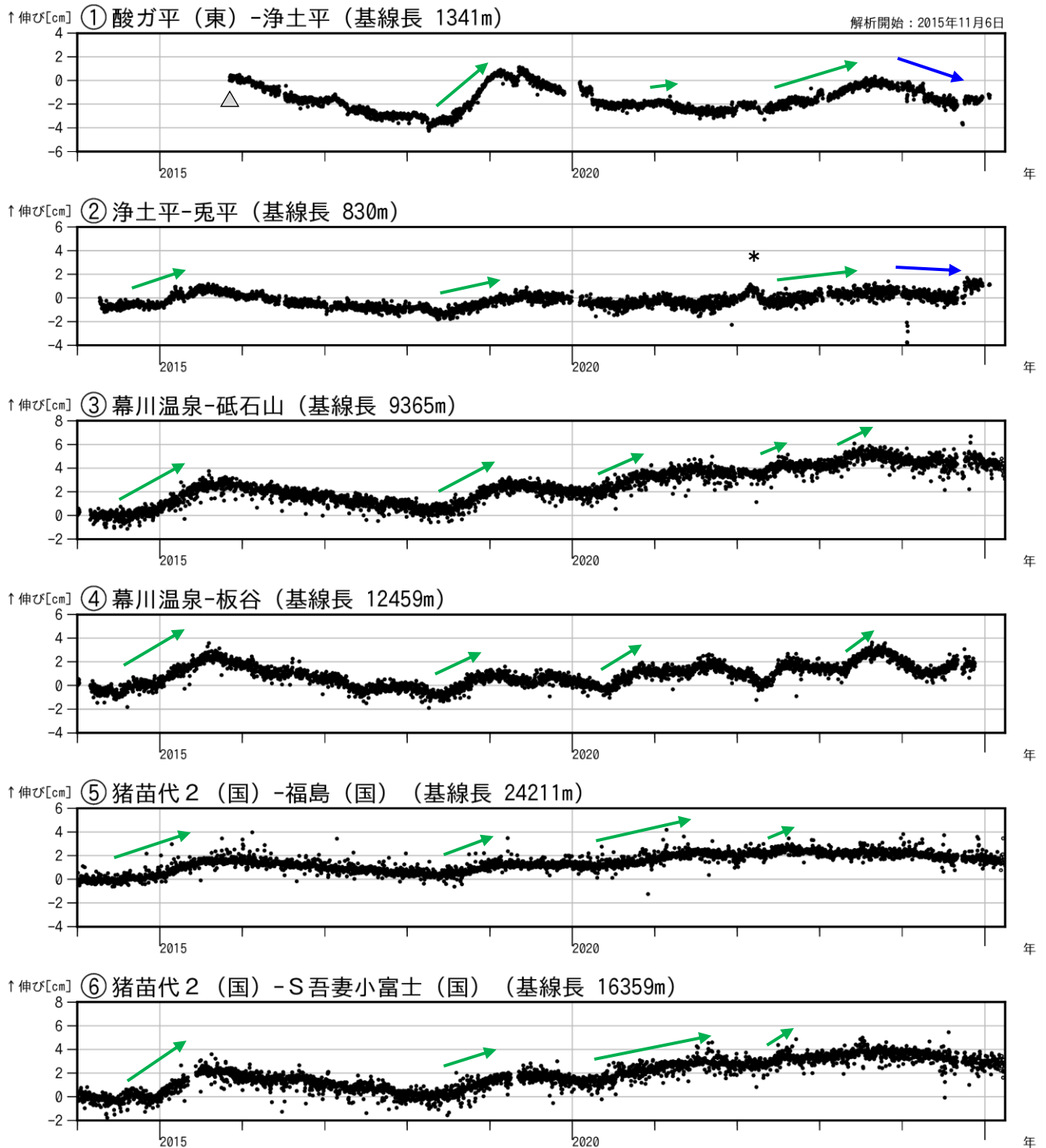
図4 吾妻山 吾妻山浅部・深部の地殻変動 (2014年1月～2025年3月)
