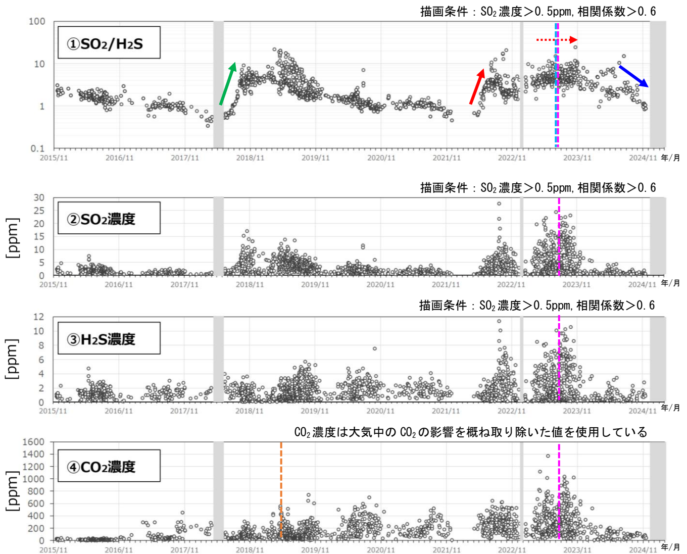
図6 吾妻山 火山ガス観測装置による観測（2015年11月～2025年3月）
