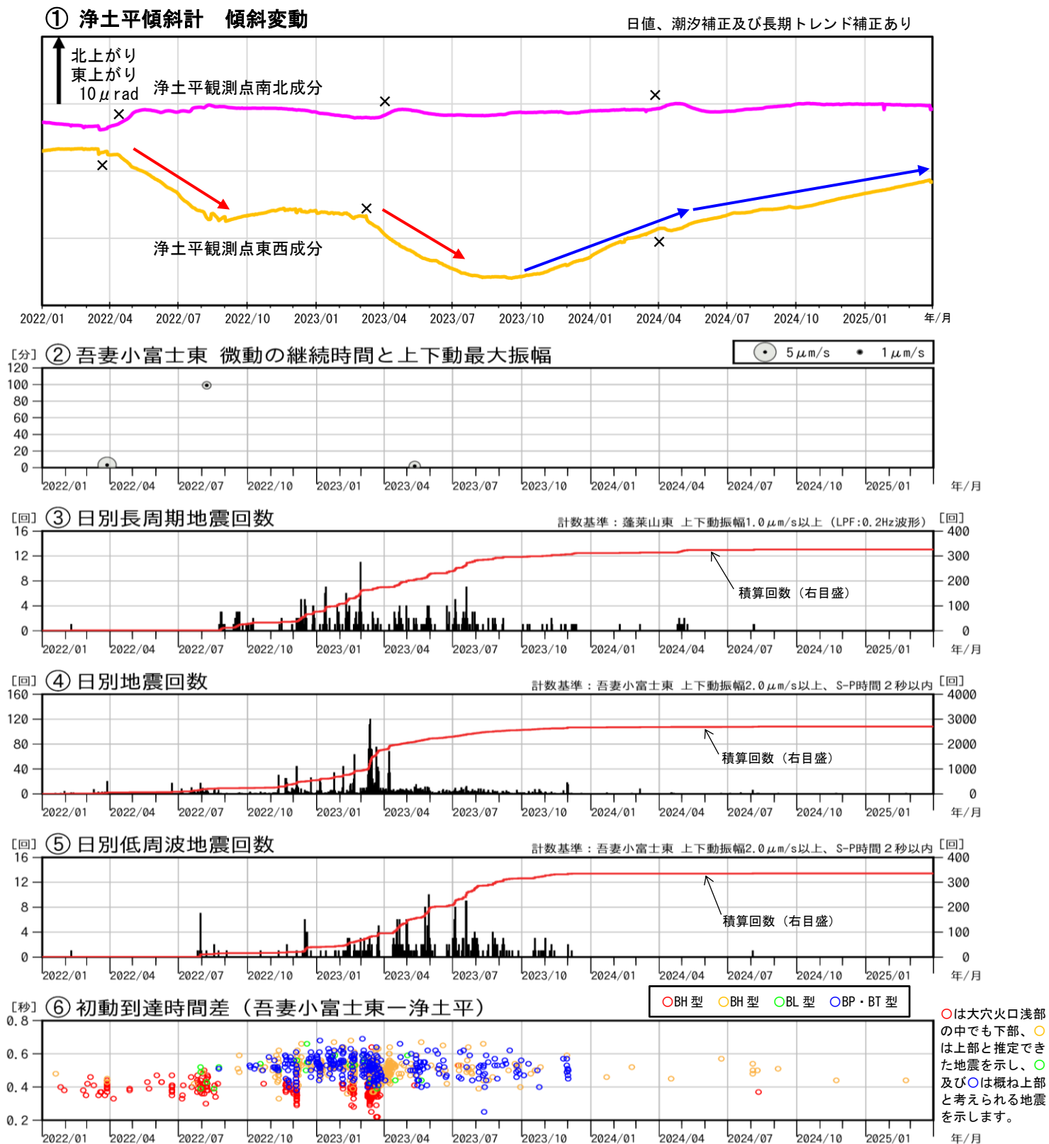
図3 吾妻山 火山活動経過図（2022年1月～2025年3月）
