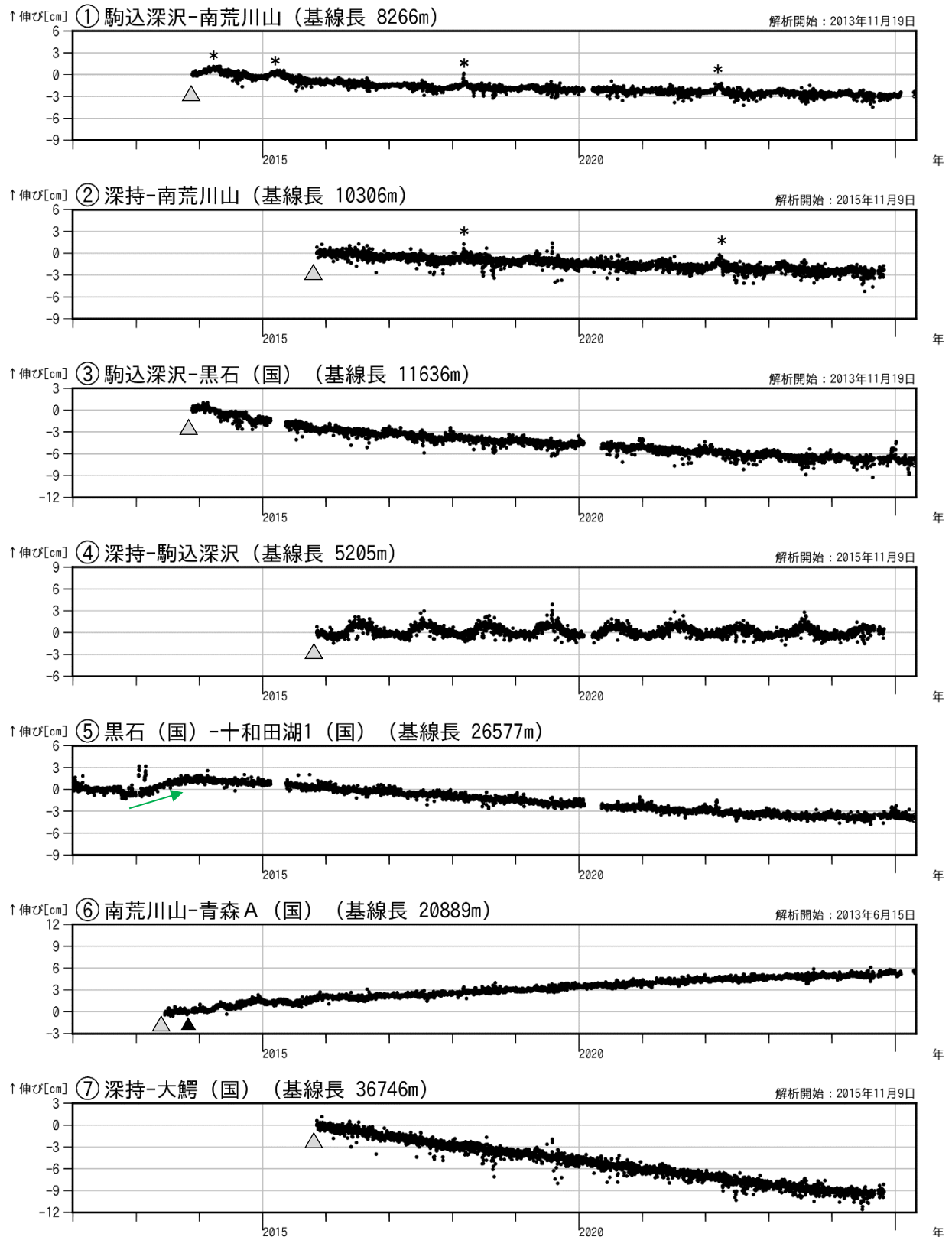
図3 八甲田山 GNSS 基線長変化図（2012年1月～2025年4月）
