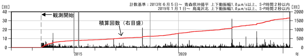
図2 八甲田山 日別地震回数（2013年6月～2025年4月）
