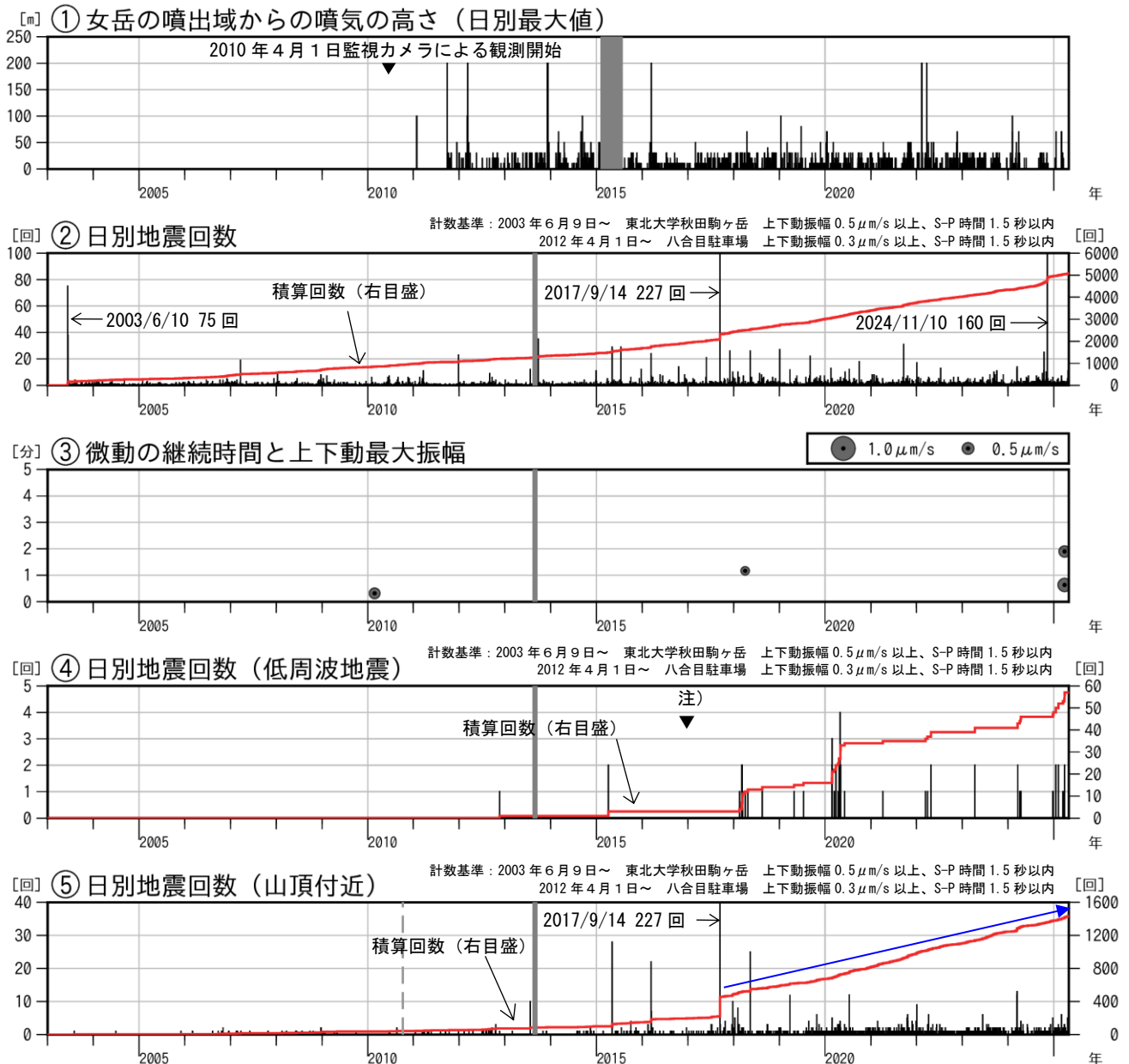
図2 秋田駒ヶ岳 火山活動経過図（2003年6月～2025年4月）
