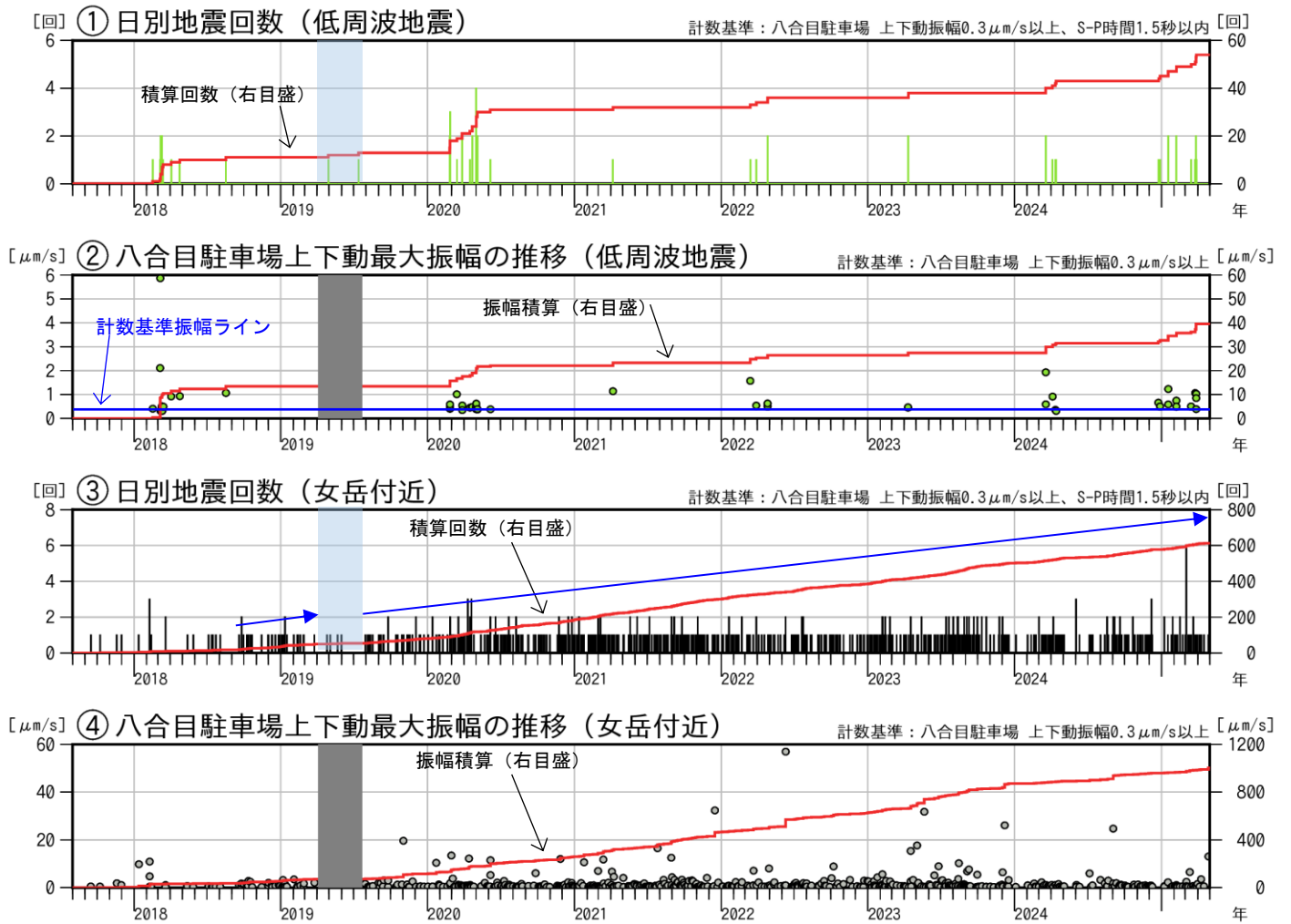
図3 秋田駒ヶ岳 低周波地震及び女岳付近の日別回数と最大振幅（2017年8月～2025年4月）
