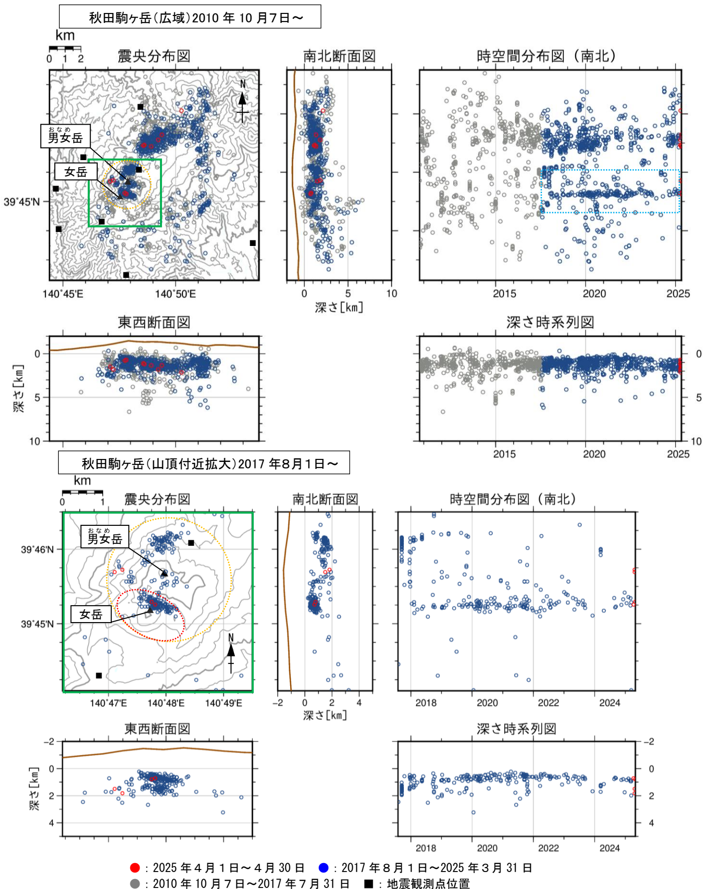
図4 秋田駒ヶ岳 地震活動（2010年10月7日～2025年4月）
