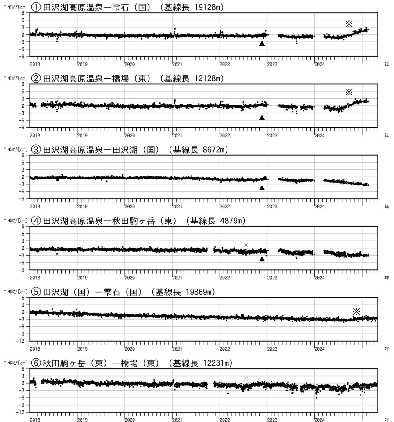
図5 秋田駒ヶ岳 GNSS 基線長変化図（2018年1月～2025年4月）
