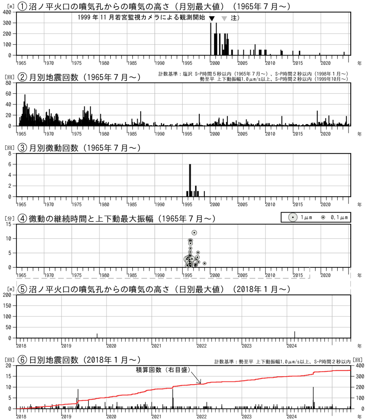
図3 安達太良山 火山活動経過図（1965年7月～2025年5月）
