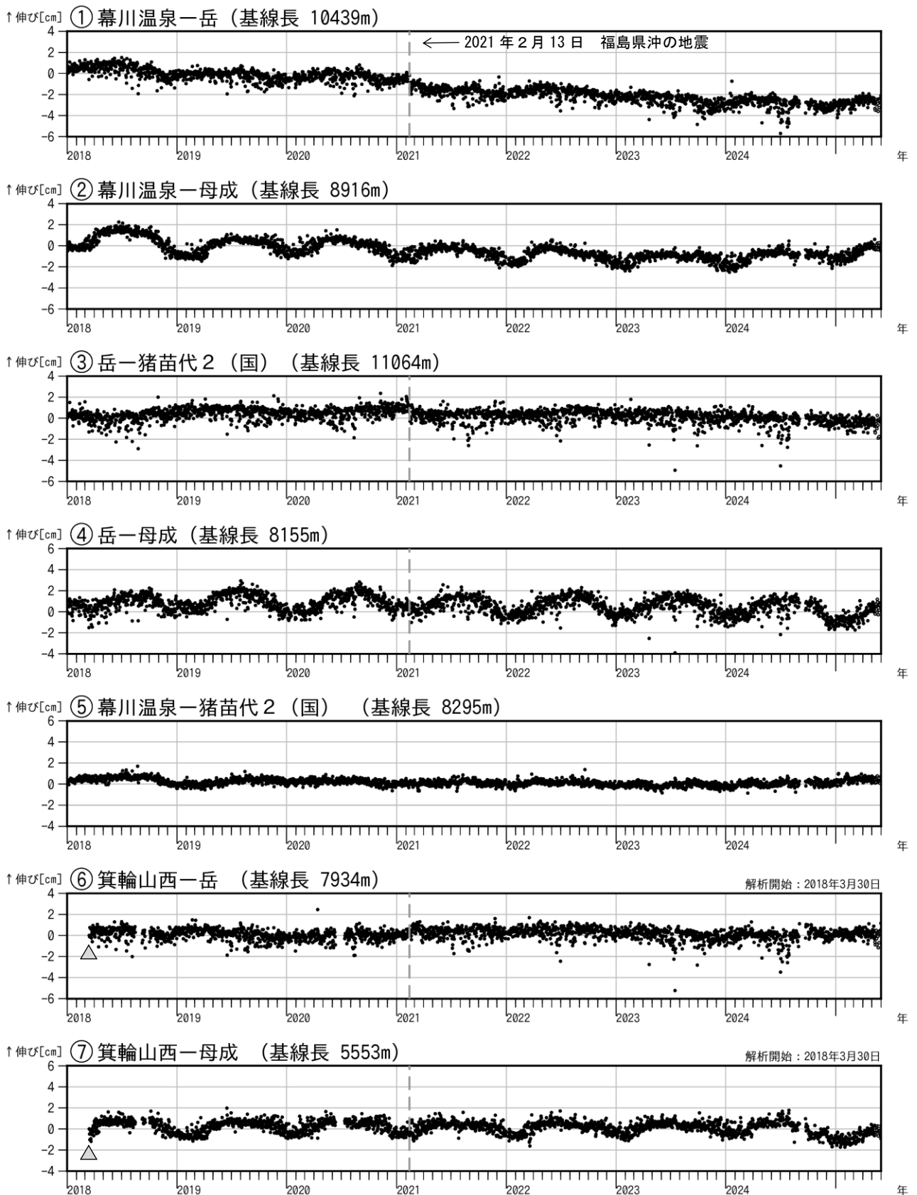
図4 安達太良山 GNSS 基線長変化図（2018年1月～2025年5月）
