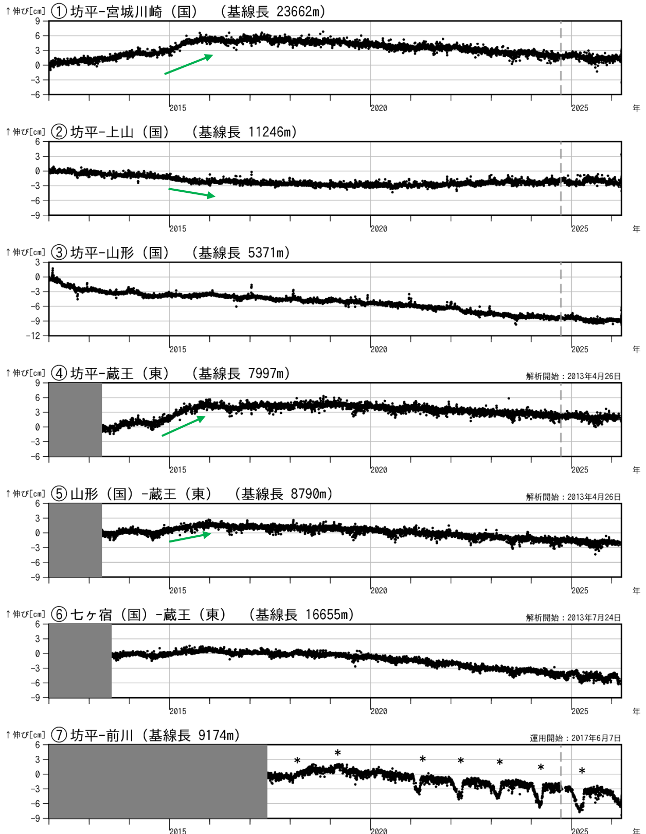
図3 蔵王山 GNSS 基線長変化図（2012年1月～2026年3月）
